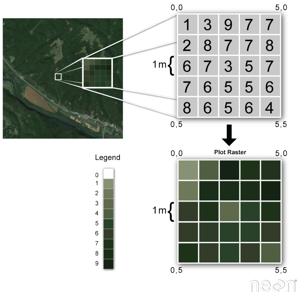
Figuur 11.1.8: Raster data uitgelegd (Bron: National Ecological Observatory Network, NEON).
