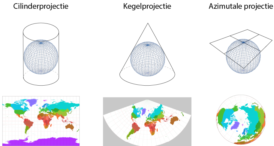
Figuur 4.1.4: Cilinderprojectie, kegelprojectie en azimuthale projectie en de kaarten die ze opleveren (bronnen: gemaakt door Julia Fossa Marques; Wikimedia Commons).
