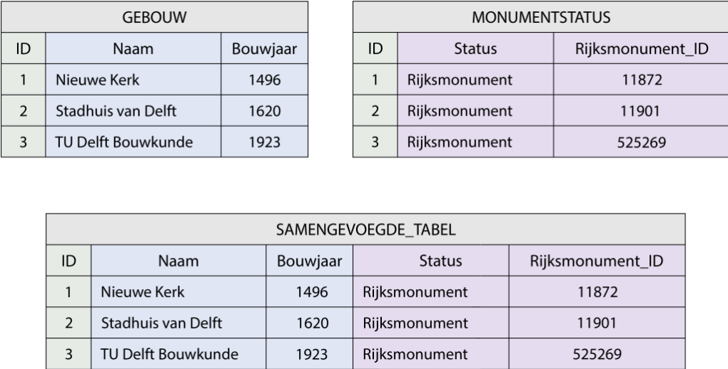
Figuur 11.1.2: Tabellen koppelen op basis van een ID-kolom (Gemaakt door Julia Fossa Marques).
