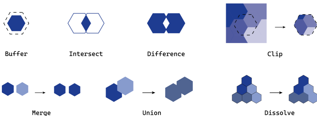
Figuur 11.1.7: Overzicht van geoprocessing tools (gemaakt door Julia Fossa Marques).
