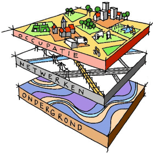
Afbeelding 10.2.1: de lagenbenadering.
