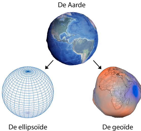
Figuur 4.1.1: De vorm van de aarde (bron: NASA, bewerkt door Julia Fossa Marques).
