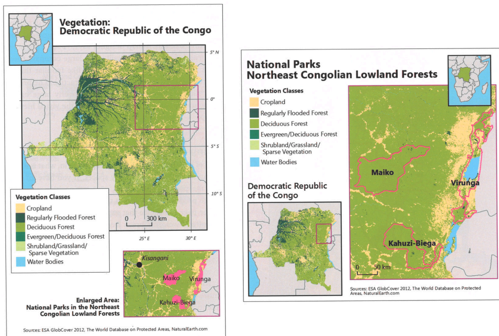
Figuur 4.1.7: Voorbeeld voor het gebruik van kleuren volgens de basisregels (bron: Brewer 2016, copyright Brewer).
