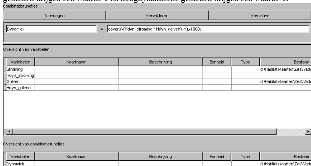
Figuur 24 Screenshot HABITAT. Model "Dynamiek". De functie cover() heeft als resultaat dat alle missing values worden vervangen door de waarde -1000 (PCRaster, 1996).
