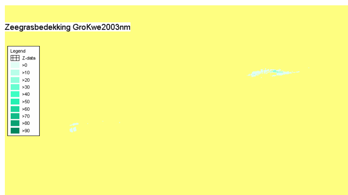
Figuur 7 Grokwe1.bil. Bedekking (%) zeegras op de Groninger Kwelders in 2003.
