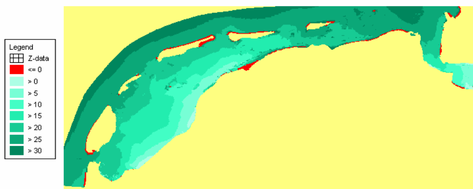
Figuur 3 B88.bil. Zoutconcentratie in een natte periode van een nat jaar. Alle gele cellen zijn missing values.
