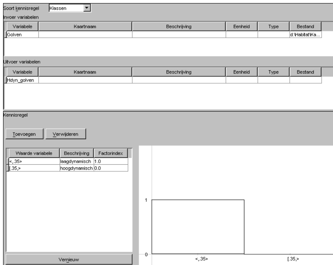
Figuur 23 Screenshot HABITAT. Kennisregel "Golgen" binnen het model "Dynamiek". Gebieden met lage golfdynamiek krijgen de waarde 1 voor Hdyn_golgen en gebieden met hoge golfdynamiek krijgen de waarde 0.
