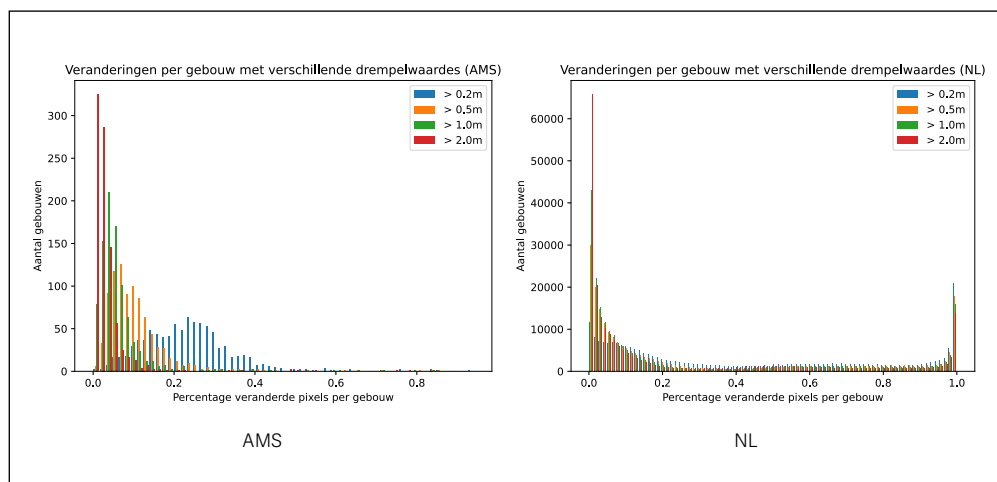
Figuur 7. Hoogteverschillen tussen AHN3 en AHN4 per ongewijzigd BAG-pand.
