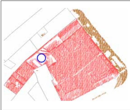
Figuur 10. Voorbeeld no data -cirkel (de grootste cirkel binnen een BAG-polygoon die geen AHN-punten bevat).
