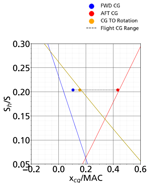
Fig. 6 D239 (Point design) scissors
