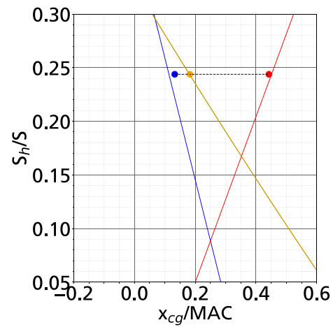
Fig. 9 D239-S (Family design) scissors
