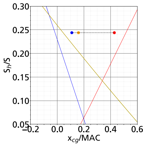
Fig. 8 D239 (Family design) scissors
