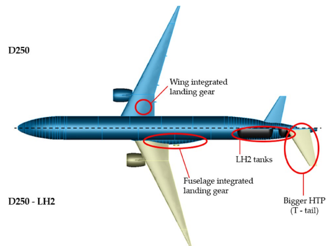
Fig. 20 D250-LH2 (bottom) and D250 (top) concepts
