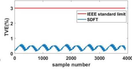
Fig 5. TVE (Test 3.1)
