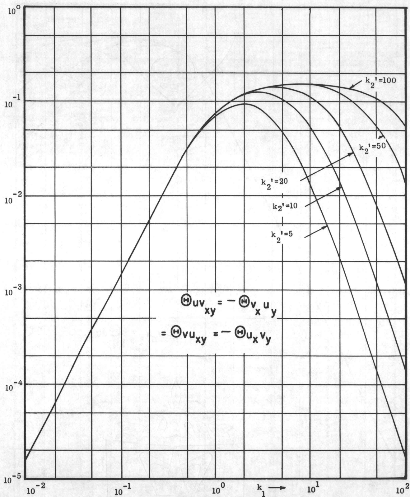
FIG. 18 SPECTRUM FUNCTION \Phi_{uv} L / \sigma^2 xy
