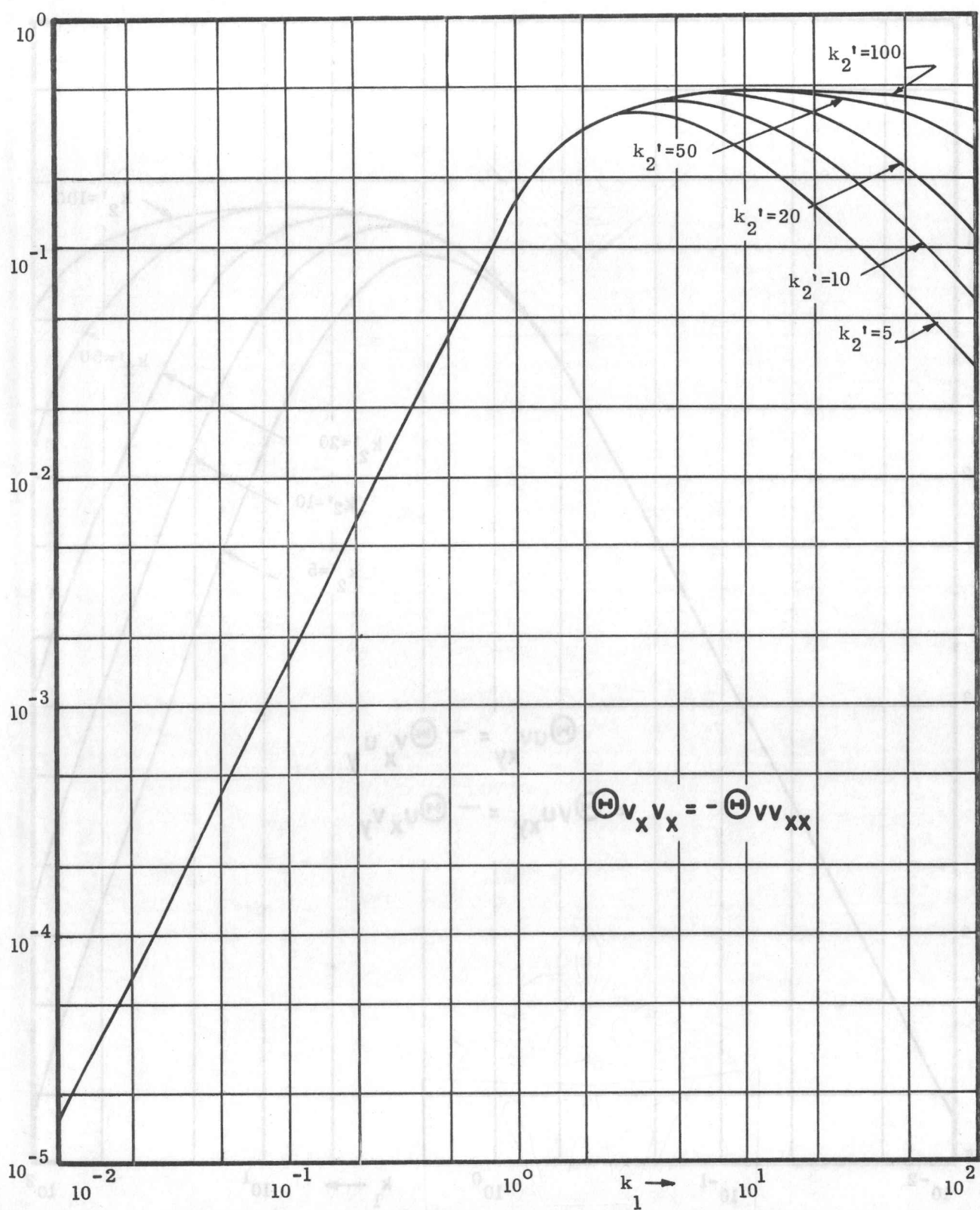
FIG. 19 SPECTRUM FUNCTION \Phi_{v_x v_x} L / \sigma^2
