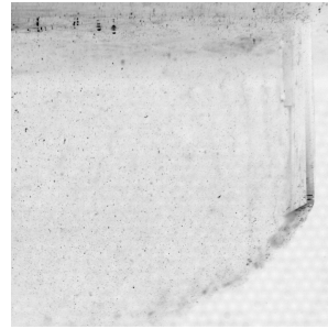
(f) h = 0 mm, t = 4.00 s. Steady phase.
