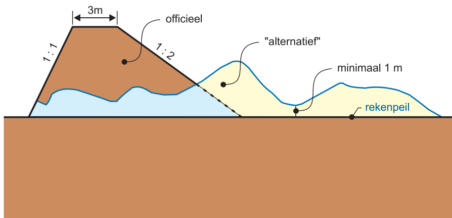
Figuur 8. Grensprofiel met alternatief grensprofiel
