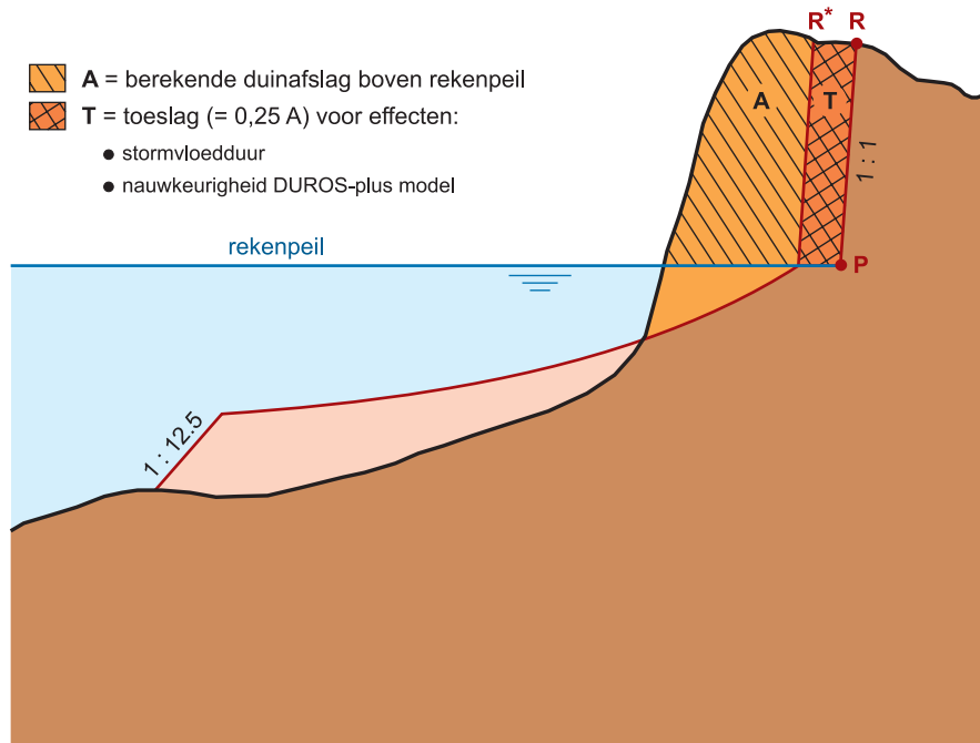
Figuur 5. DUROS-plus model met Toeslag
