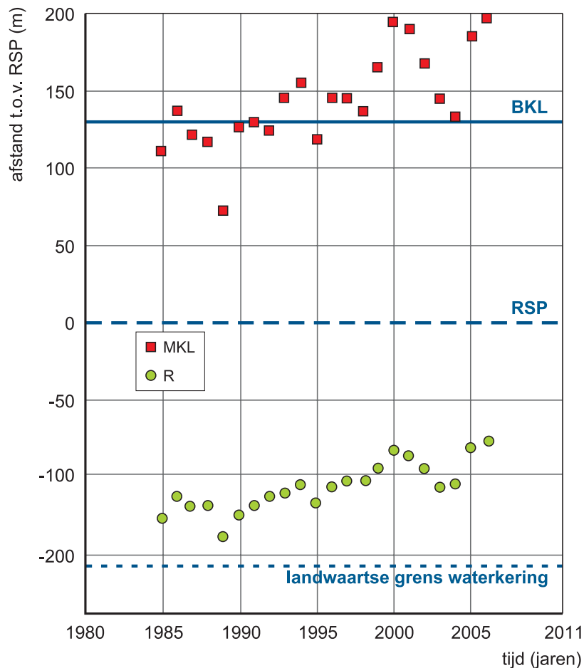
Figuur 6. R-t figuur met BKL , MKL , R en landwaartse grens waterkering
