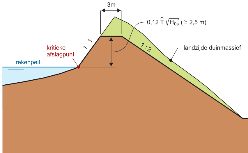
Figuur 7. Gensprofiel met inpassing achterkant duin
