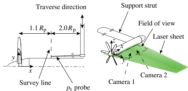
b) Pitot probe
