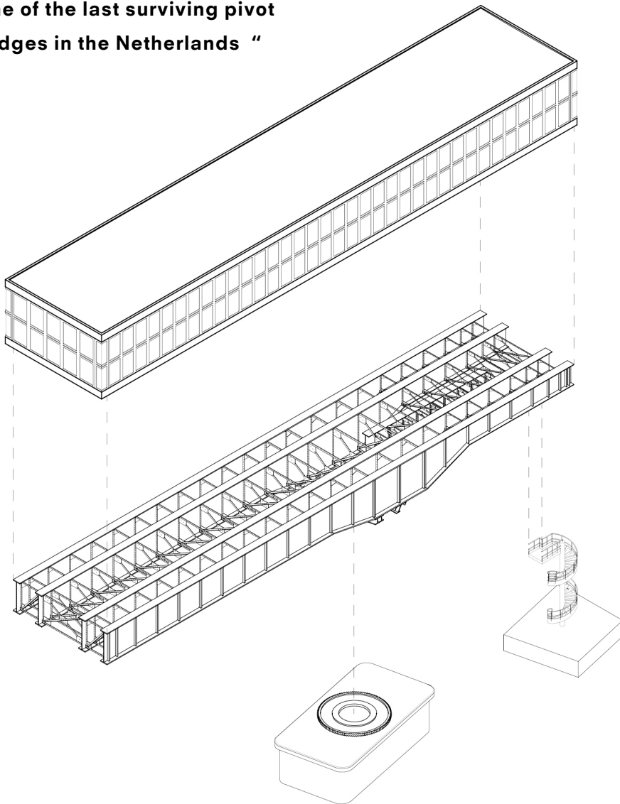
Axonometry
