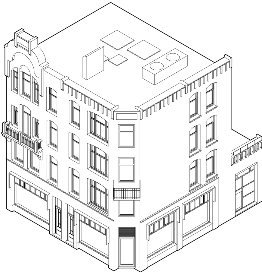
Axonometry
