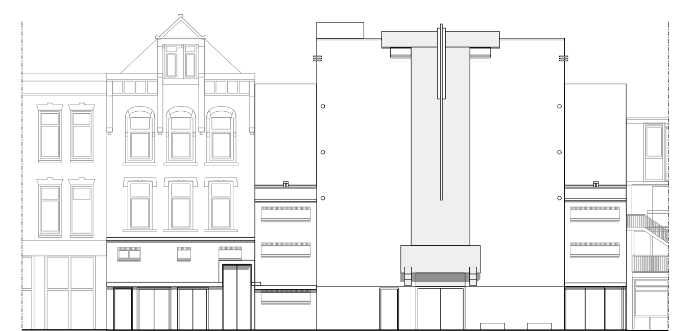
ELEVATION GOURVERNESTRAAT 1:200
