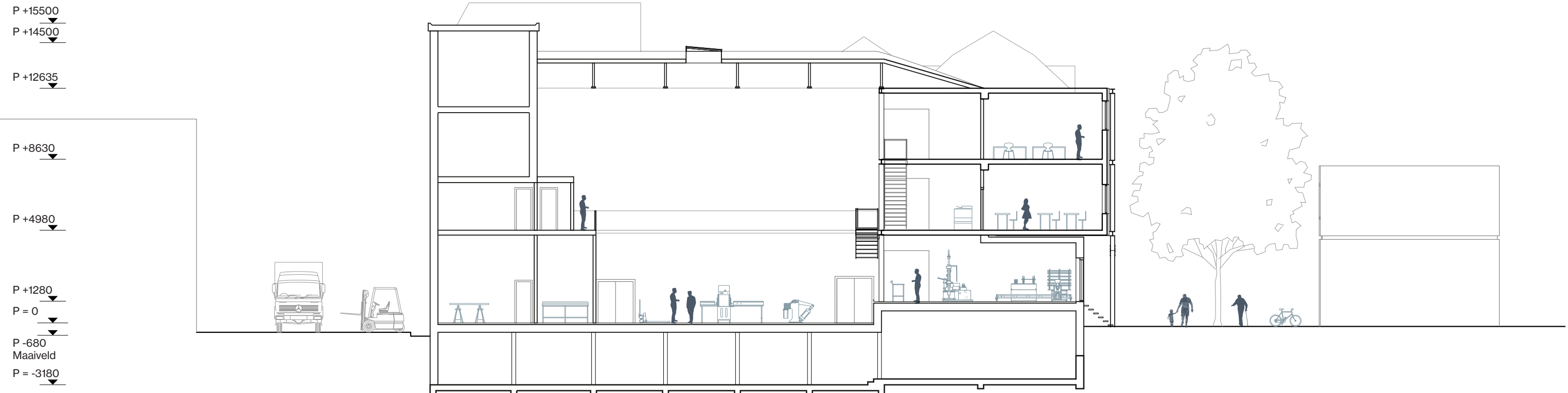
SECTION BB' 1:200
