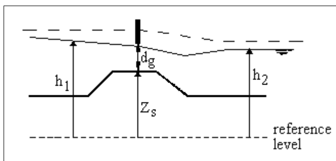
Figuur 16 Principe van een onderlaat
