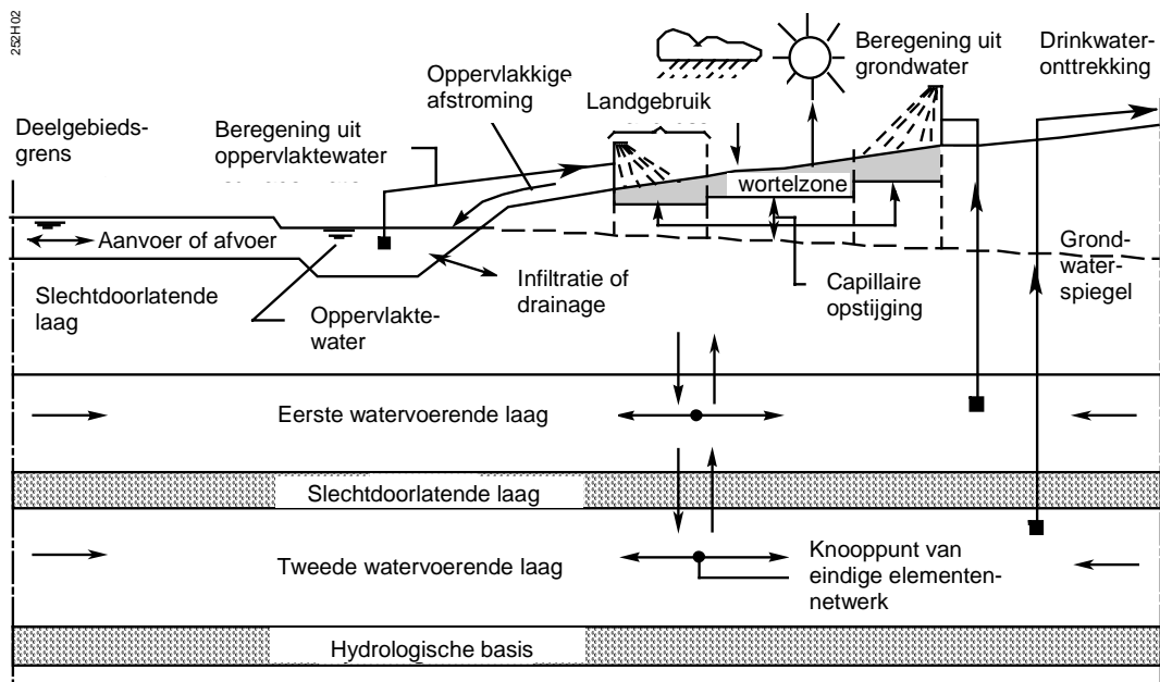
Figuur 5 Schema van processen in het regionaal hydrologisch model SIMGRO
