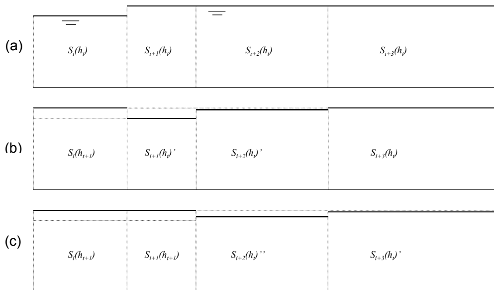
Figuur 13 Rekenwijze (in SIMGRO) voor stroming in de ‘omgekeerde’ richting. De aanname is dat het water in aanvoersituaties frictieloos kan worden verplaatst. Bij de nieuwe berekening van het peil in traject i , gaat de uitgangssituatie (a) over in (b), waarbij ervoor gezorgd wordt dat er een sluitende waterbalans is, en dat het peil in i niet hoger stijgt dan in traject i+1 en traject i+2 . In stap (c) wordt het peil in traject i+1 op het niveau van i+3 gebracht, enz. Het netto effect is het ‘schuiven’ met water
