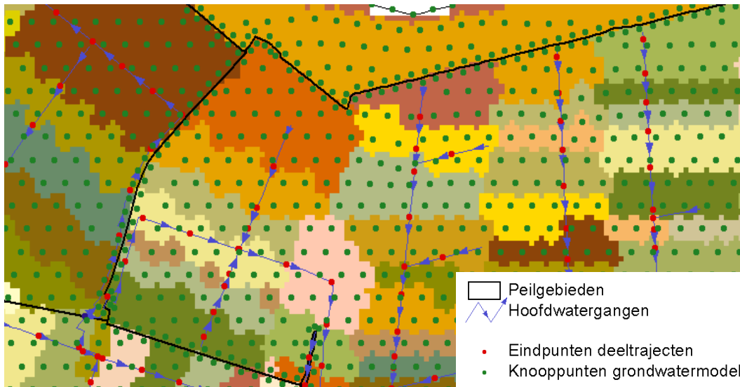
Figuur 18 Indeling in afwateringseenheden op basis van het kortste afstand criterium naar het eindpunten van de oppervlaktewaterdeeltrajecten (rode stippen). De plaatsing van de knooppunten is dusdanig dat de grenzen van peilgebieden ook in de modelschematisering worden aangehouden
