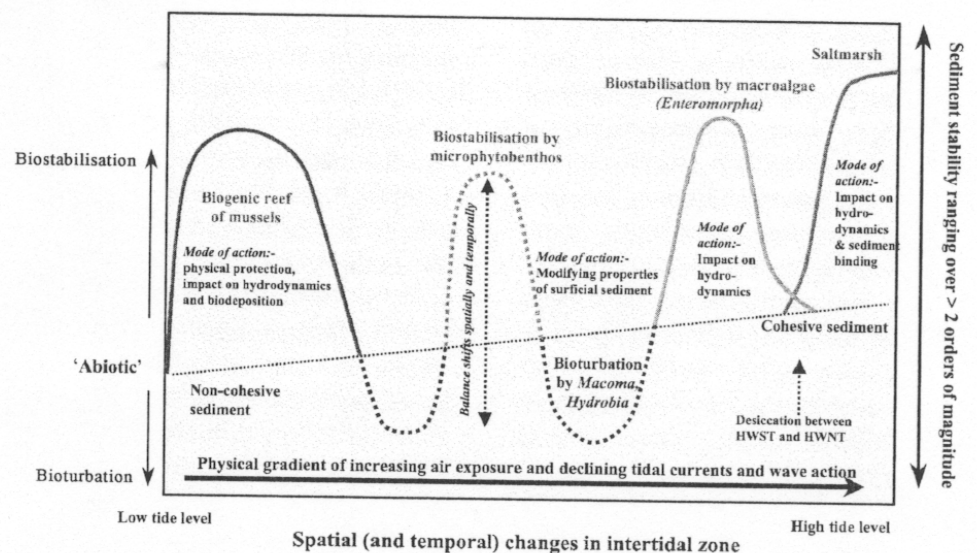
Figuur 23 Schematische weergave van aantal biologische en fysische processen die invloed hebben op de sediment stabiliteit in een getijdengebied. Widdows, 2002.
