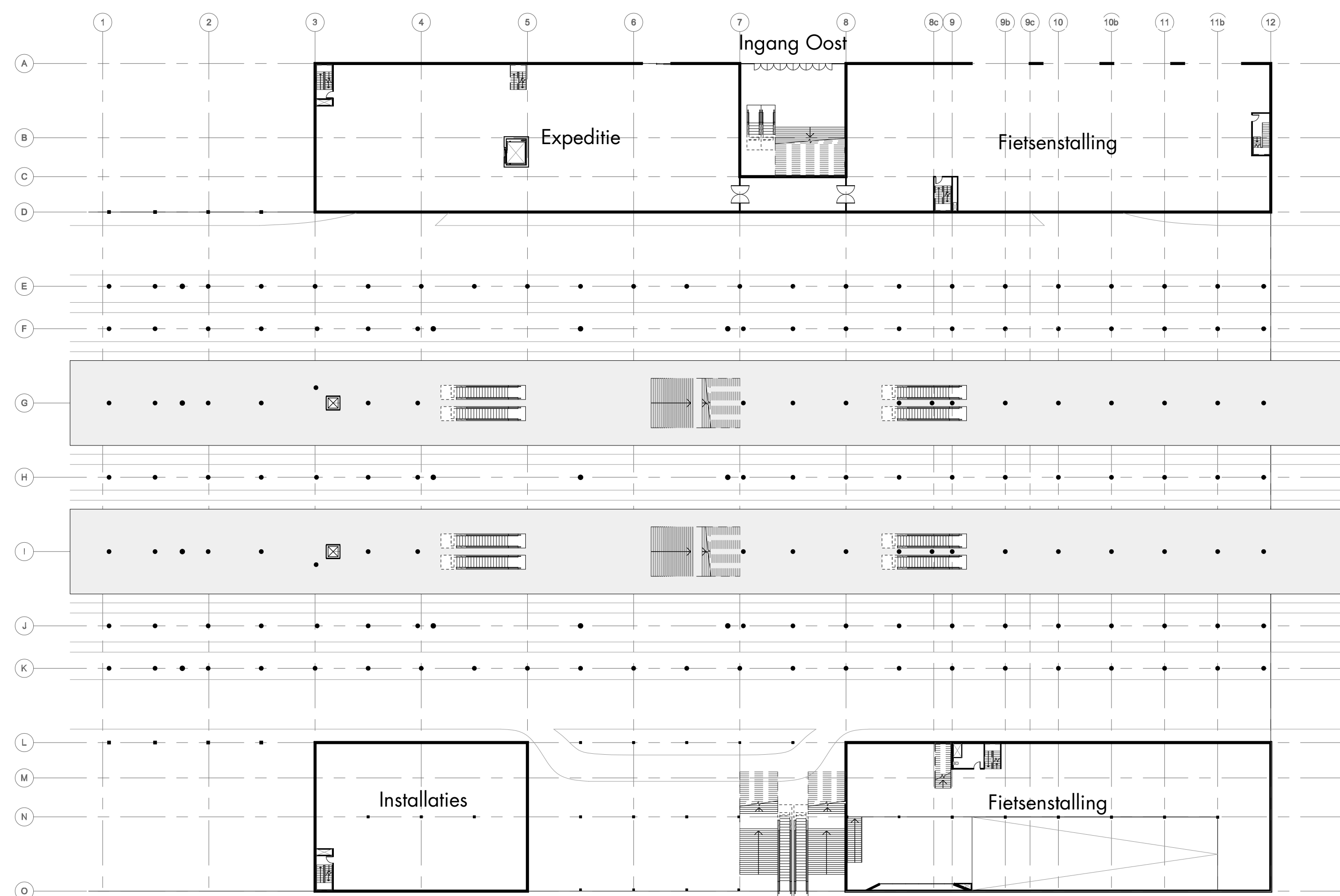
Niveau 0: Entree Moskeezijde & Perrons
