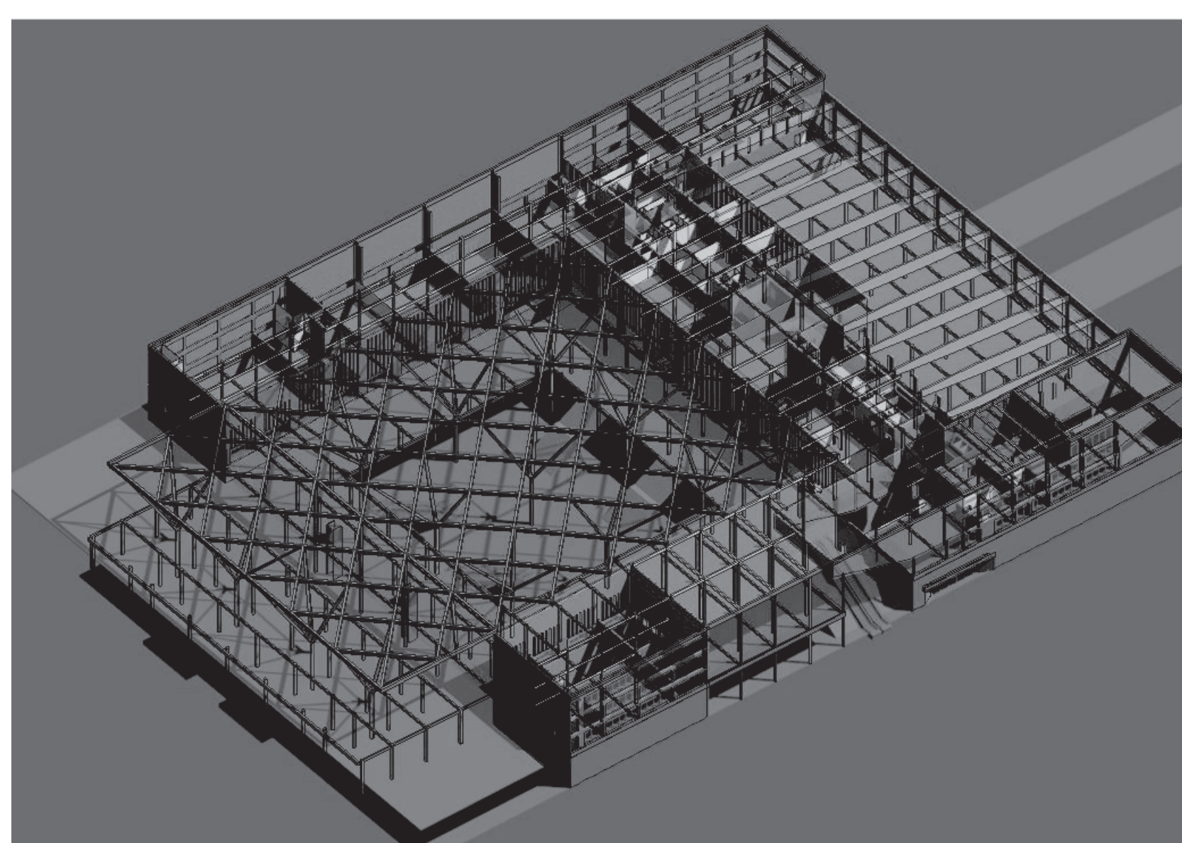
Ruimtelijke werking constructie
