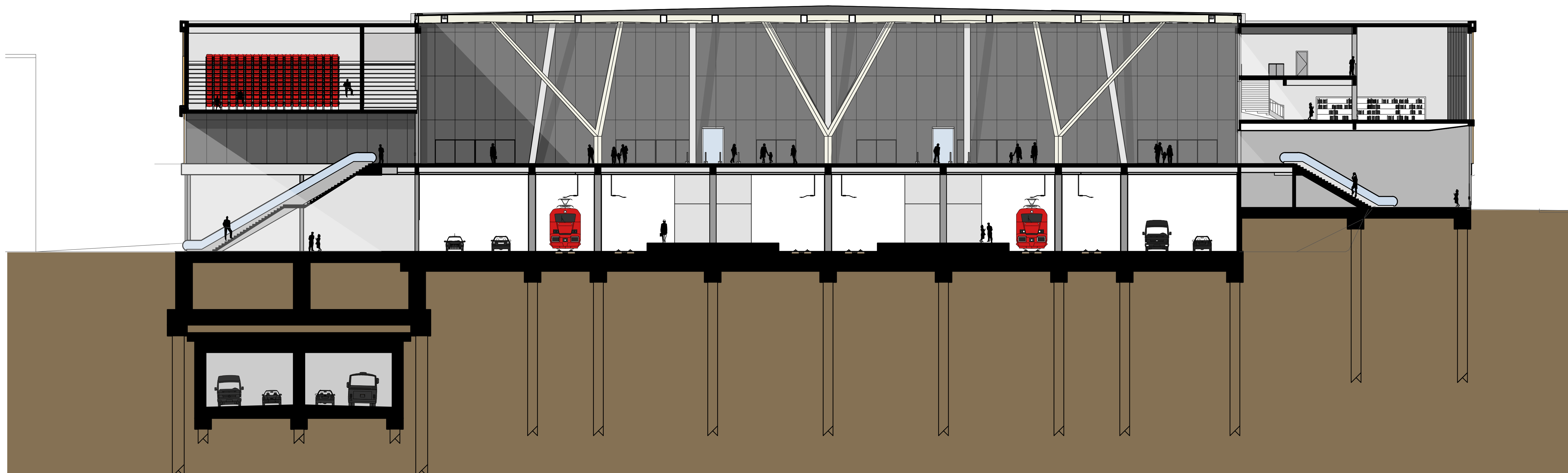
Dwarsdoorsnede
