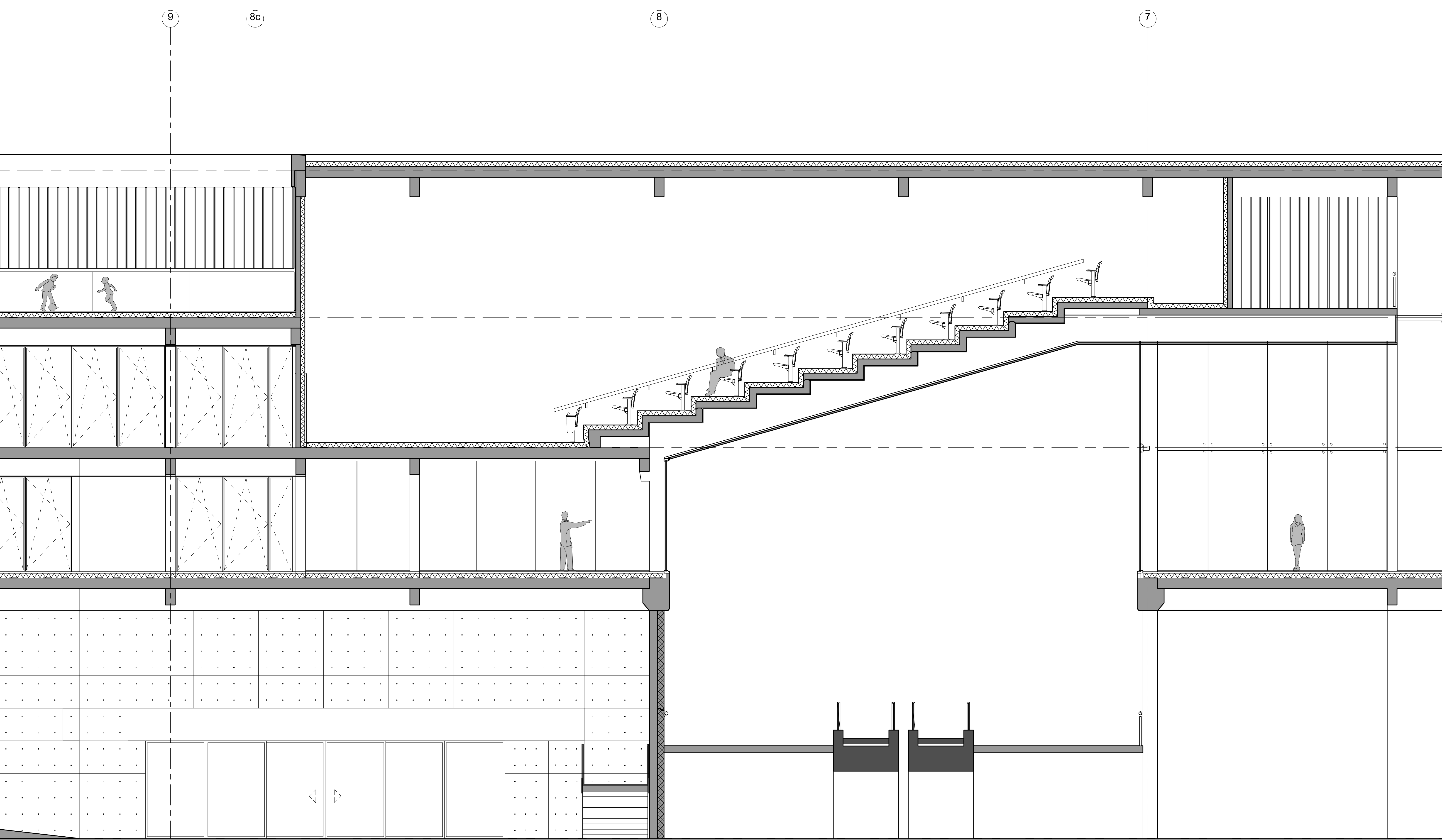
Langsdoorsnede Ingang Moskeezijde
