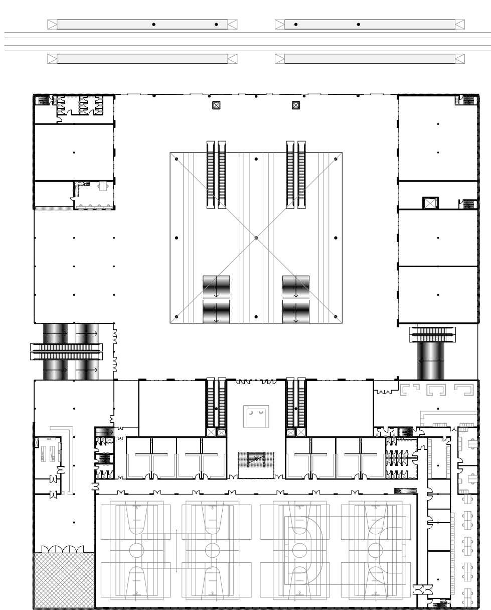
Constructieve opzet stationshal
