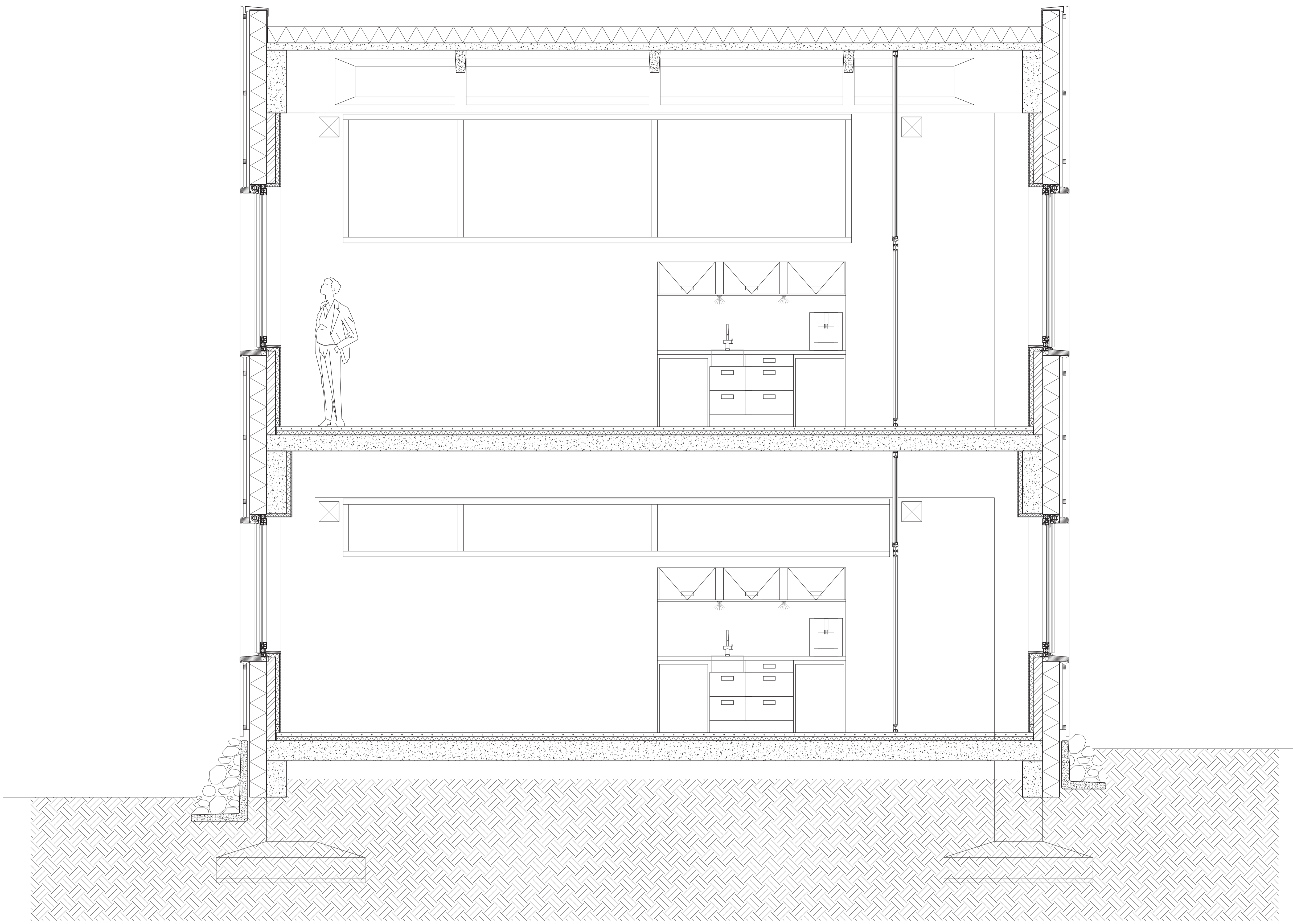
doorsnede startersruimte 1:25
