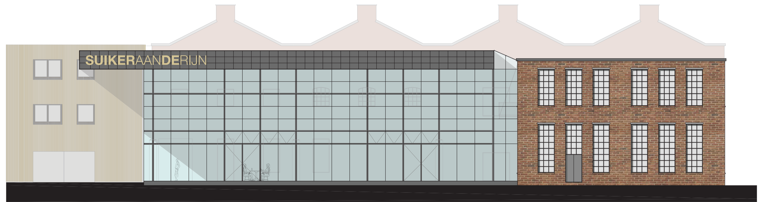
oostgevel 1:150
