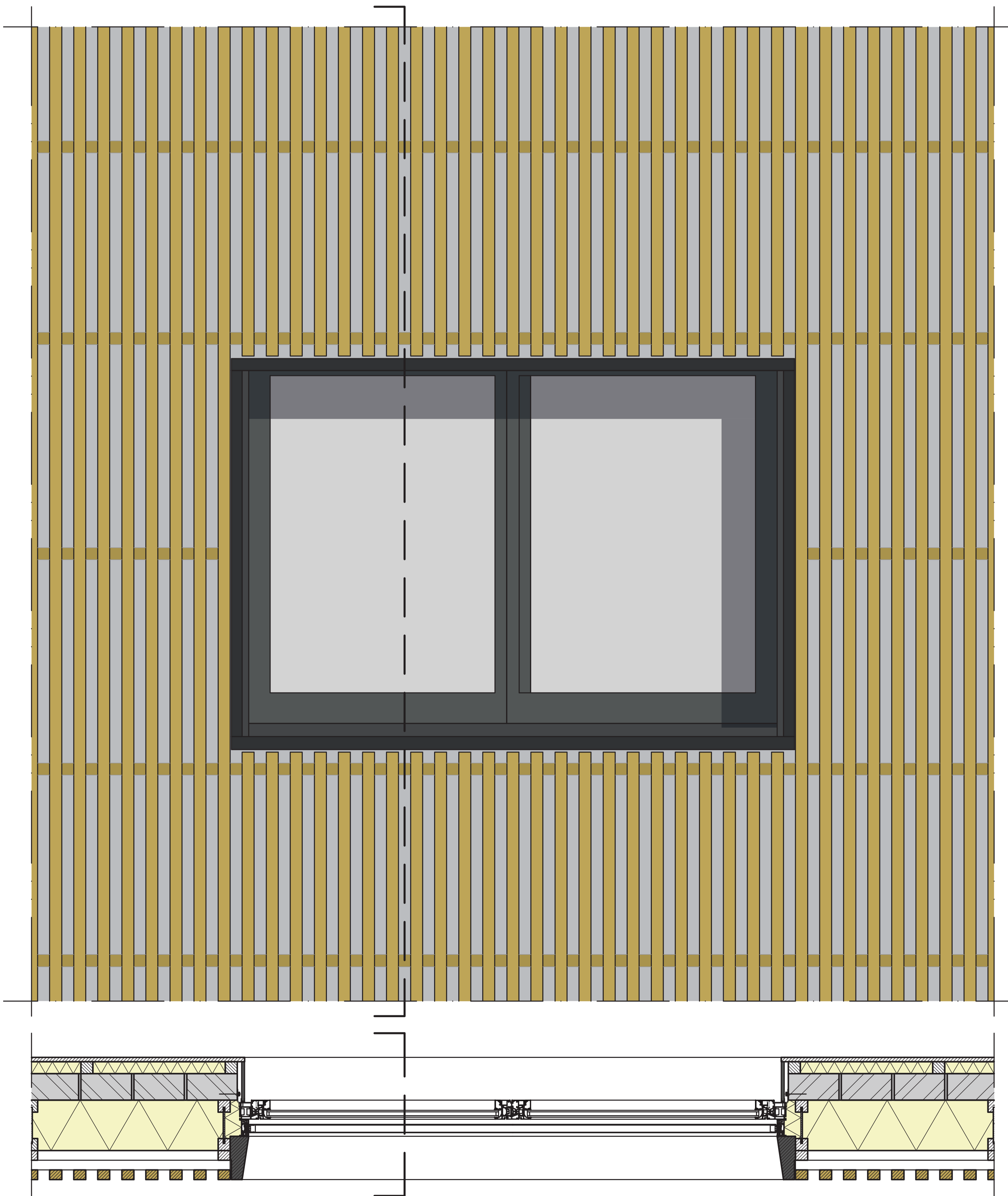
details gevel 1:10
