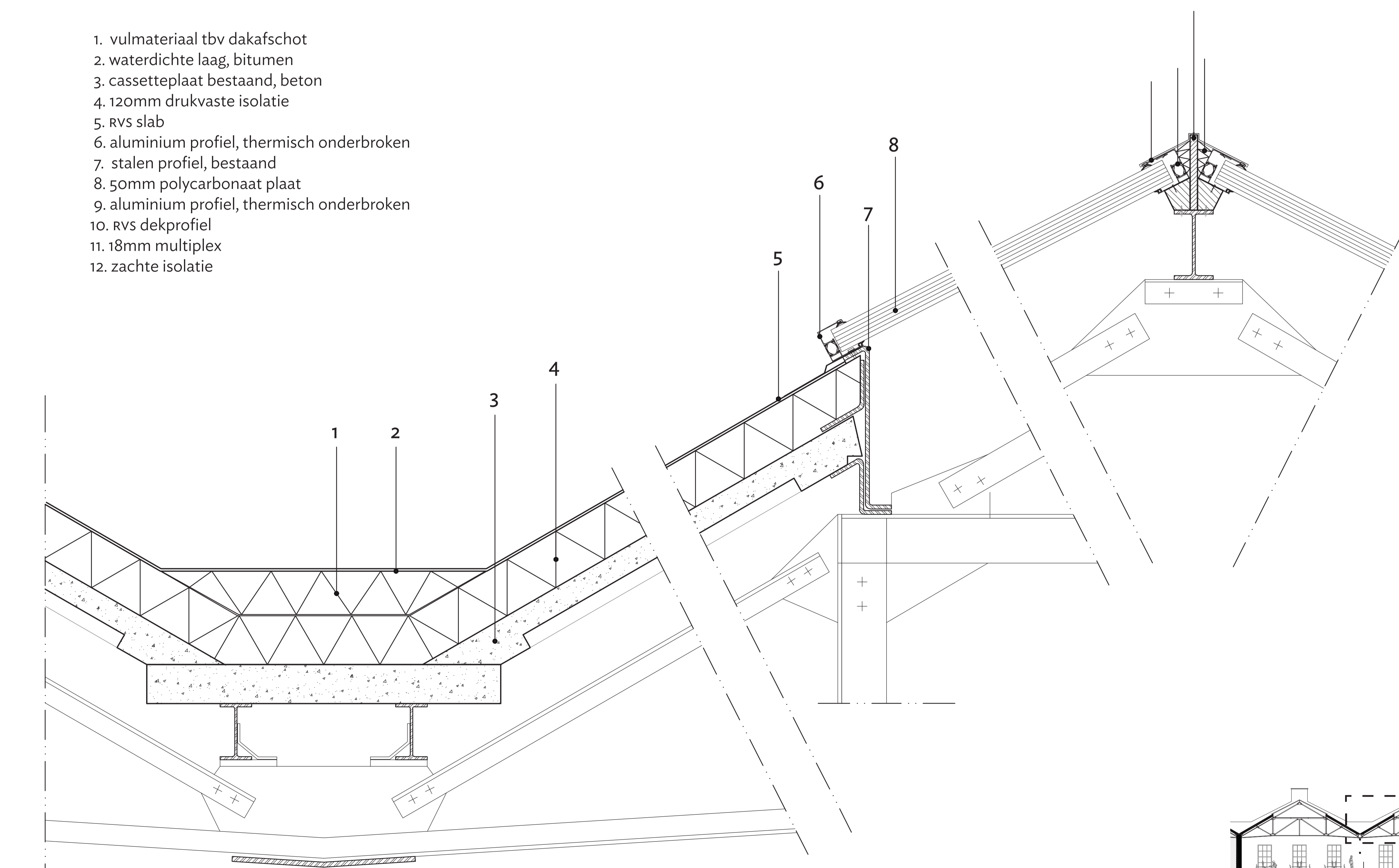
detail dak FABRIEK 1:5
