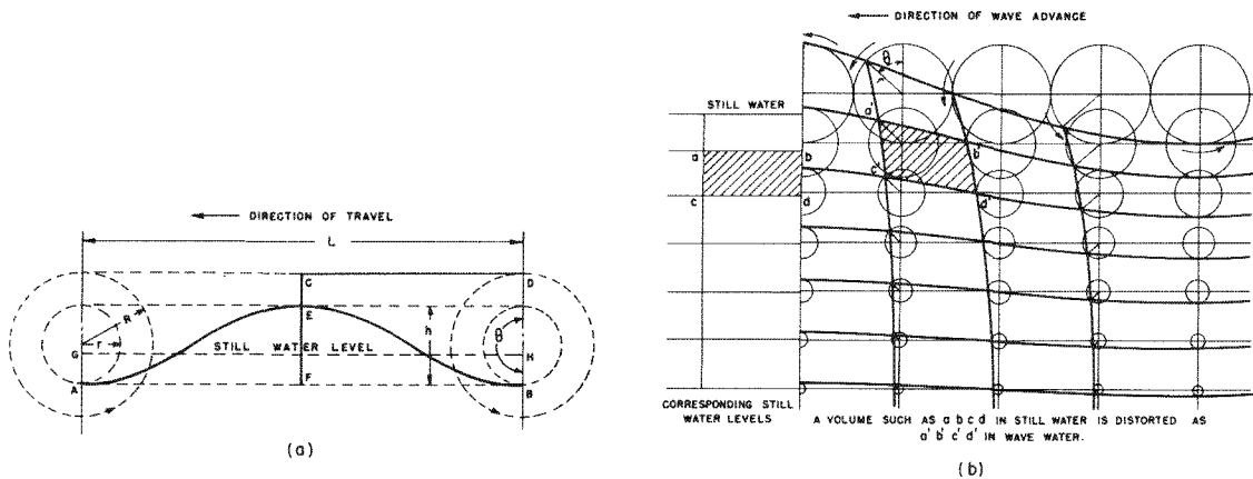
Fig. 12. Trochoidal Wave.
