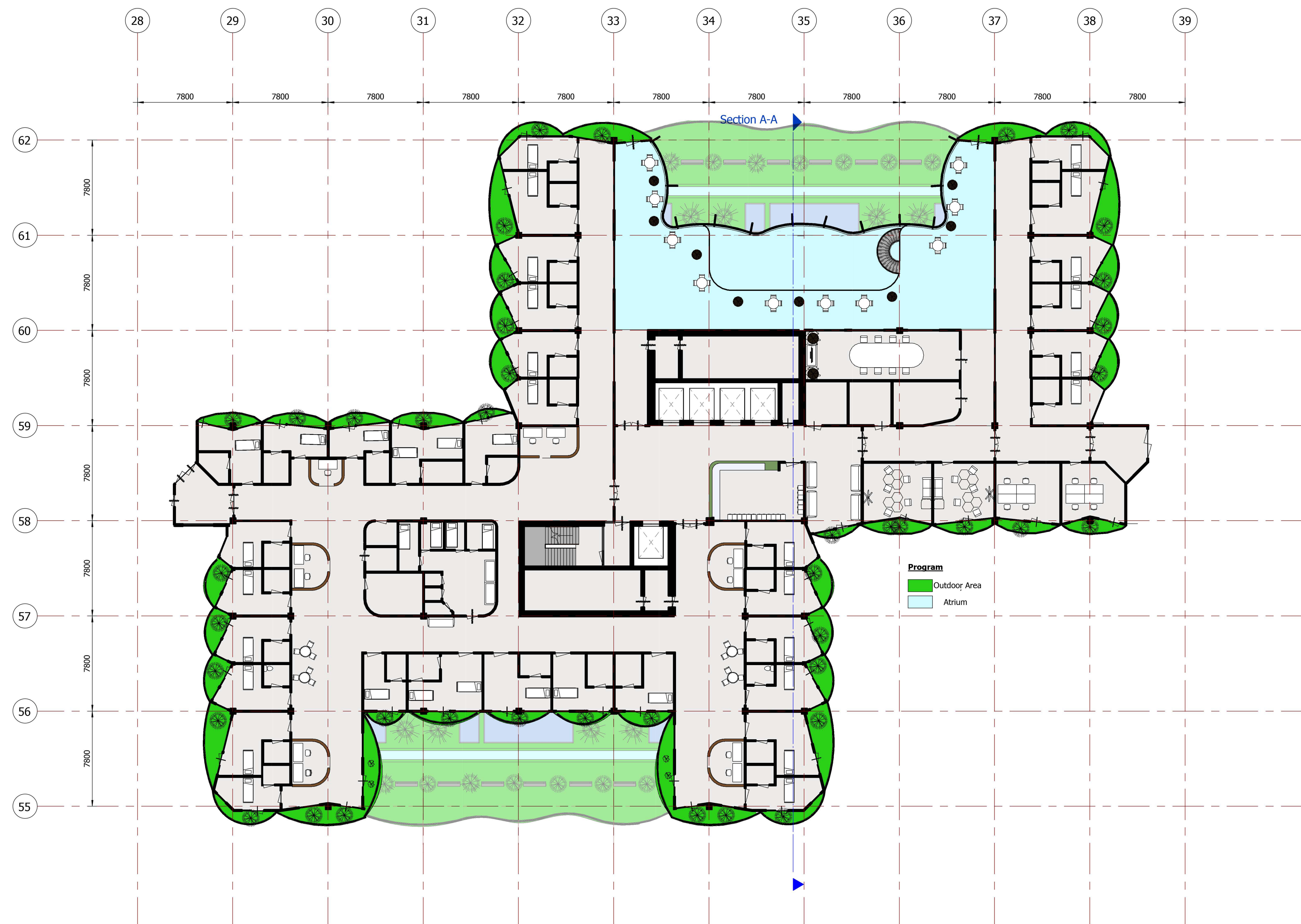
3 Level 8 1 : 200
