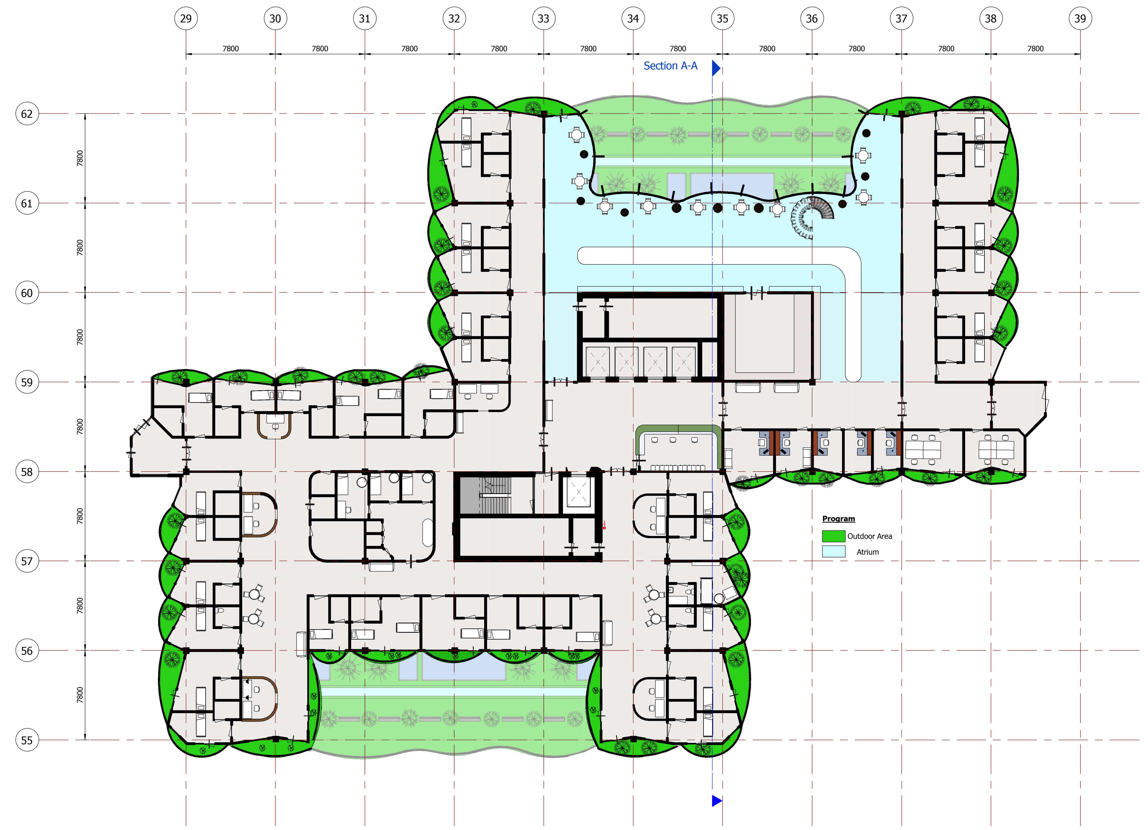
2 Level 7 1 : 200
