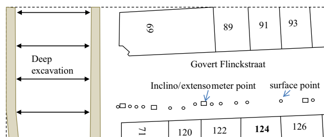
Fig. 15. Top view of deep excavation and buildings Govert Flinckstraat (Ceintuurbaan)
