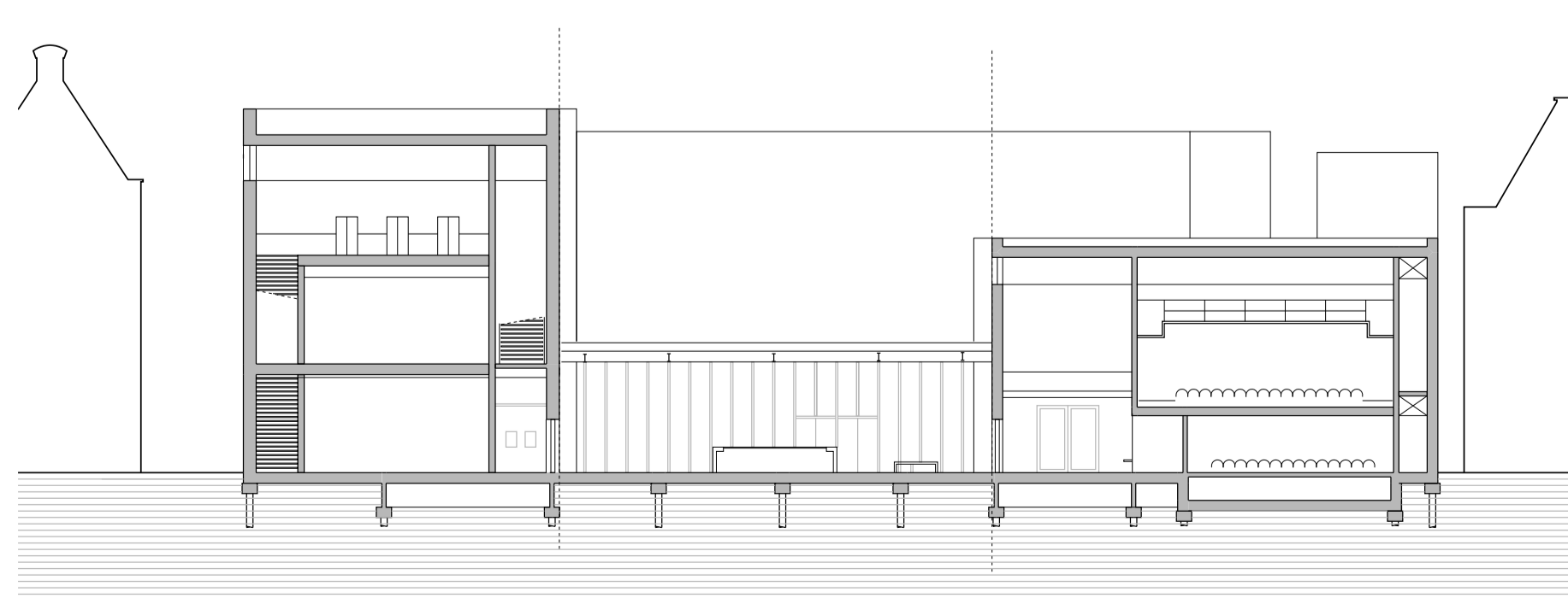
doorsnede A schaal 1: 300
