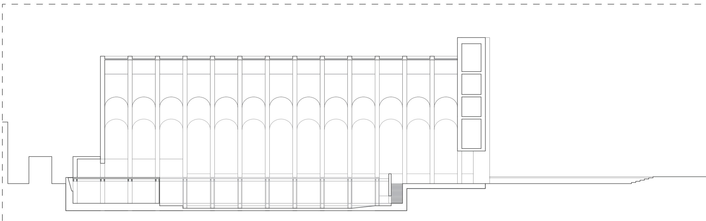
C'-C Section
