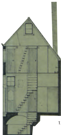
7.6.8. Doorsnede woningen, onderleggers
