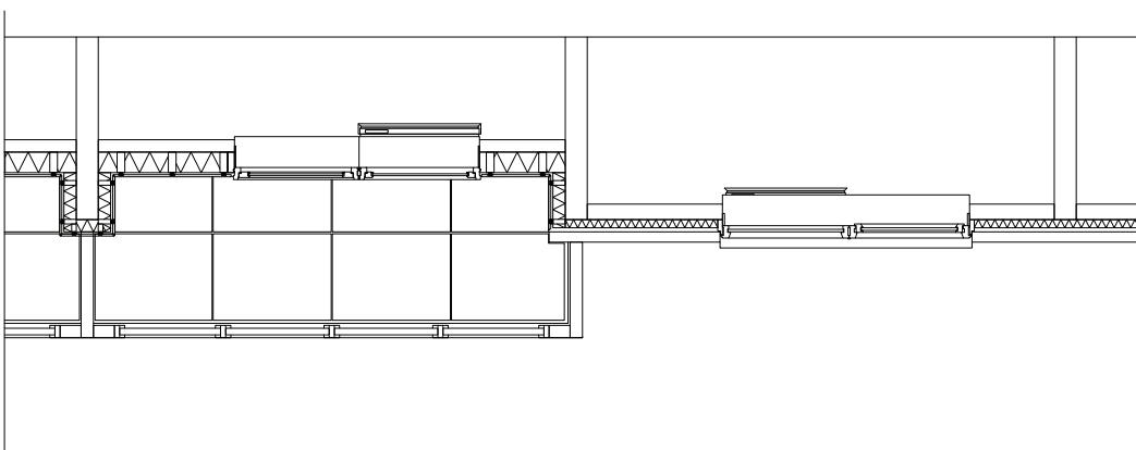
Gevelplattegrond 1:20
