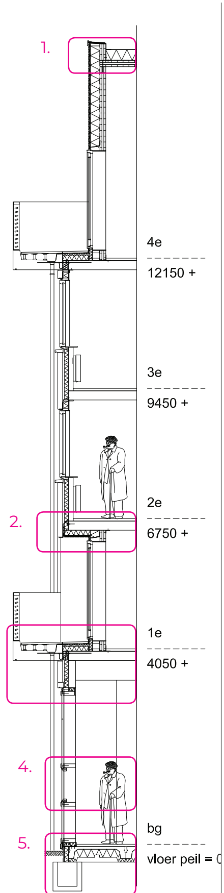
Geveldoornede 1:20
