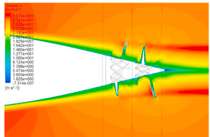
Fig. 21. The axial velocity contour [195].
