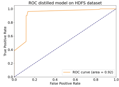
(d) HDFS dataset: Model with 14 states.
