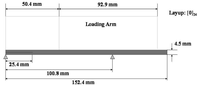
Fig. 8 MMB specimen.
