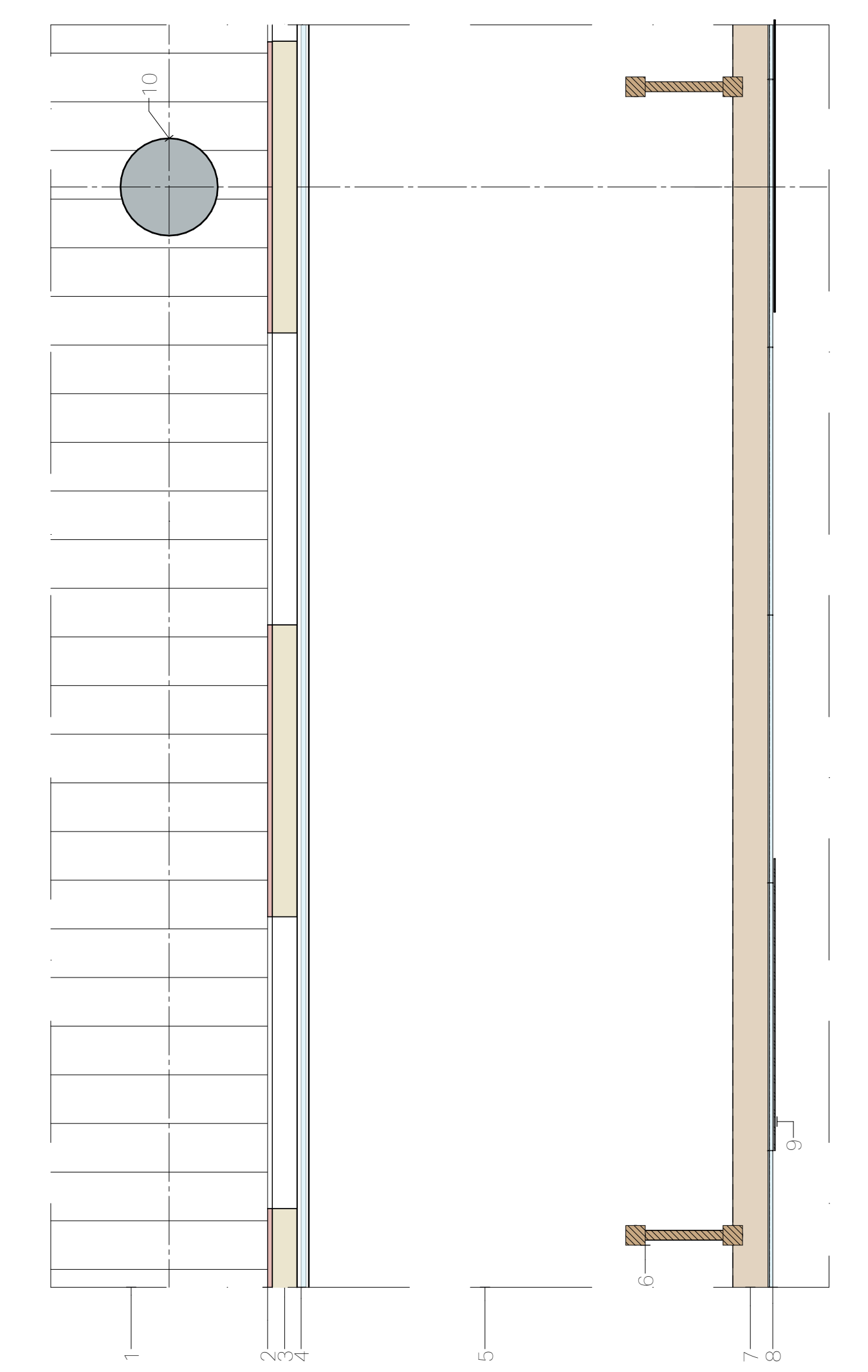
1:20 Façade
