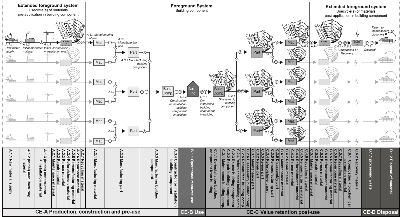
Fig. 3. CE-LCI Model.
