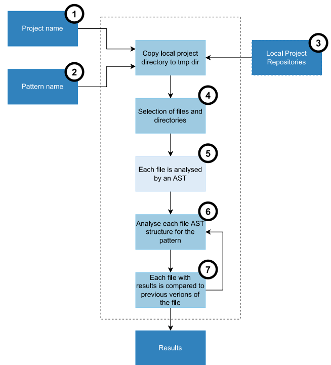
Fig. 4. AP-Spotter.
