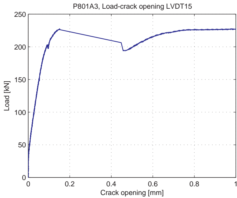
Fig. 5.85.10. Load-Crack opening for LVDT 15
