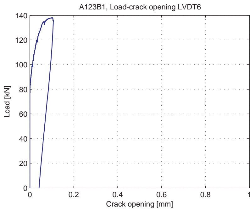
Fig. 5.10.7. Load-Crack opening for LVDT6
