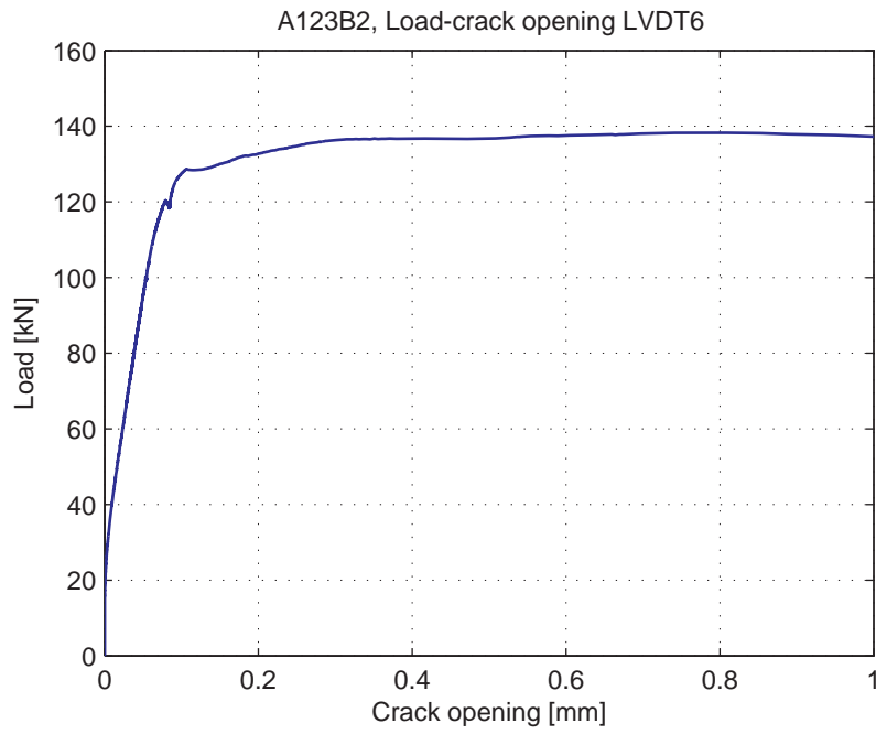
Fig. 5.11.7. Load-Crack opening for LVDT6
