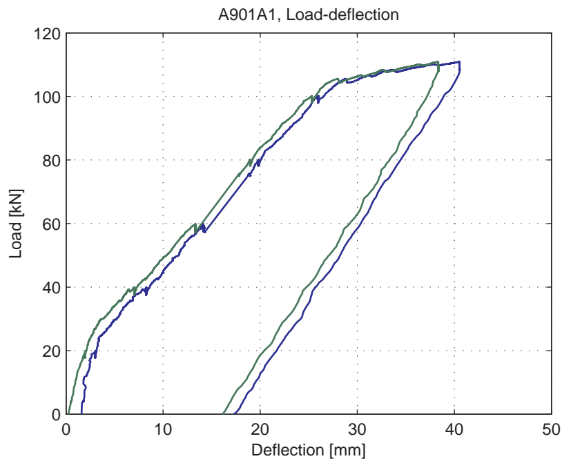
Fig. 5.12.4. Load-deflection curve
