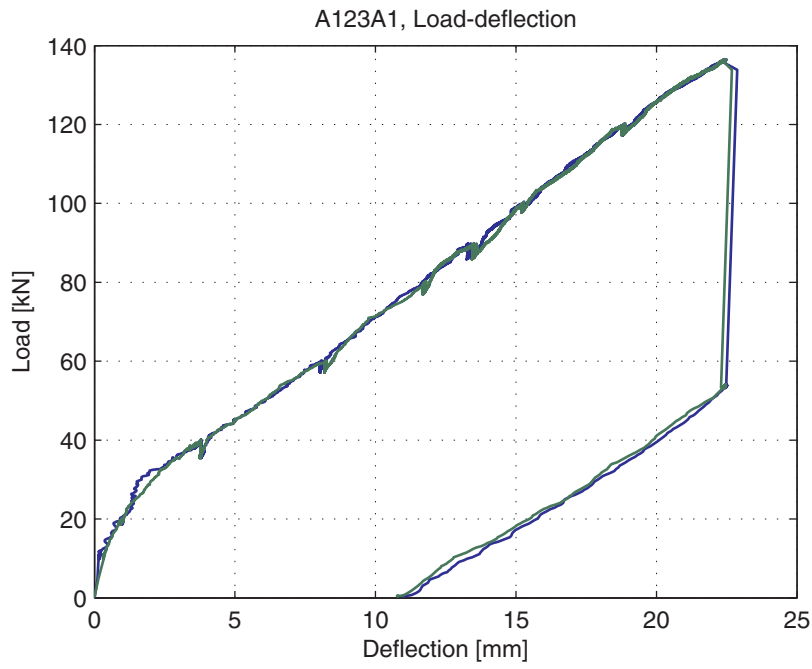
Fig. 5.8.4. Load-deflection curve
