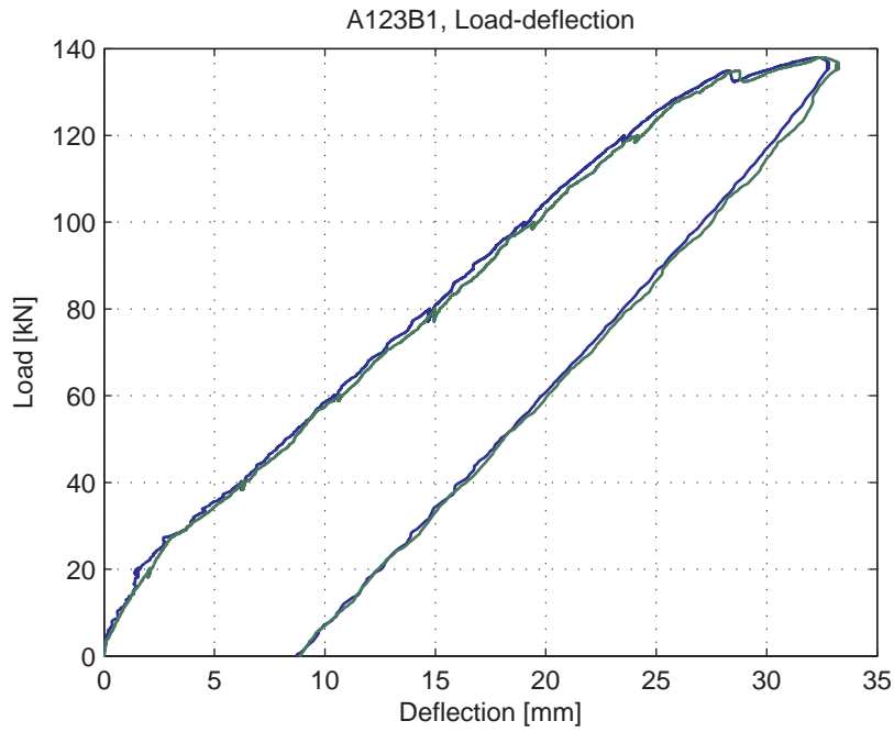
Fig. 5.10.4. Load-deflection curve
