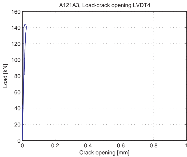
Fig. 5.3.8. Load-Crack opening for LVDT4
