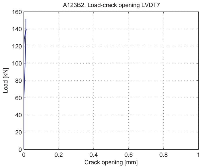
Fig. 5.11.8. Load-Crack opening for LVDT7
