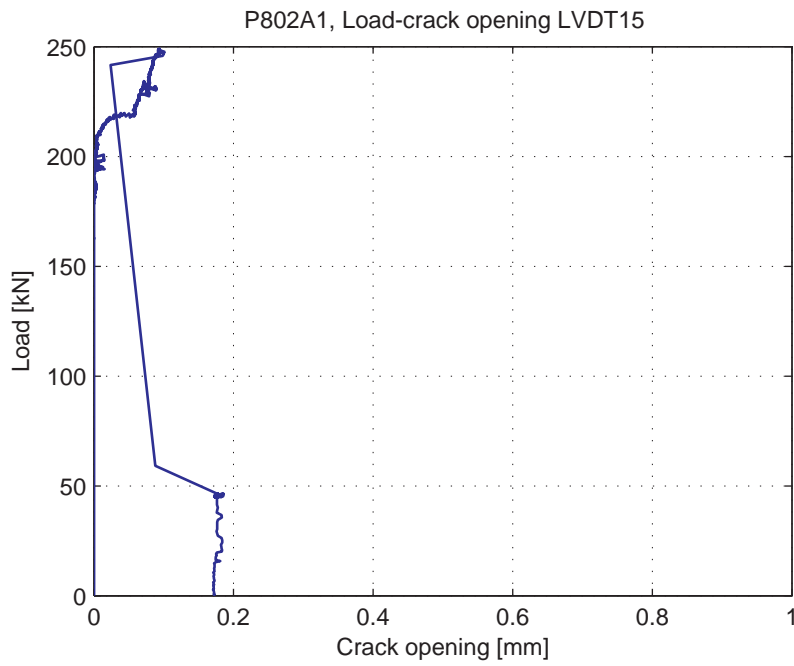
Fig. 5.87.10. Load-Crack opening for LVDT15
