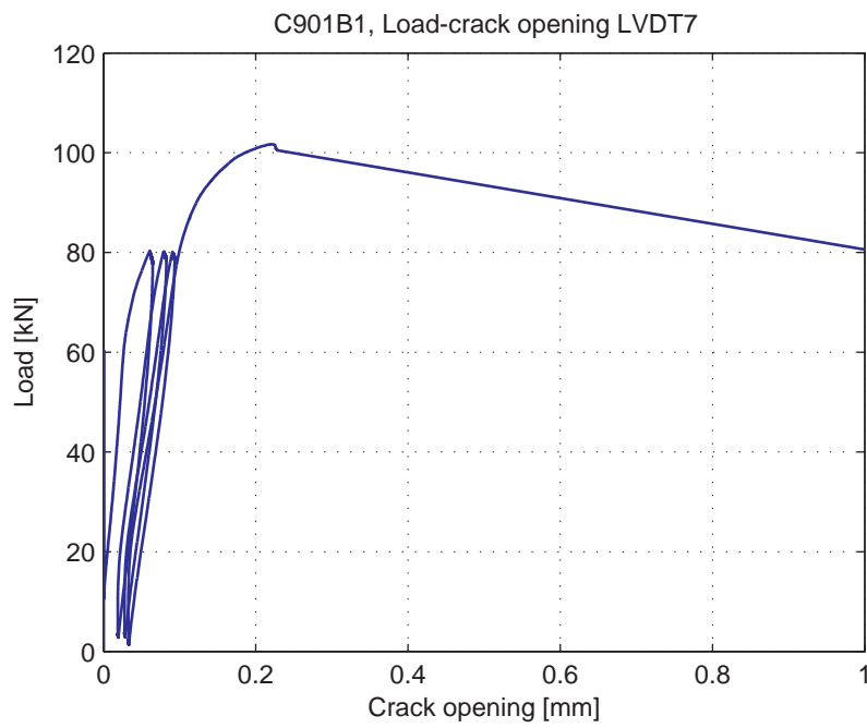
Fig. 5.57.10. Load-Crack opening for LVDT7
