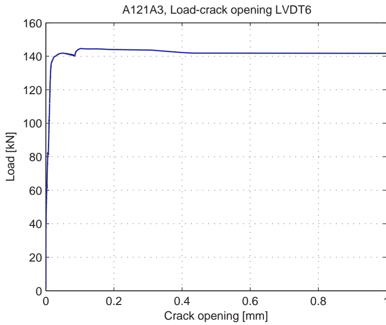
Fig. 5.3.10. Load-Crack opening for LVDT6
