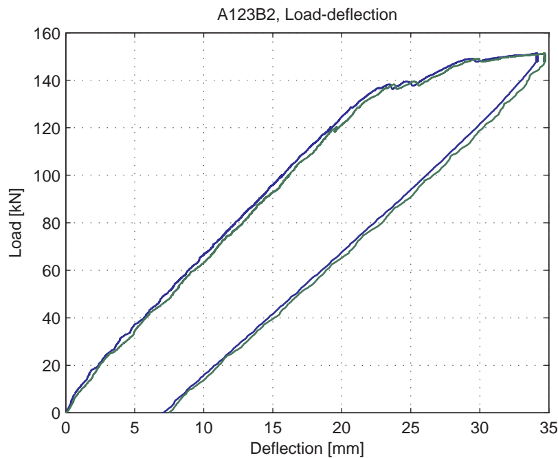
Fig. 5.11.4. Load-deflection curve
