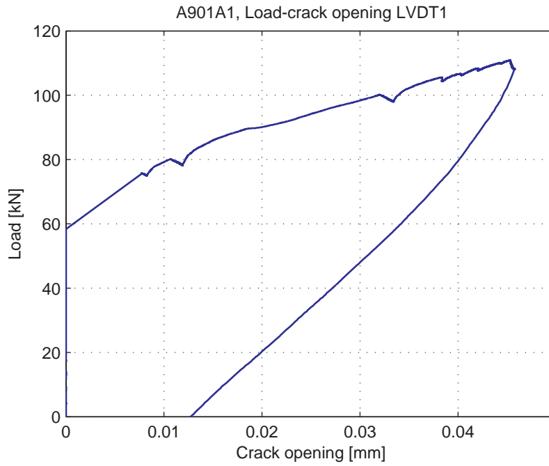
Fig. 5.12.5. Load-Crack opening for LVDT1
