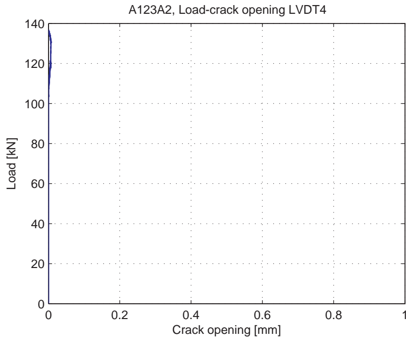
Fig. 5.9.5. Load-Crack opening for LVDT4
