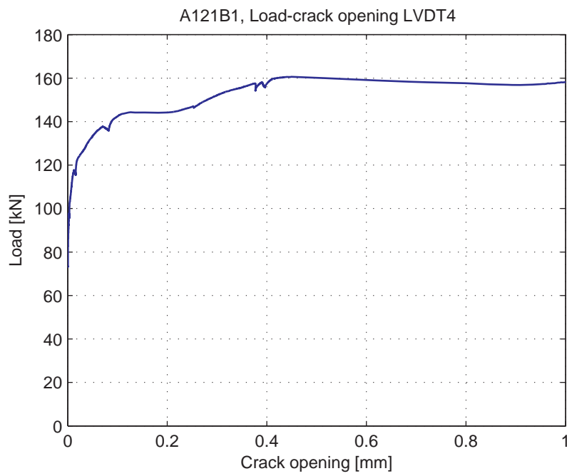
Fig. 5.4.8. Load-Crack opening for LVDT4
