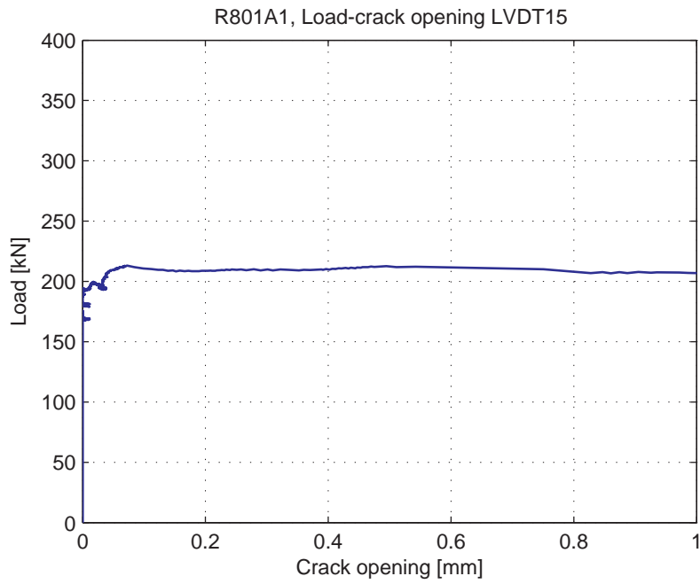
Fig. 5.100.10. Load-Crack opening for LVDT 15
