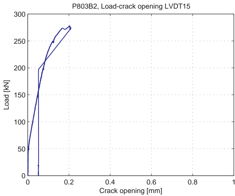
Fig. 5.91.10. Load-Crack opening for LVDT 15
