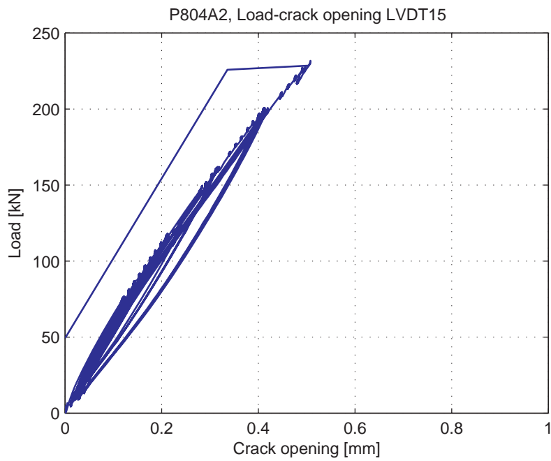
Fig. 5.93.10. Load-Crack opening for LVDT 15
