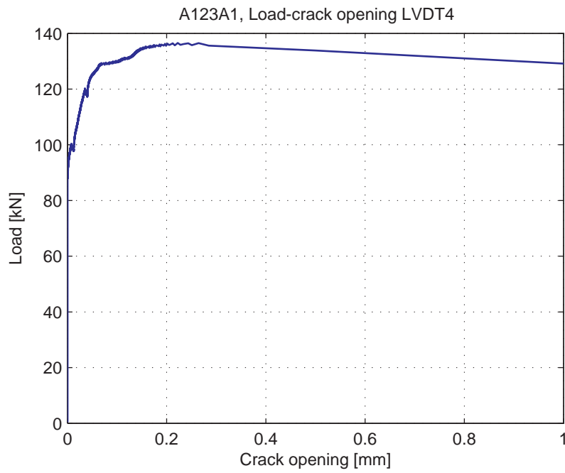
Fig. 5.8.5. Load-Crack opening for LVDT4
