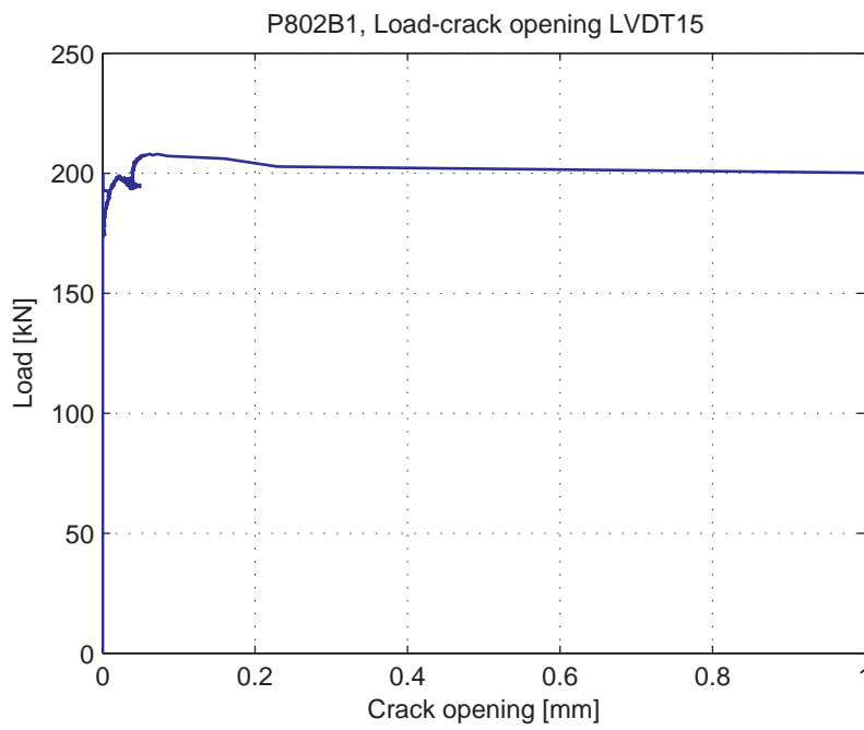
Fig. 5.88.10. Load-Crack opening for LVDT15
