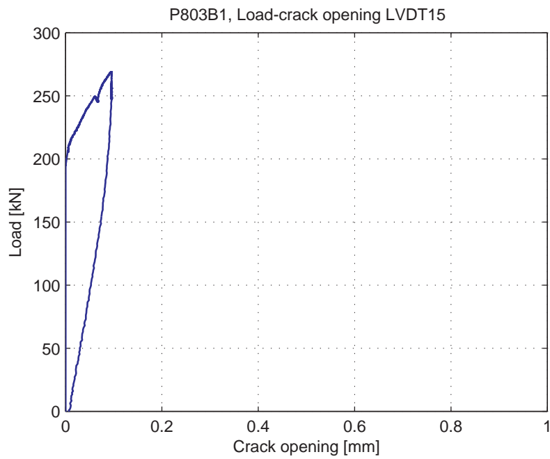
Fig. 5.90.10. Load-Crack opening for LVDT 15
