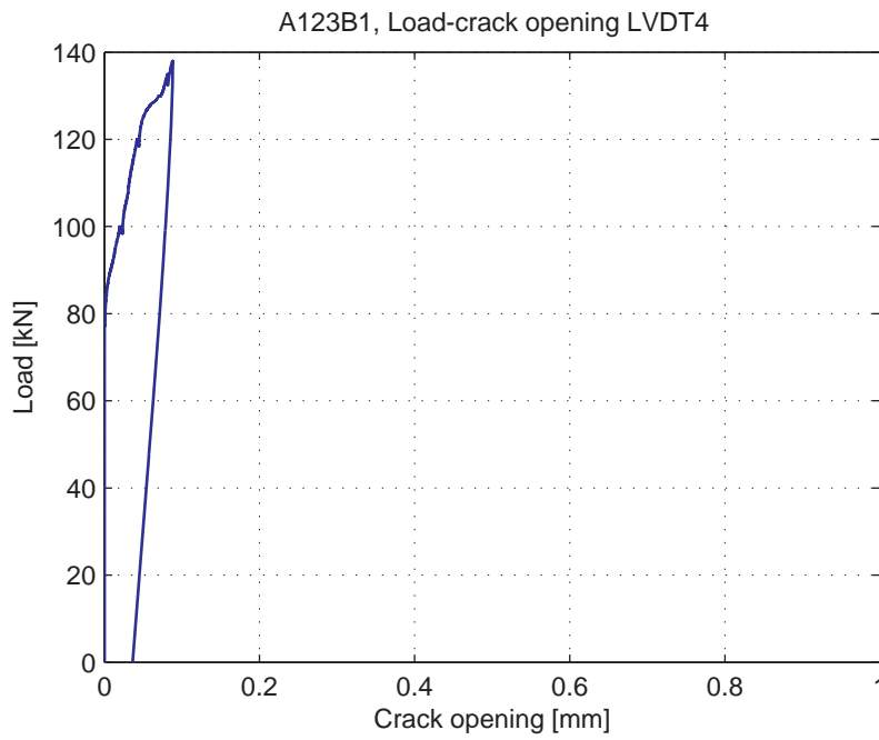
Fig. 5.10.5. Load-Crack opening for LVDT4
