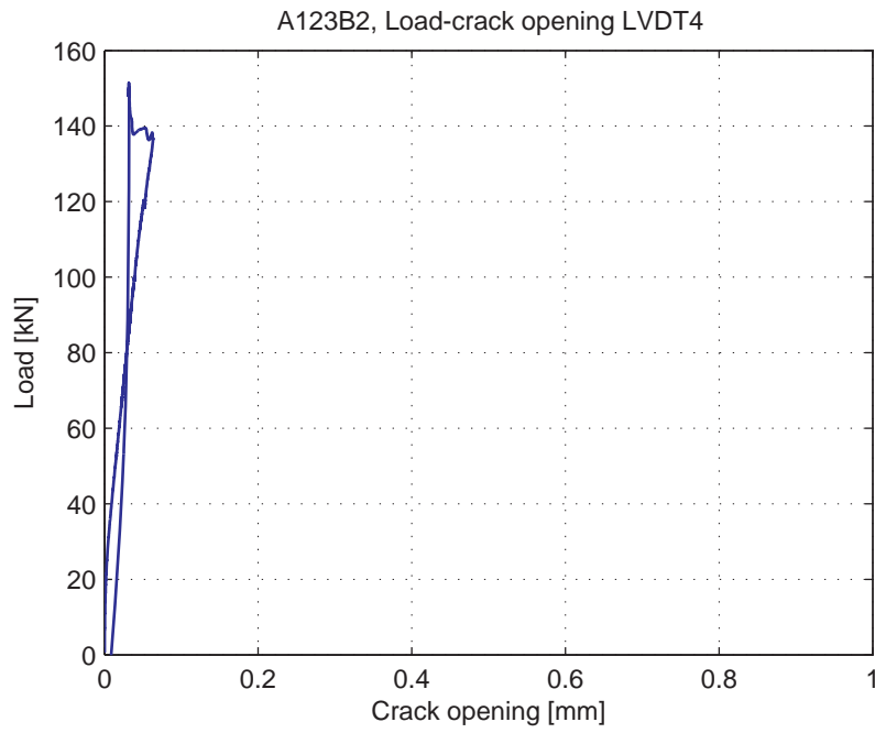
Fig. 5.11.5. Load-Crack opening for LVDT4
