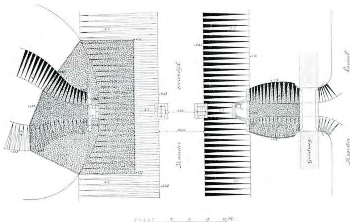
Fig. 56. Inlaatduiker bij Genderen. Situatie.
