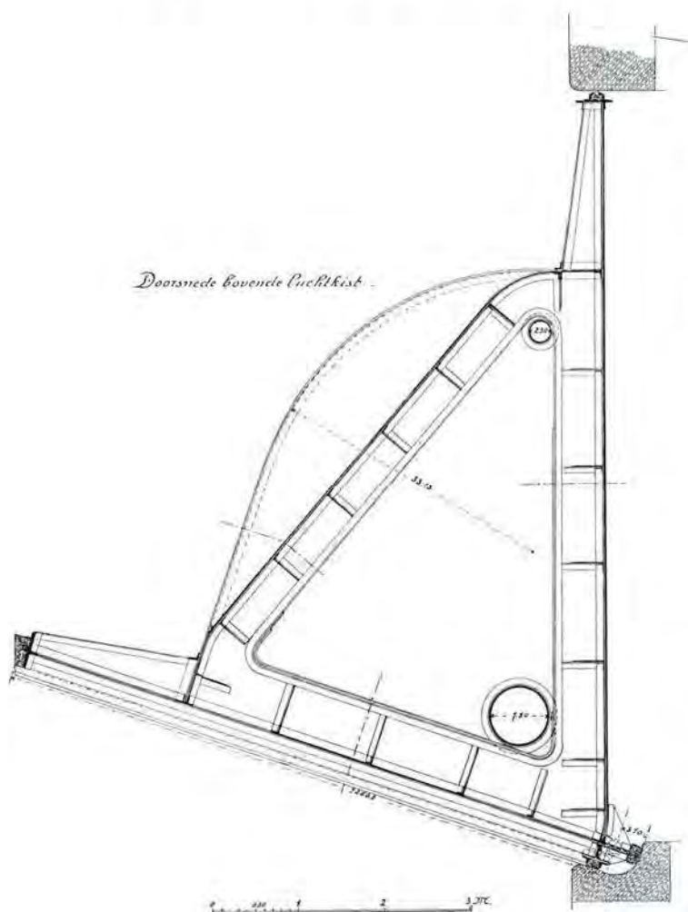
Fig. 70. De afsluitingswerken van de Maas bij Andel. Waaervlotdeur. Doorsnede.
