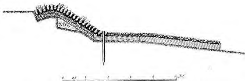
Fig. 8. Oevervoorziening op het benedendeel der rivier.
