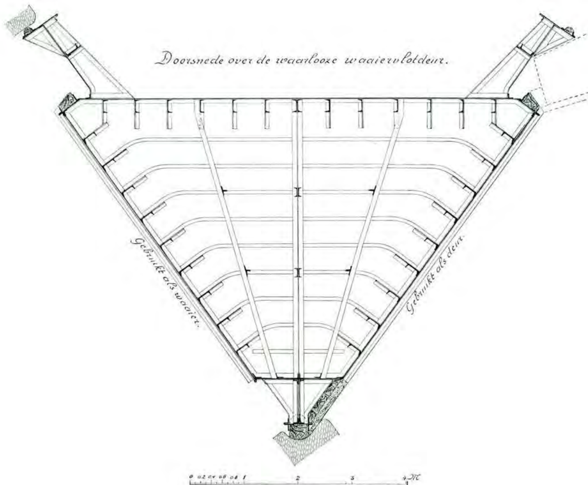
Fig. 71. De afsluitingswerken van de Maas bij Andel. Waarlooze deur.
