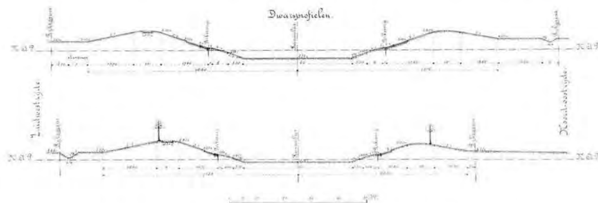
Fig. 60. Schipvaartkanaal Engelen-Henriëttewaard. Dwarsprofiel.
