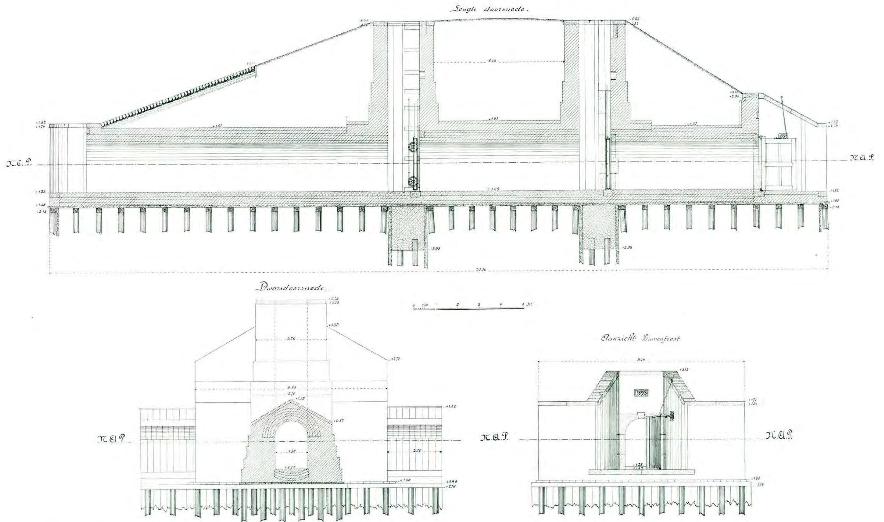
Fig. 57. Inlaatduiker bij Genderen. Samenstelling.
