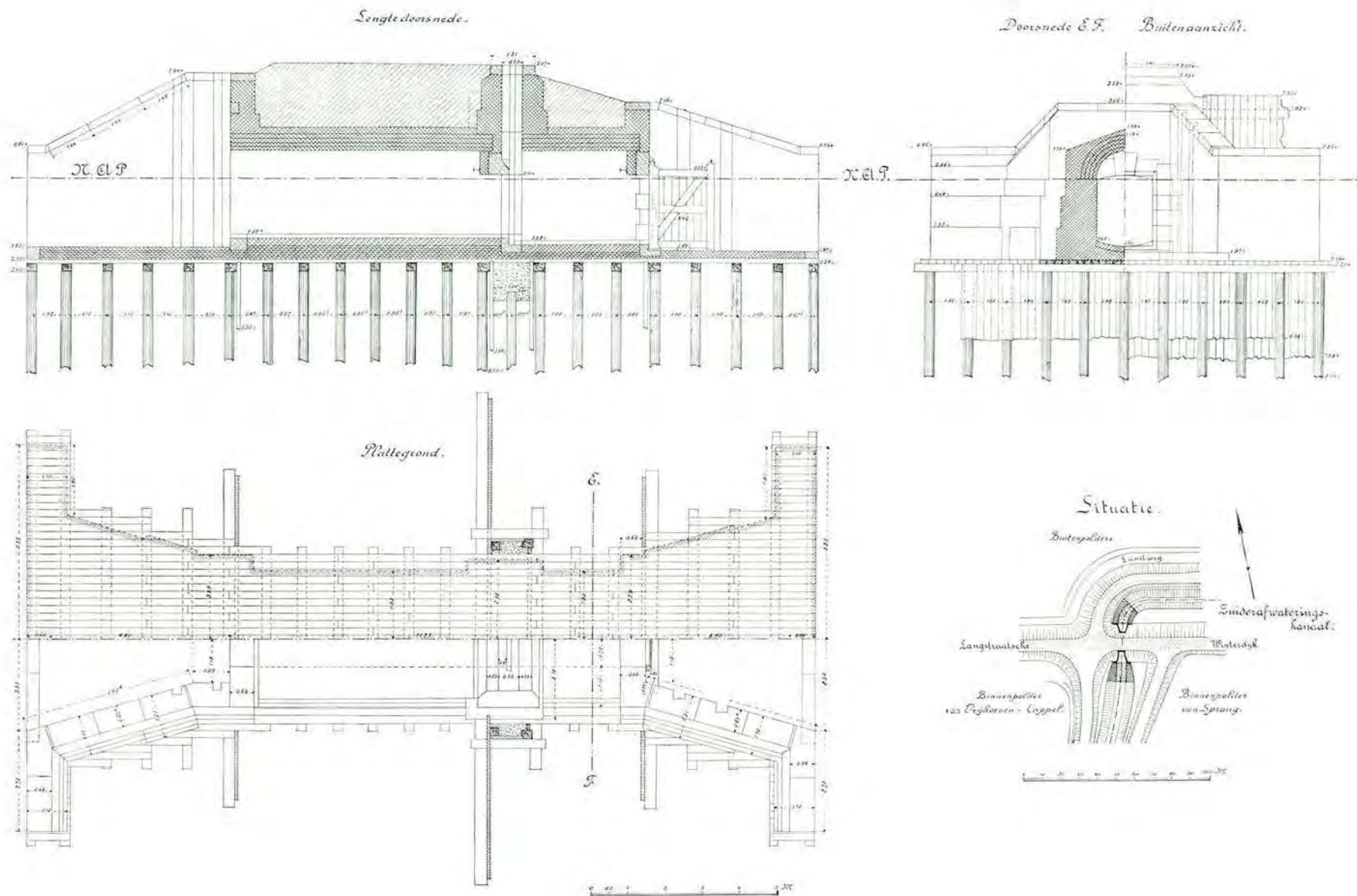
Fig. 46. Zuiderafwateringskanaal. Duikersluis in den Winterdijk.
