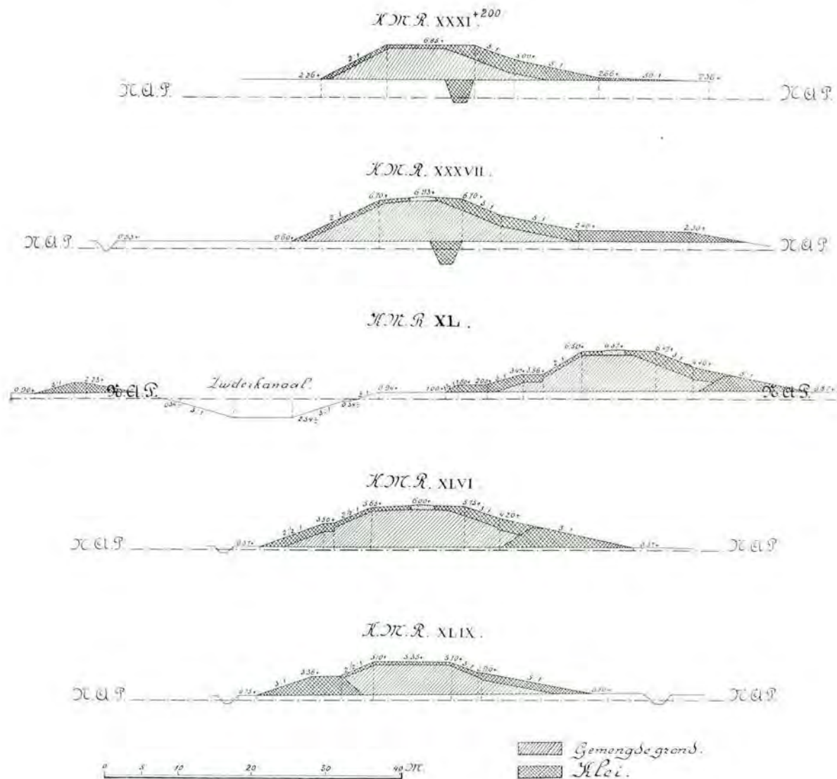
Fig. 4. Dwarsprofielen van den Zuiderrivierdijk.
