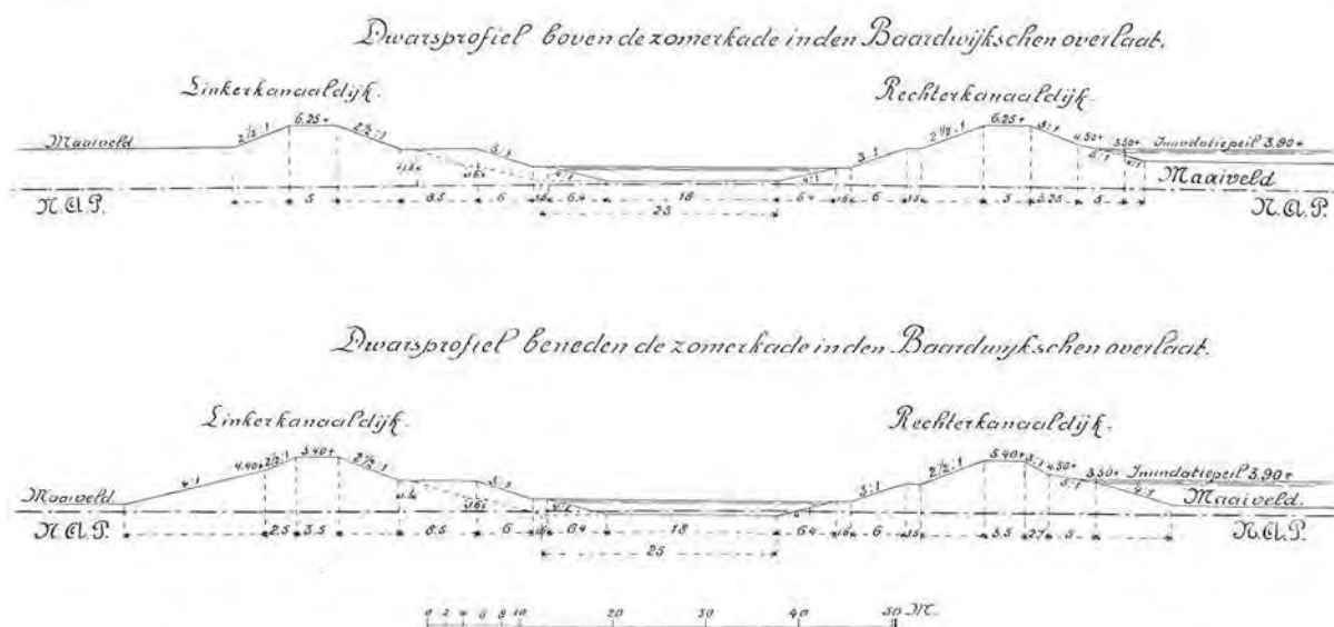
Fig. 79. Afwateringskanaal 's-Hertogenbosch-Drongelen. Dwaarsprofiel.
