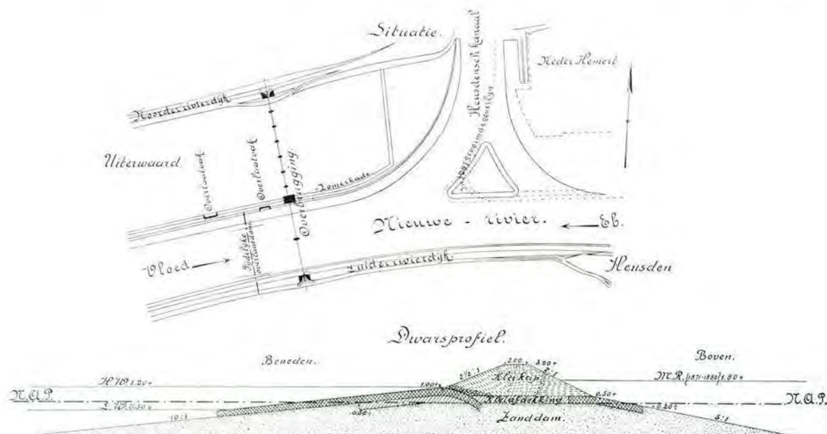
Fig. 75. Tijdelijke overlaatdam in de nieuwe rivier beneden Heusden.
