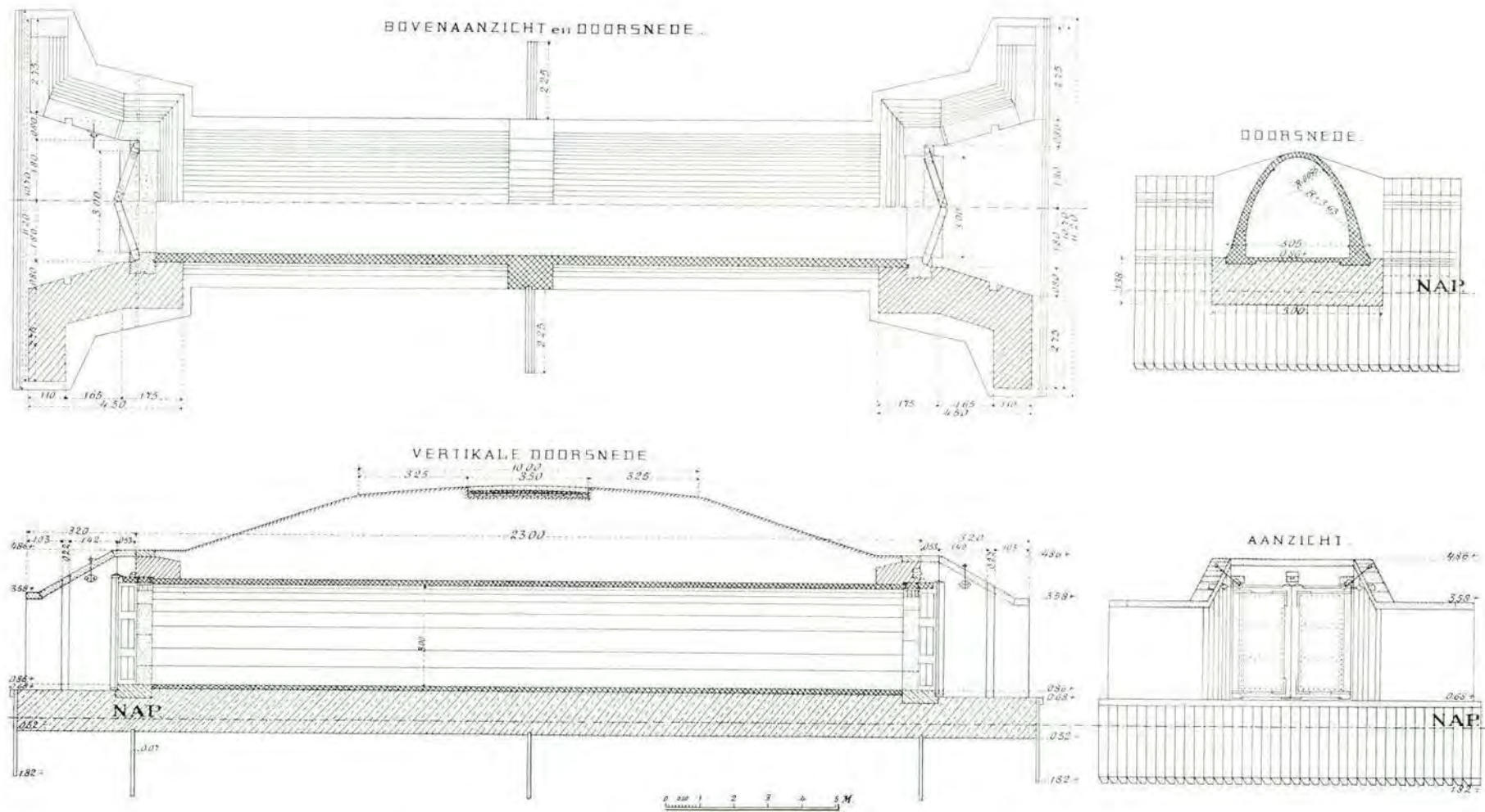
Fig. 10. Duiker van gewapend beton in den noorderleidijk op het eiland Nederhemert.
