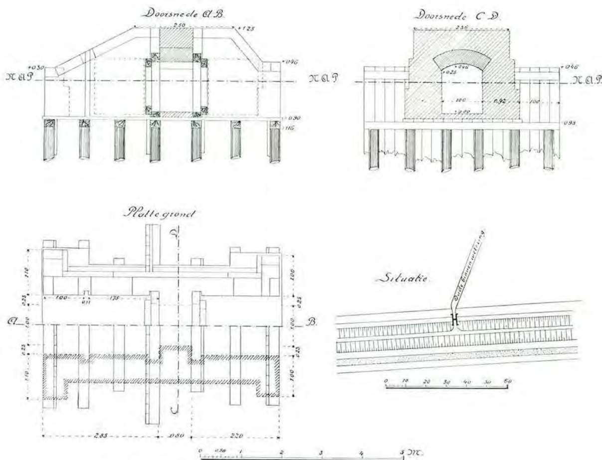
Fig. 32. Steenen duiker nabij de Oude Binnenwetering.
