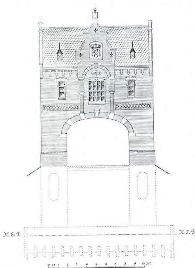
Fig. 29. Brug over het Heusdensch kanaal. Poortgebouw.
