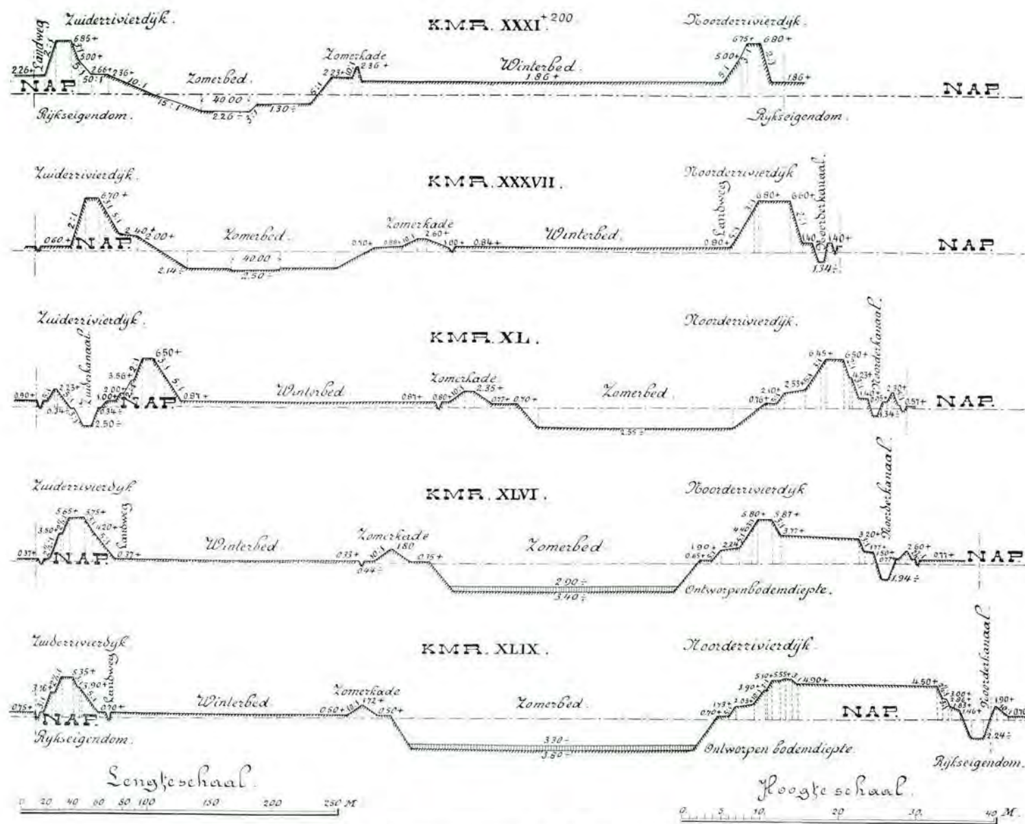
Fig. 2. Dwarsprofielen van de nieuwe rivier.
