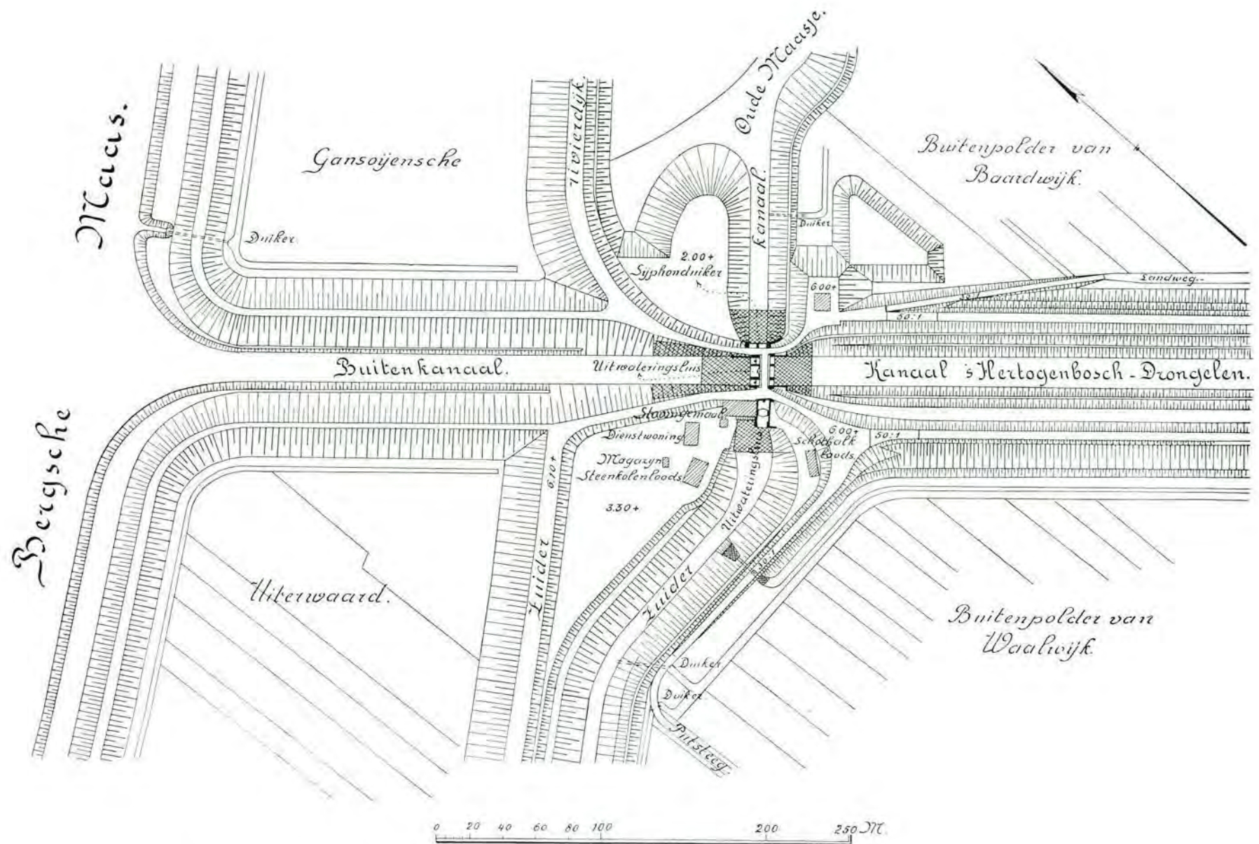
Fig. 40. Situatie van het Waalwijksche stoomgemaal en de werken aan den benedenmond van het afwateringskanaal 's-Hertogenbosch-Drongelen.
