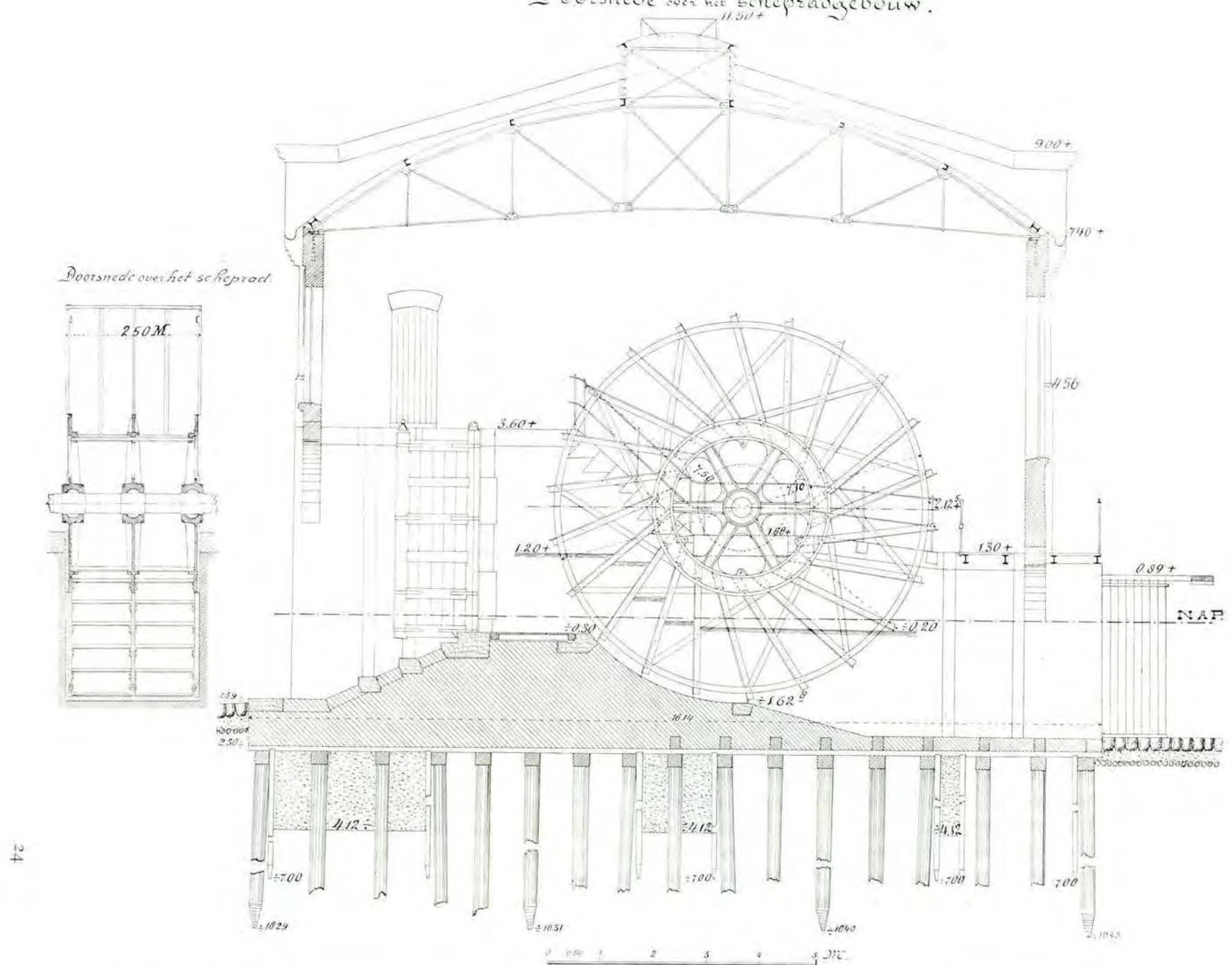
Fig. 49. Afsluitings- en bemalingswerken aan den benedenmond van het zuiderafwateringskanaal. Scheprad met gebouw.
