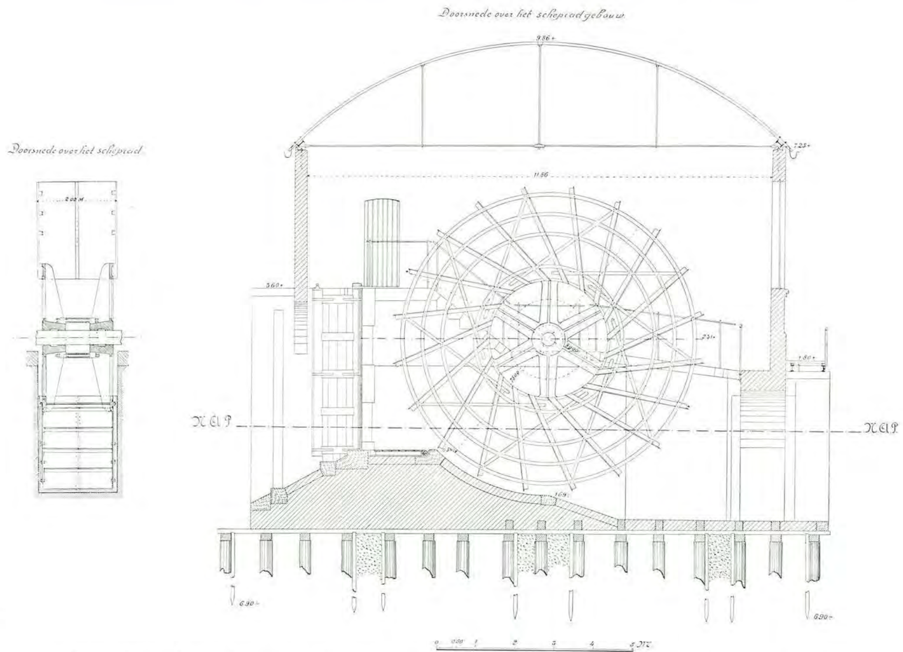
Fig. 39. Scheprad met gebouw van de afsluitings- en bemalingswerken aan den benedenmond van het noorderkanaal.
