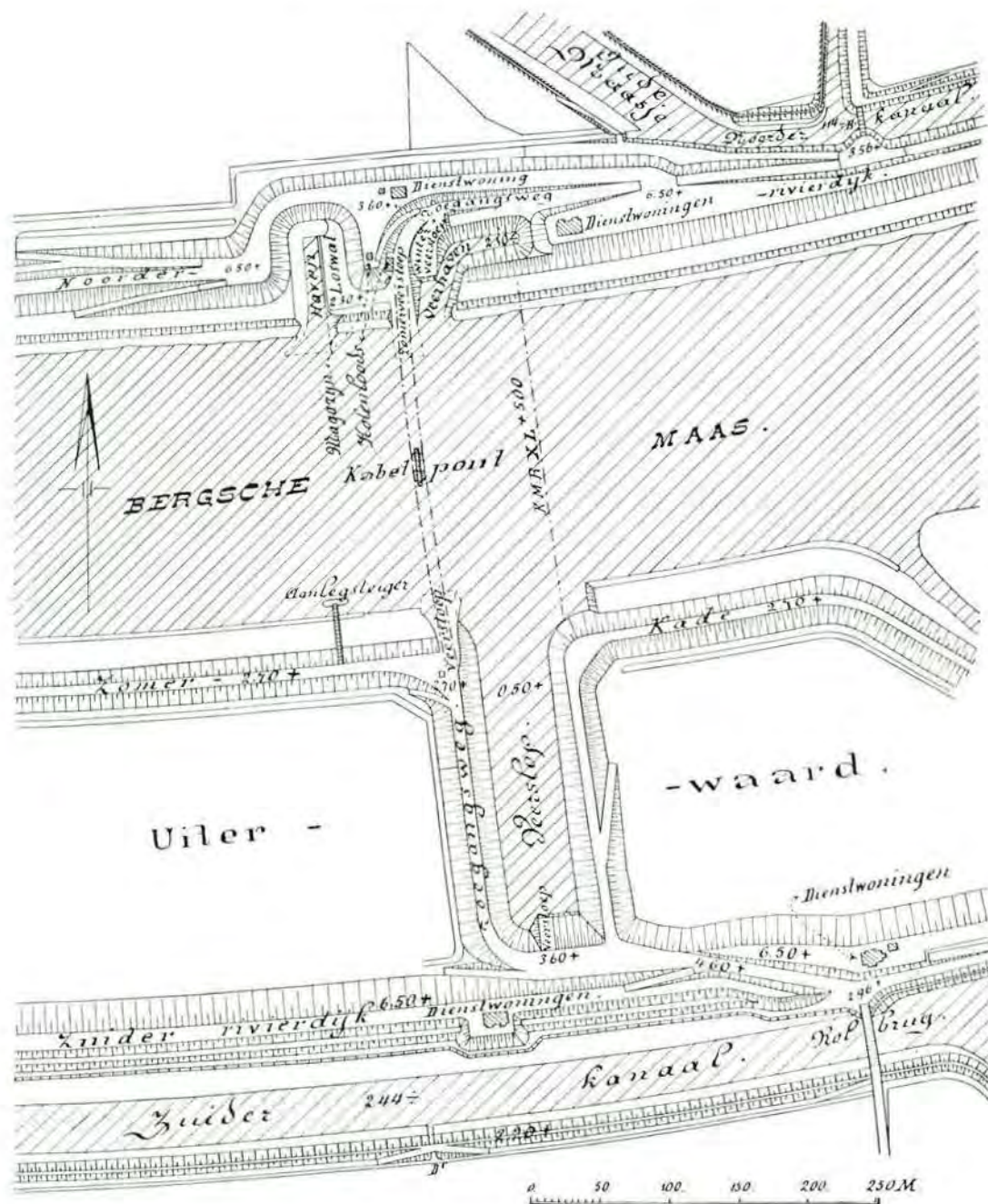
Fig. 15. Situatie van het Drongelensche veer.
