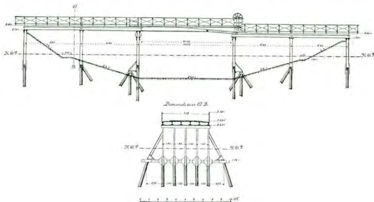
Fig. 20. Rolbrug onder Beroien.
