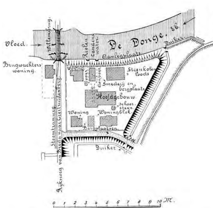
Fig. 50. Electrische bemaling van de Dongepolders. Situatie van het centraalstation.
