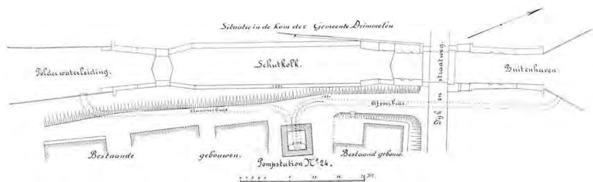
Fig. 53. Elektrische bemaling van de Dongepolders. Pompstation N o . 24.
