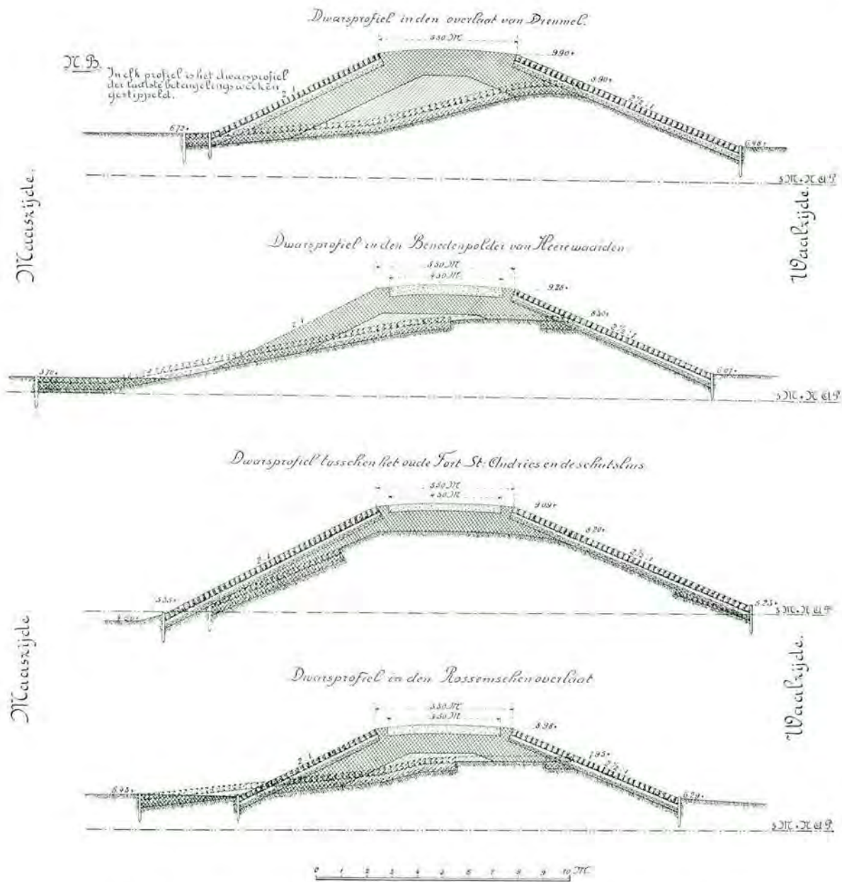
Fig. 64. De Heerewaardensche overlaten. Dwarsprofielen van den afsluitdijk.
