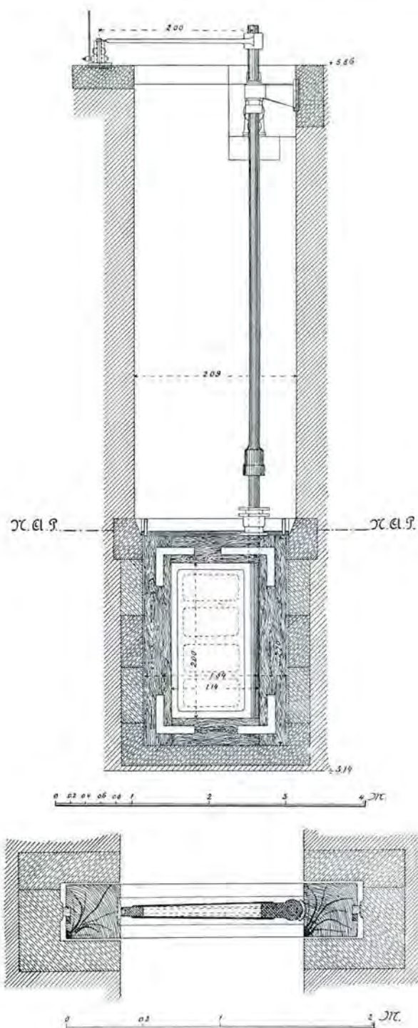
Fig. 68. De afsluitingswerken van de Maas bij Andel. Schutsluis. Aanzicht en horizontale doorsnede van de roerklep.
