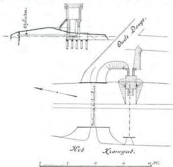
Fig. 52. Electrische bemaling van de Dongepolders. Type der pompstations.
