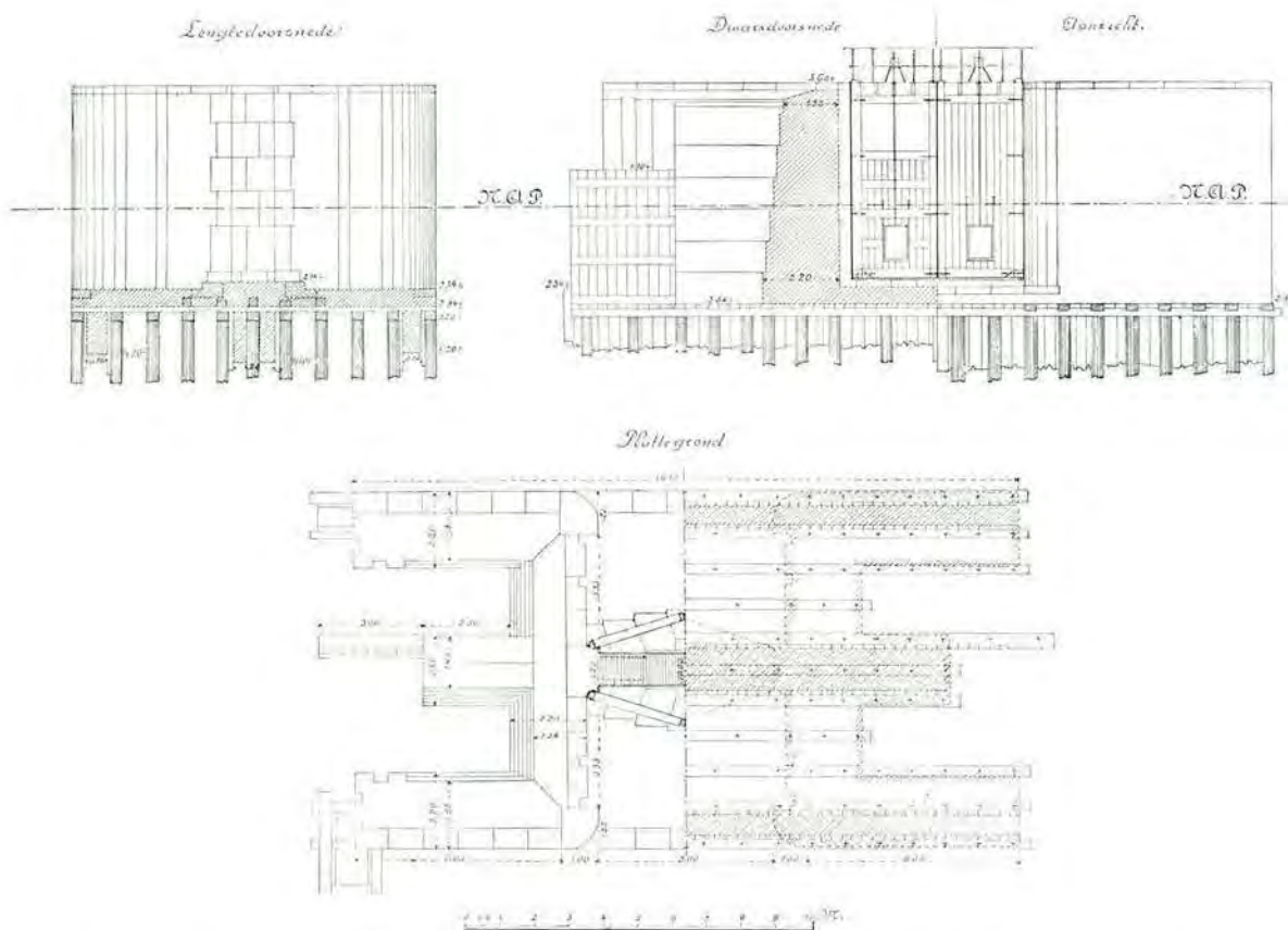
Fig. 38. Uitwaterings- en inlaatsluis van de afsluitings- en bemalingswerken aan den benedenmond van het noorderkanaal.
