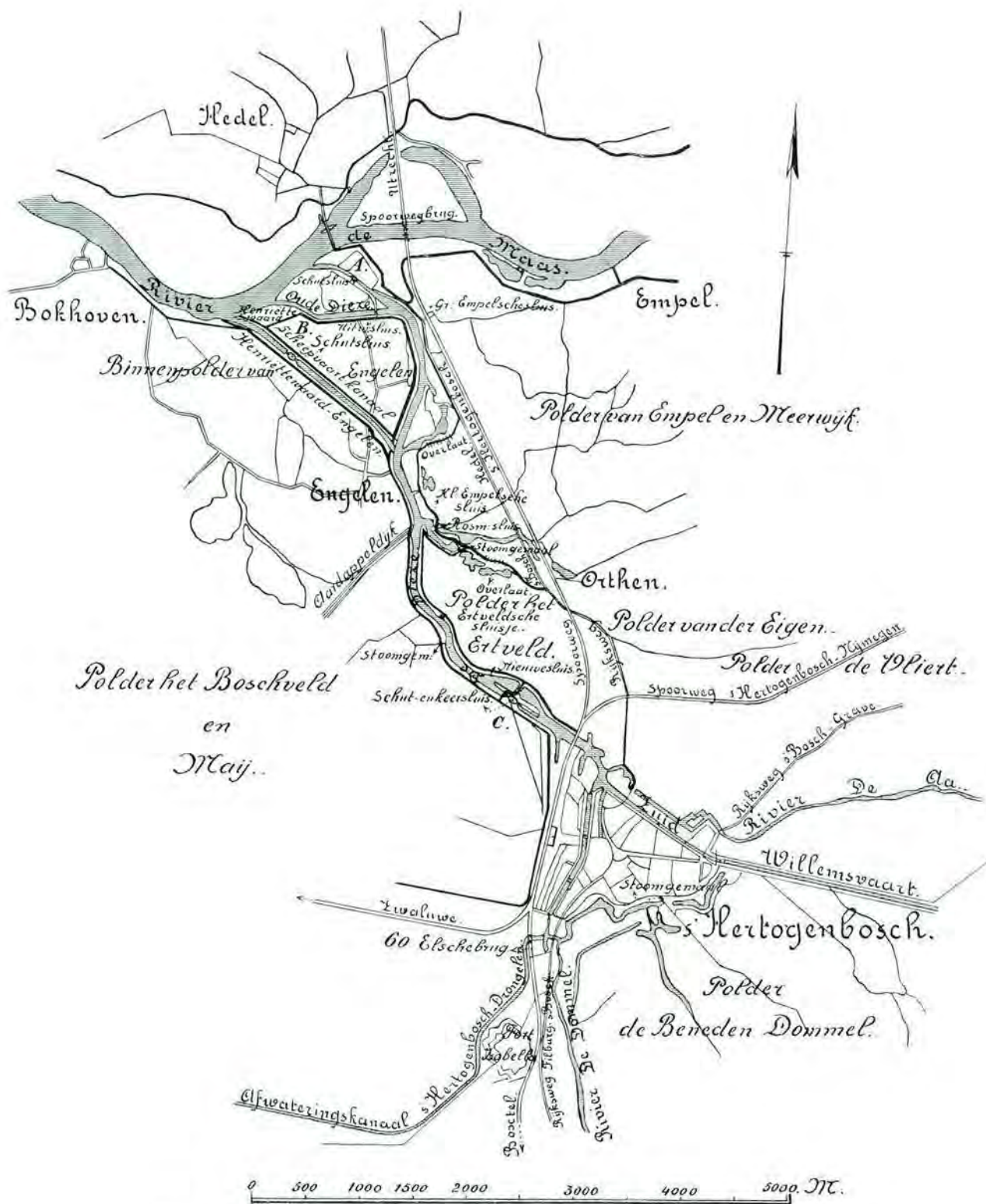
Fig. 59. De Dieze met het scheepvaartkanaal Engelen-Henriëttewaard.
