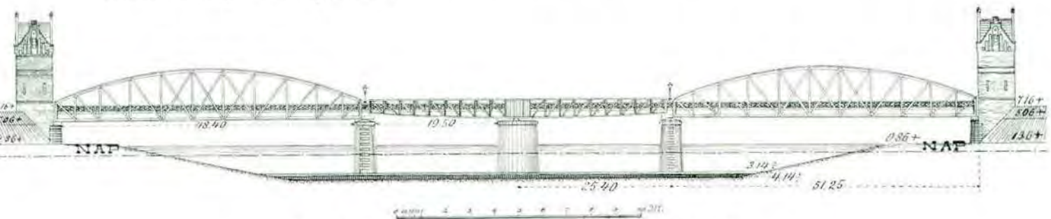
Fig. 26. Brug over het Heusdensch kanaal. Aanzicht.
