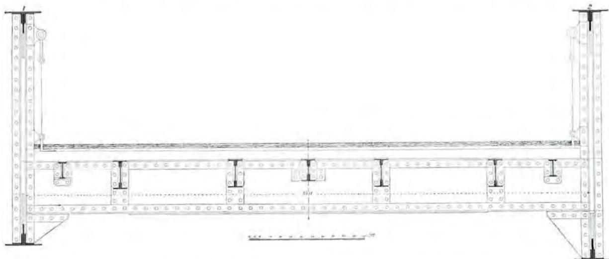
Fig. 28. Brug over het Heusdensch kanaal. Normale dwarsdoorsnede van de draaibrug.
