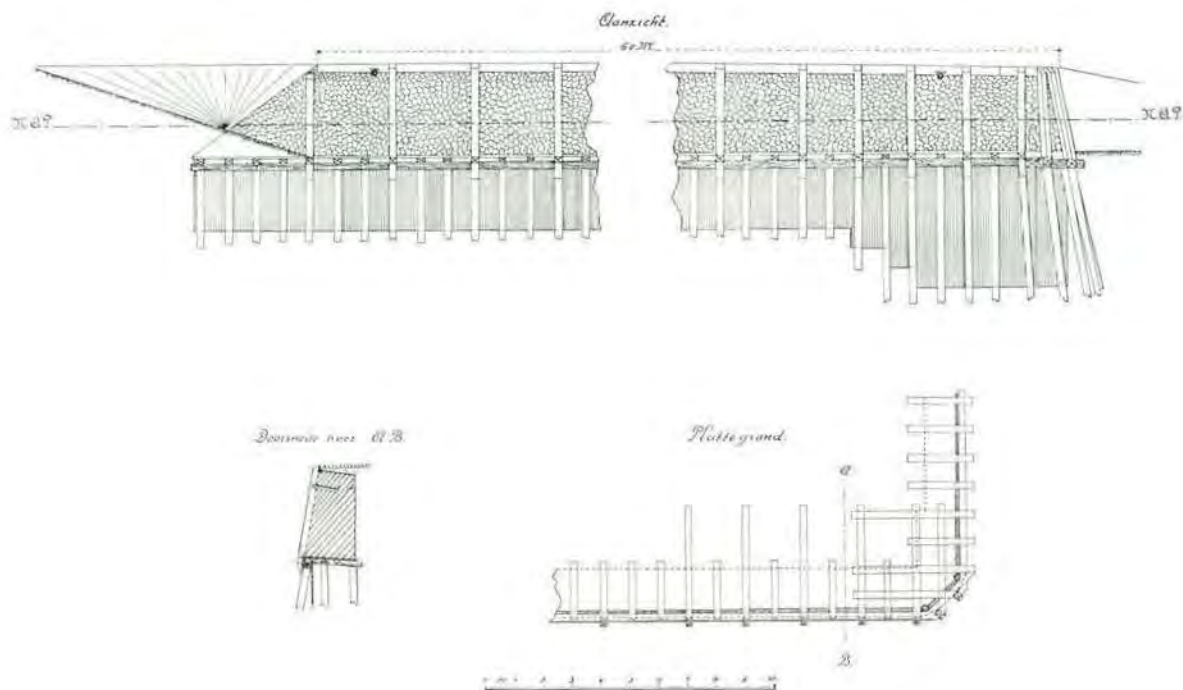
Fig. 6. Steenen loswal.
