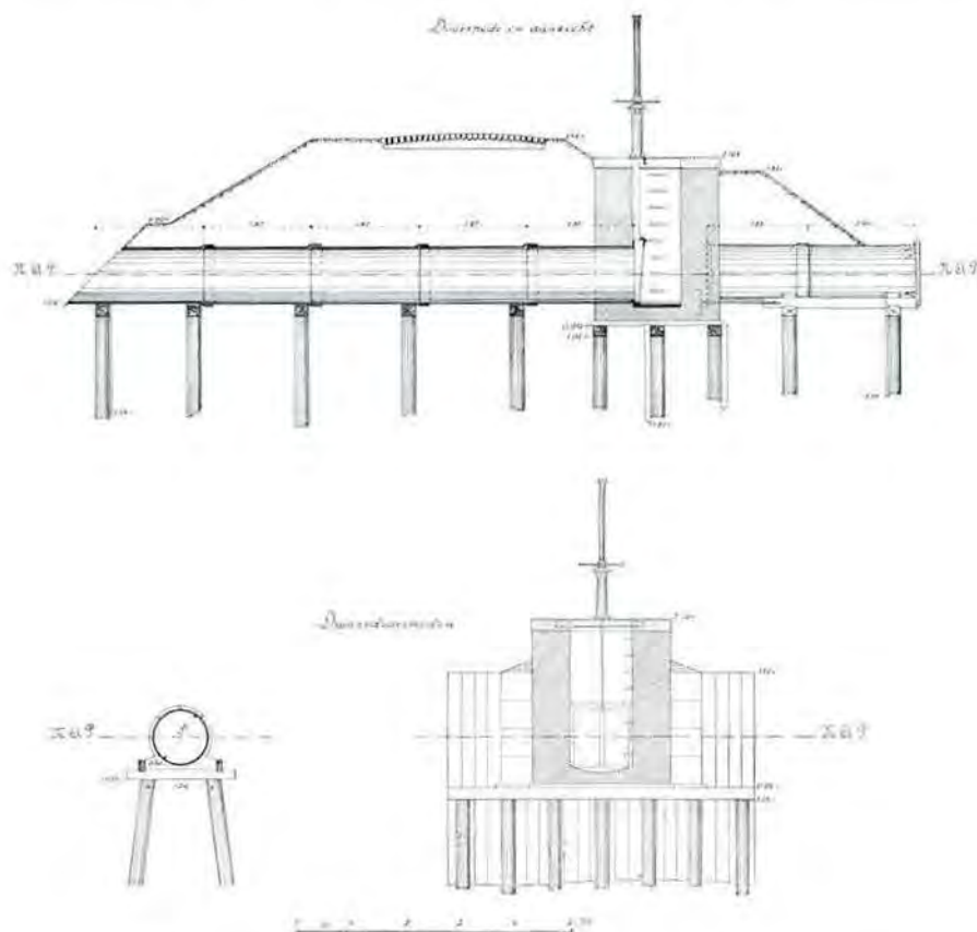
Fig. 33. IJzeren duiker aan de Dussensche Gantel.
