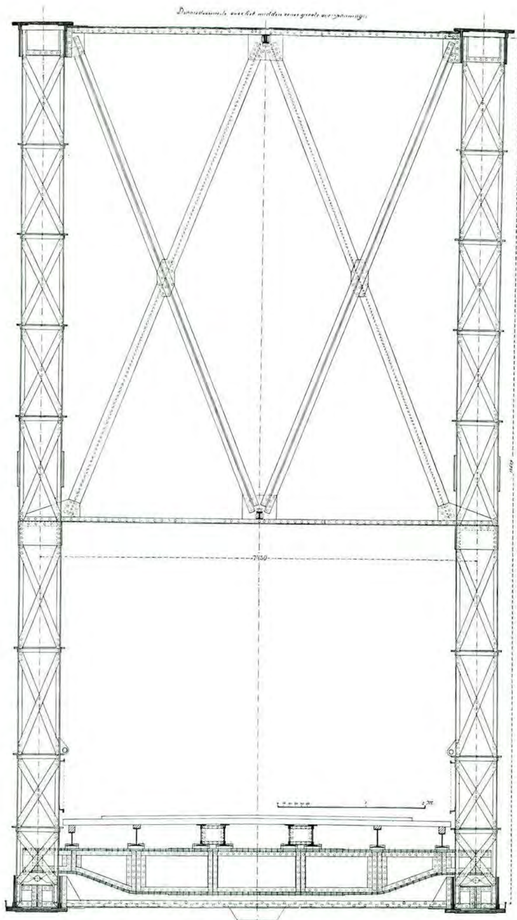
Fig. 24. Brug bij Heusden. Dwarsdoorsnede over het midden eener groote overspanning.
