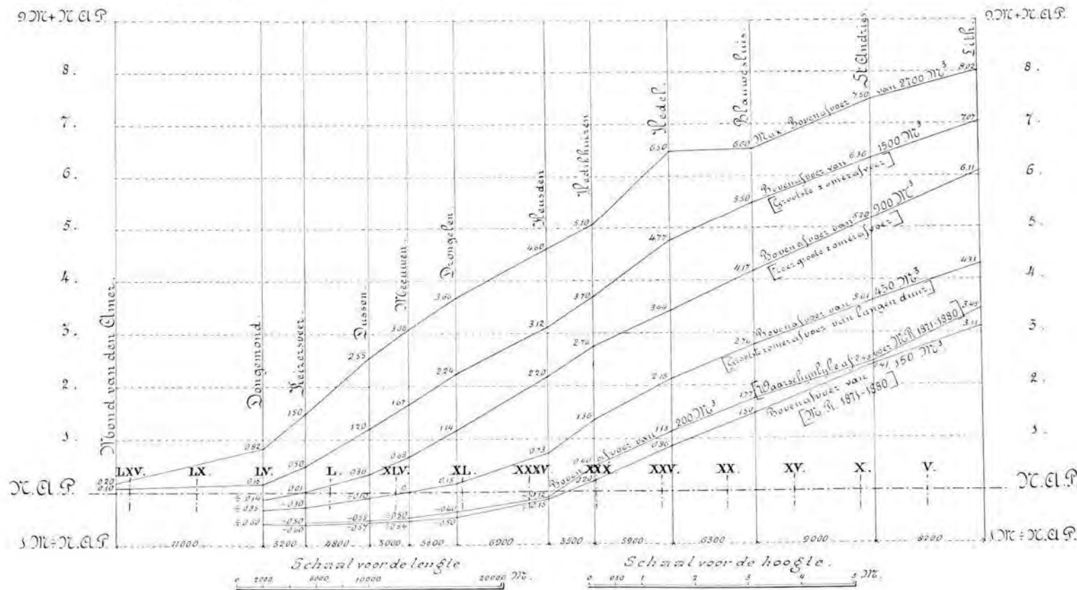
Fig. 84. Berekende verhanglijnen bij laagwater in den mond van den Amer.
