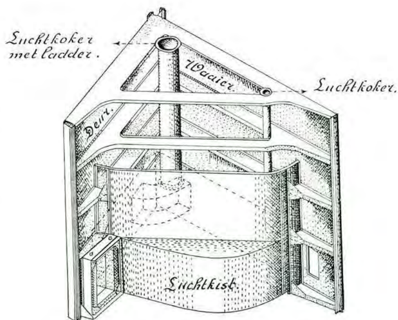
Fig. 69. De afsluitingswerken van de Maas bij Andel. Waaervlotdeur. Aanzicht.
