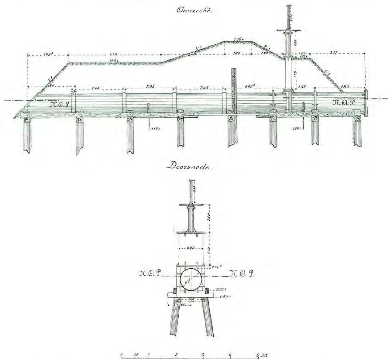
Fig. 34. Ijzeren duiker ten behoeve van het Waterschap „de Hooge en Lage Inlagen”.
