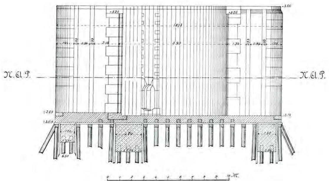
Fig. 66. De afsluitingswerken van de Maas bij Andel. Schutsluis: Maashoofd.
