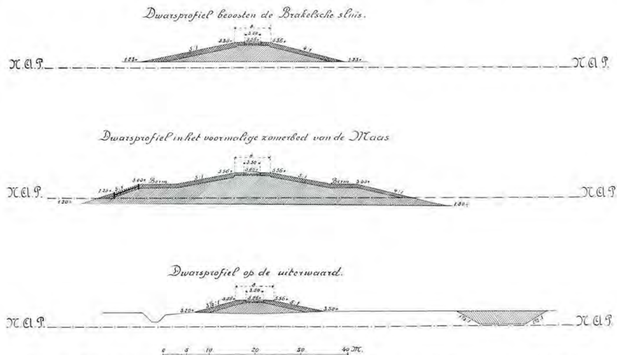
Fig. 72. De afsluitingswerken van de Maas bij Andel. Dwarsprofielen van den afsluitdijk.
