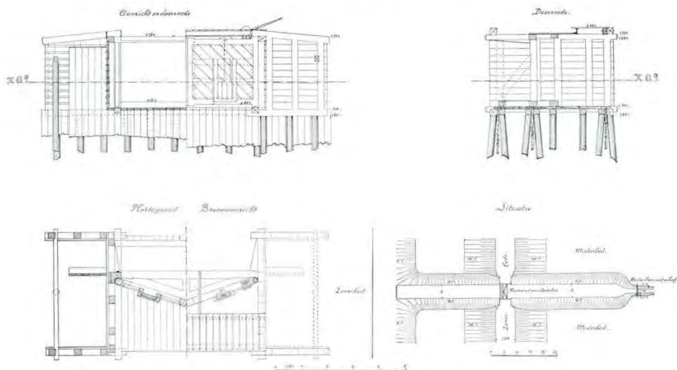
Fig. 5. Houten uit- en inlaatsluis met beer ten behoeve van het winterbed.
