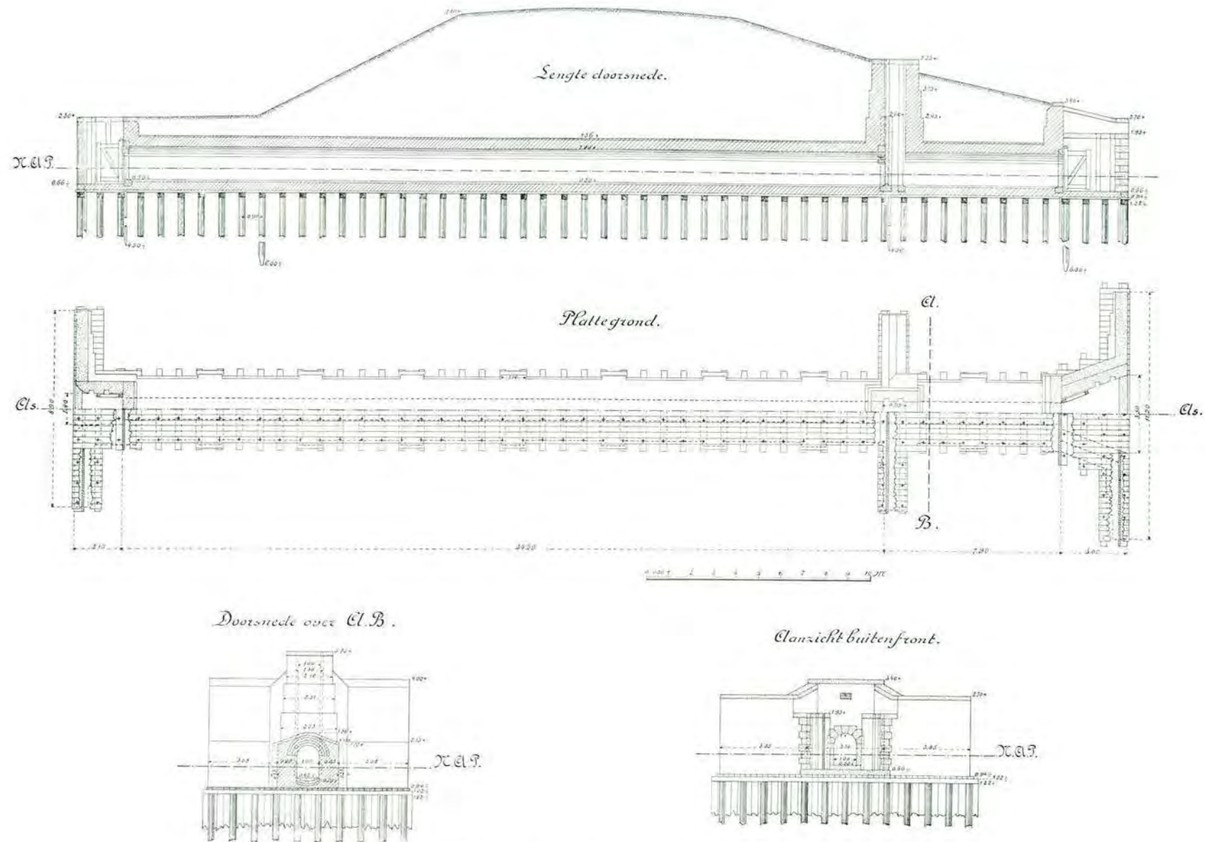
Fig. 58. Inlaatduiker bij Herpt.
