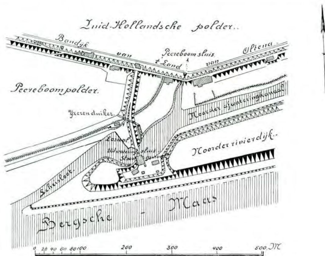
Fig. 36. Situatie van de afsluitings- en bemalingswerken aan den benedenmond van het noorderkanaal.
