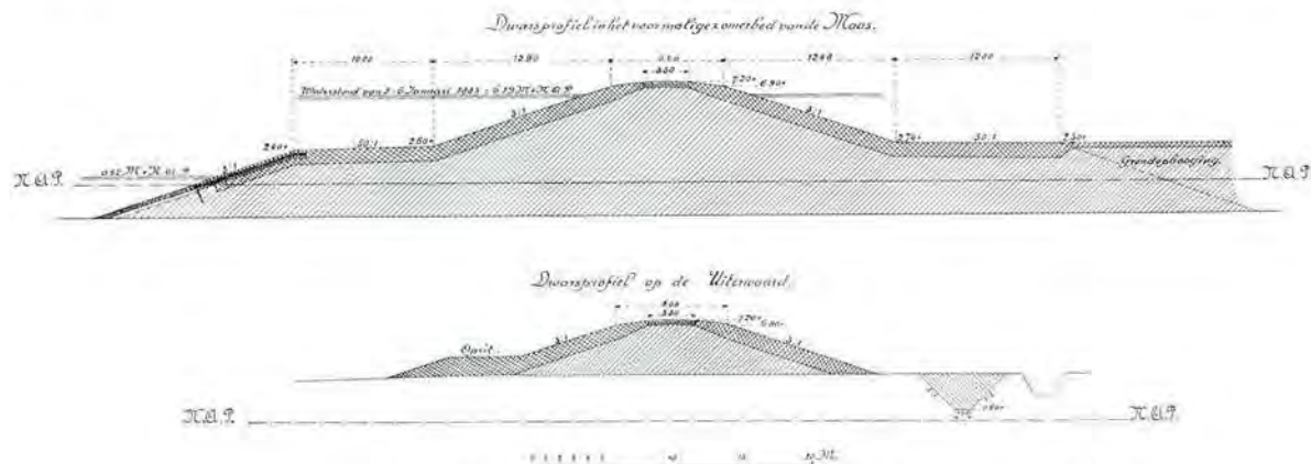
Fig. 74. De afsluitdijk van de Maas aan het Heleind. Dwarsprofielen.
