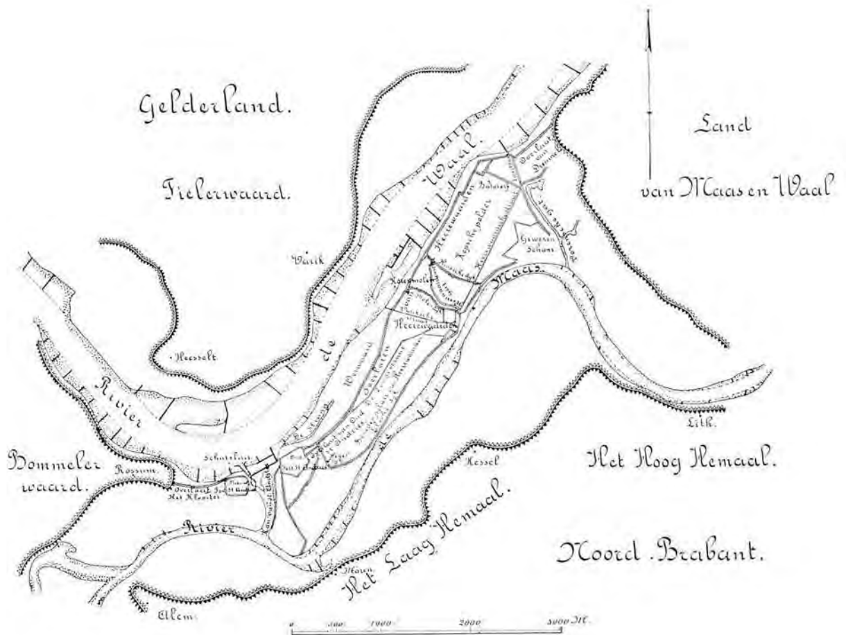
Fig. 62. De Heerewaardensche overlaten. Situatie in den voormaligen toestand.
