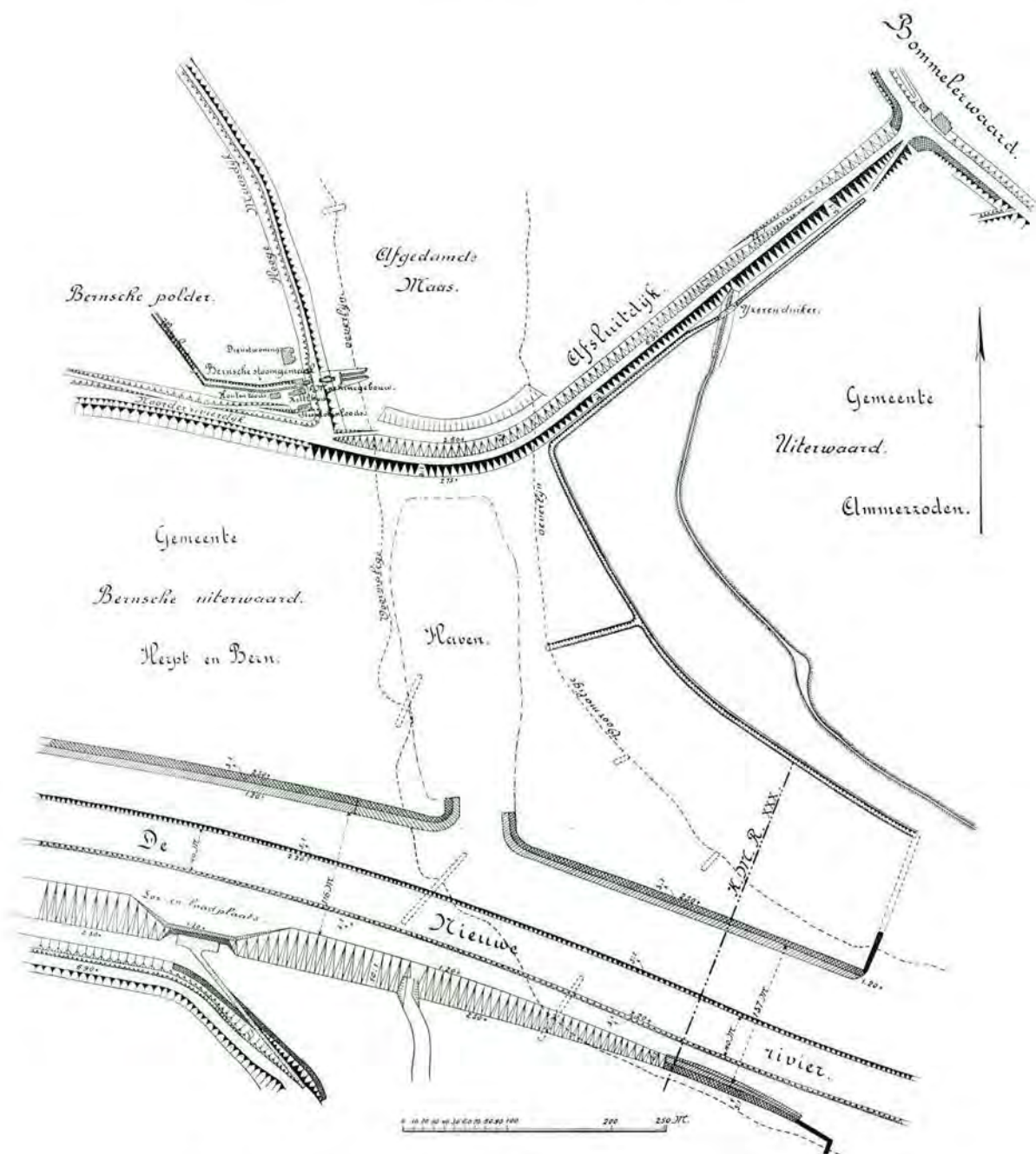
Fig. 73. De afsluitdijk van de Maas aan het Heleind. Situatie.
