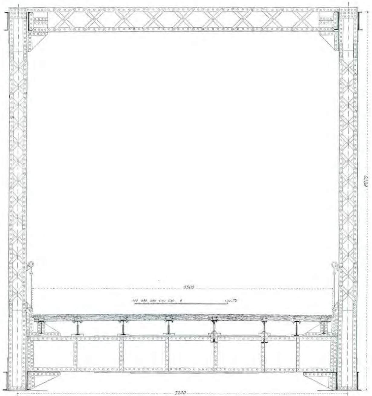
Fig. 27. Brug over het Heusdensch kanaal. Doorsnede over het midden eener vaste overspanning.
