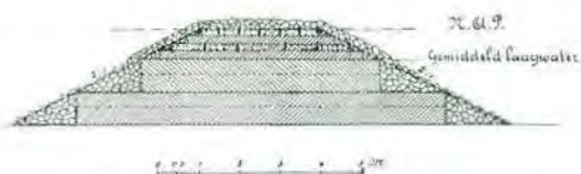
Fig. 11. Type van de rijzen dammen langs den Amer.
