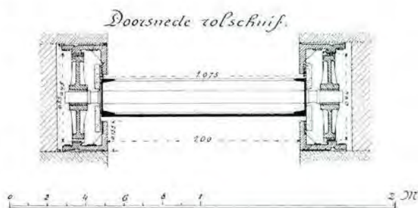
Fig. 67. De afsluitingswerken van de Maas bij Andel. Riolschuif.
