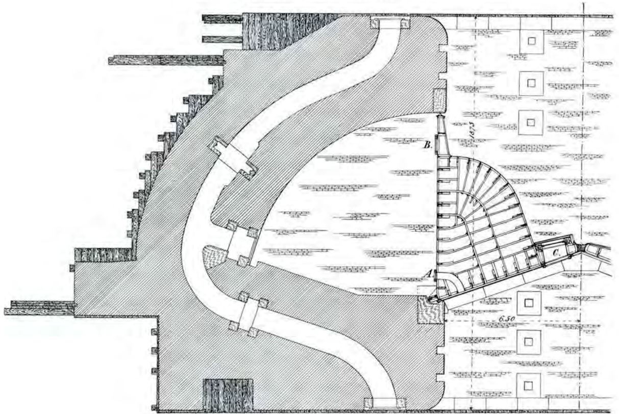
Horizontale doorsnede.
