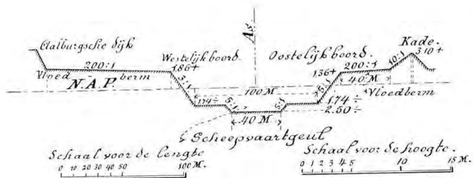
Fig. 12. Normaal dwarsprofiel van het Heusdensch kanaal.
