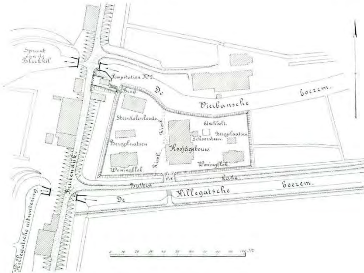
Fig. 54. Electricche bemaling op de Bleek- en Oostkil. Situatie van het centraalstation.
