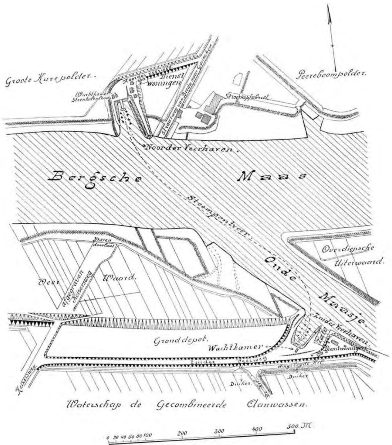
Fig. 18. Situatie van het Keizersveer.
