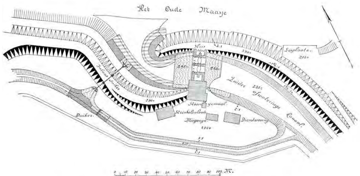
Fig. 47. Afsluitings- en bemalingswerken aan den benedenmond van het zuiderafwateringskanaal. Situatie.
