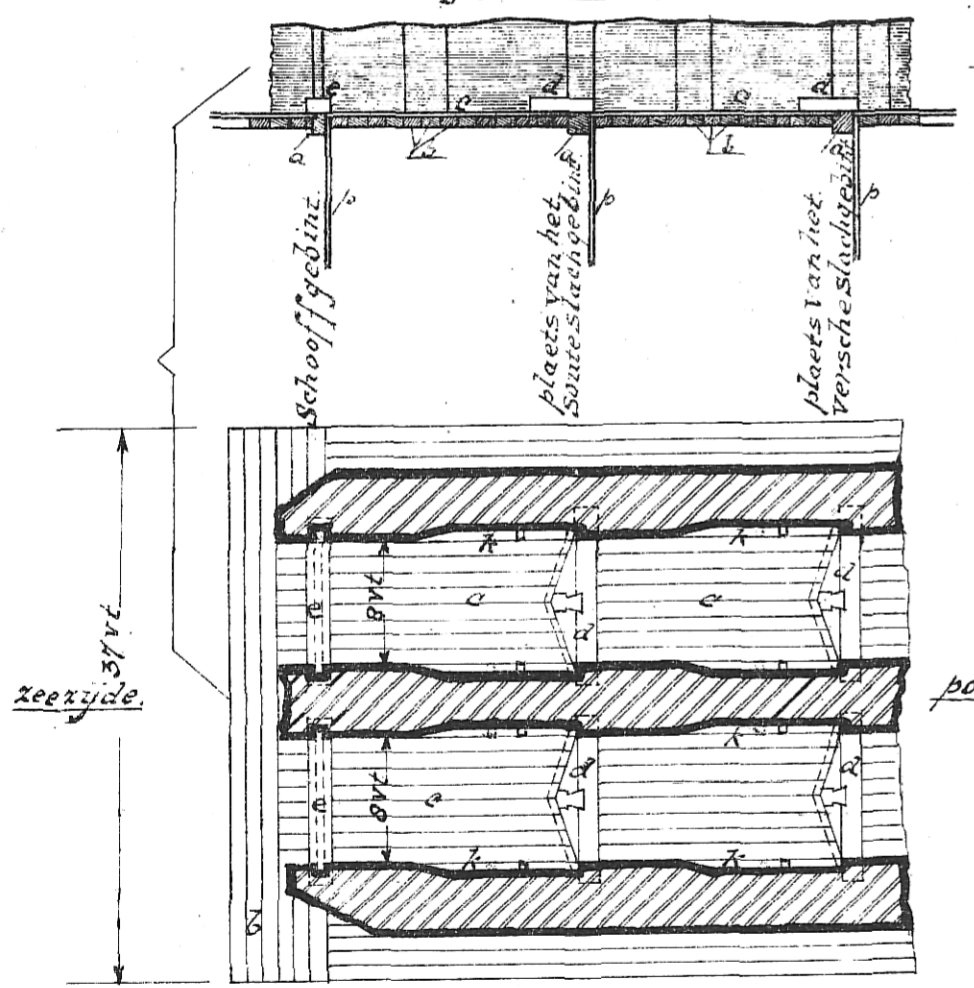
Ged. platte grond van een sluis.
