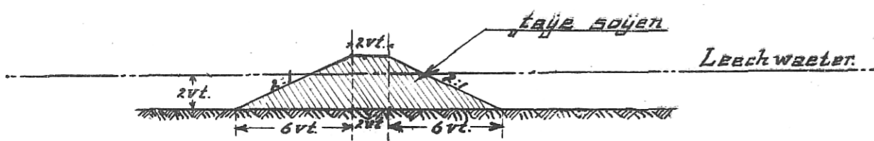
Dwaarsprofiel: duijkeldam.
