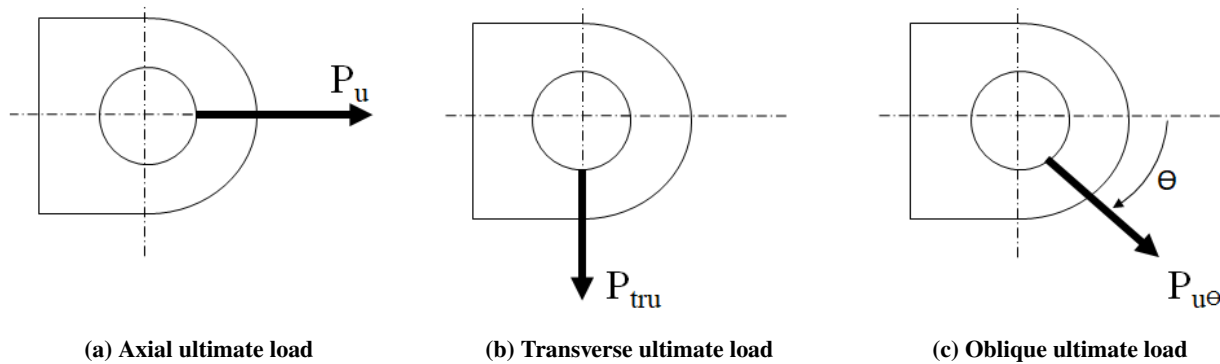
Fig. 7 Lug loading.
