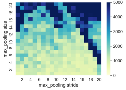
(d) T_{GE0} : tuning the last max-pooling layer (min: 638; max: >5 000)
