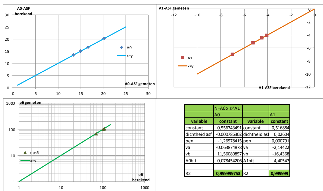
Figuur 14: Regressie relatie tussen de bitumen en asfalt vermoeiingslijn
