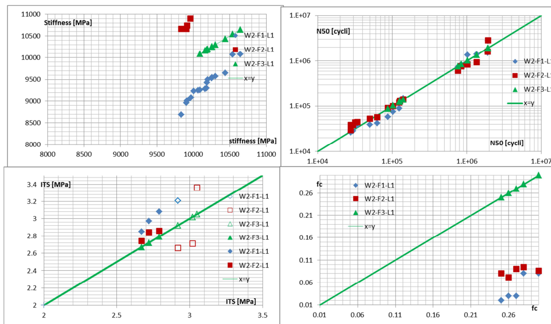
Figuur 9: Resultaten Werk 2, Lab 1 geplot per proef tegen de resultaten van F3
