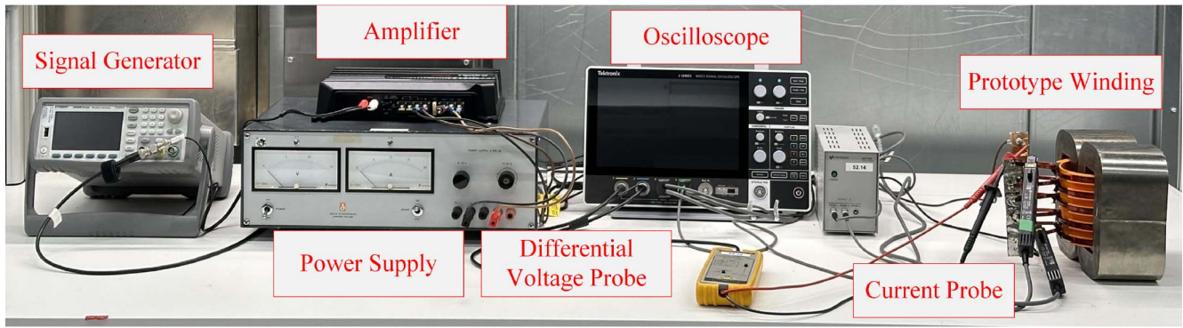
Fig. 11. Test table.
