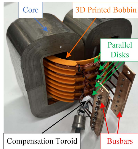
Fig. 12. Prototype.
