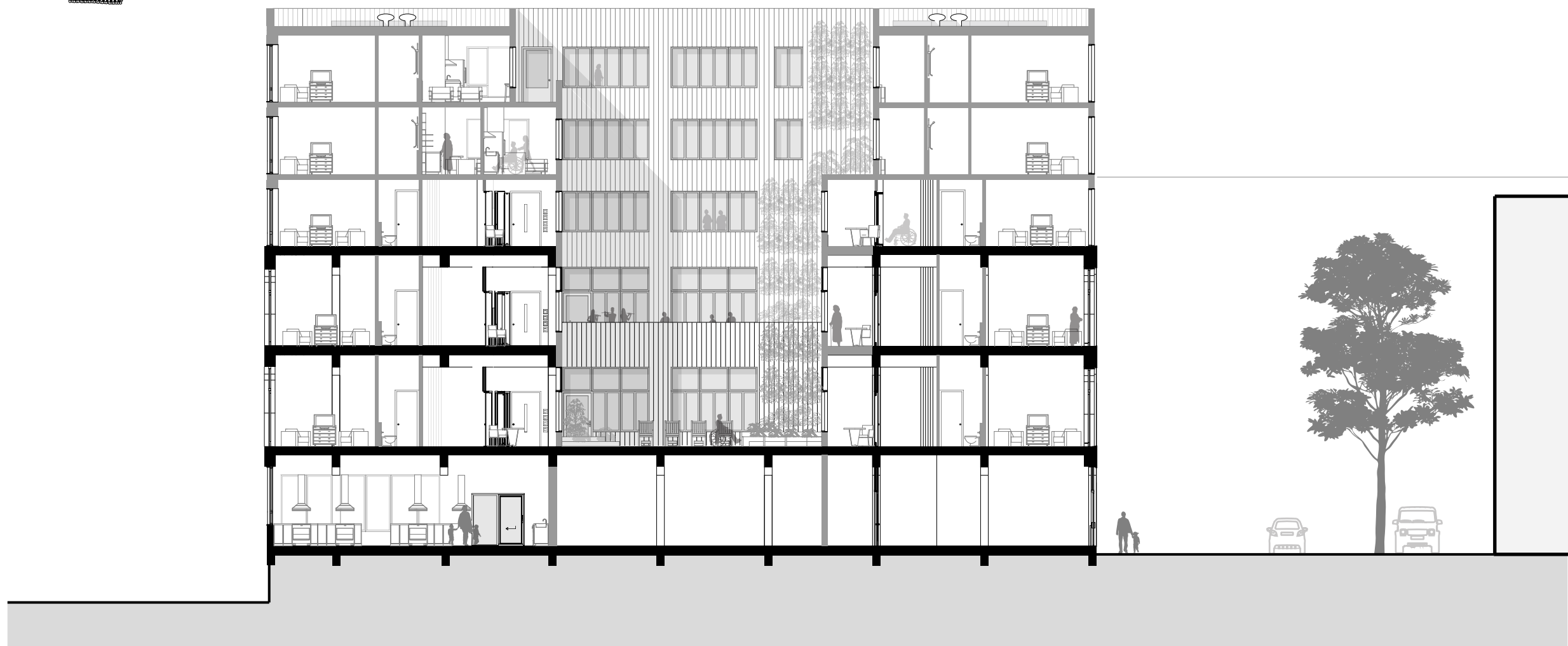
Section A-A 1:200
