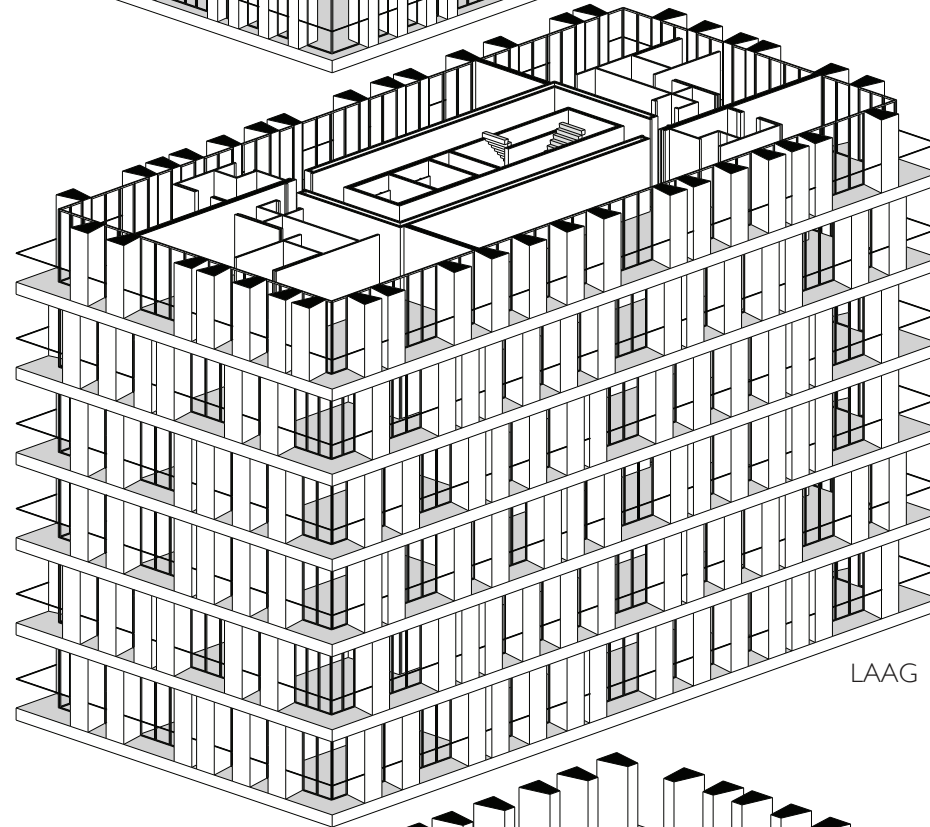
LAAG 2 WONINGEN
