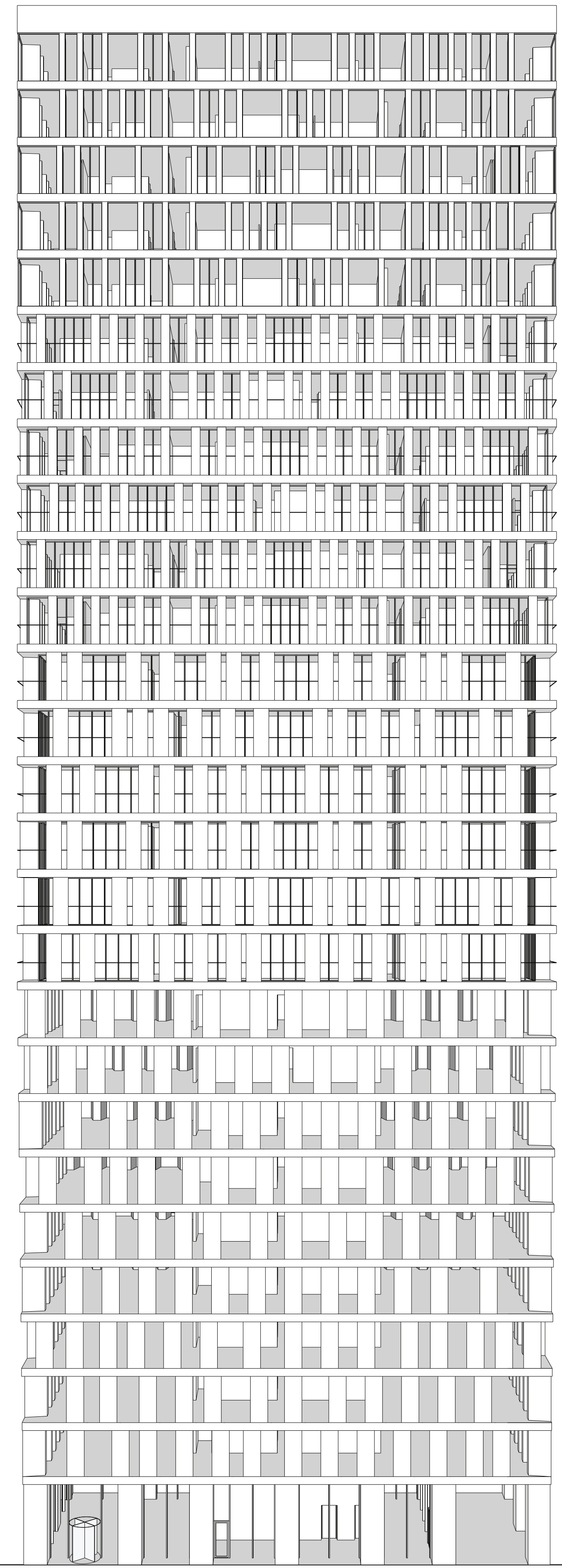
AANZICHT WESTGEVEL RICHTING RAVEL 1:200
