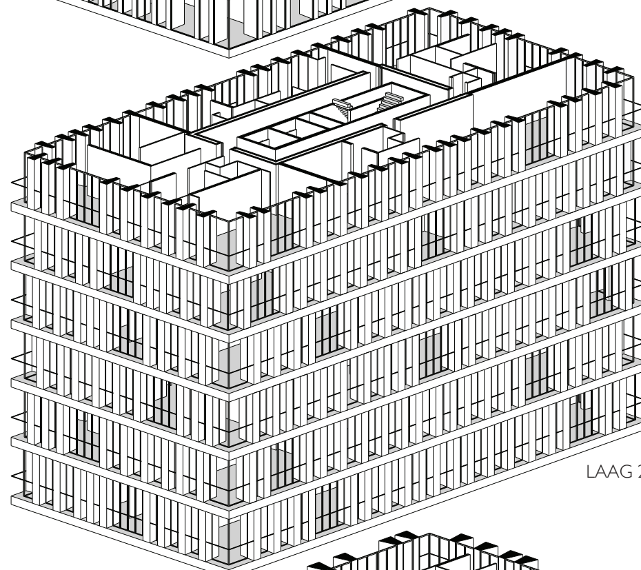
LAAG 3 WONINGEN
