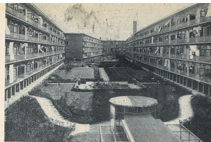
18. Particuliere woningbouw op Landlust. Binnenterrein Jan van Galenstraat. Architect J. Dunnebier 1934
