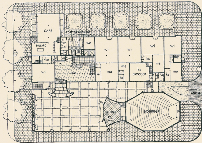
Hoogbouw A, begane grond 1 à 400
