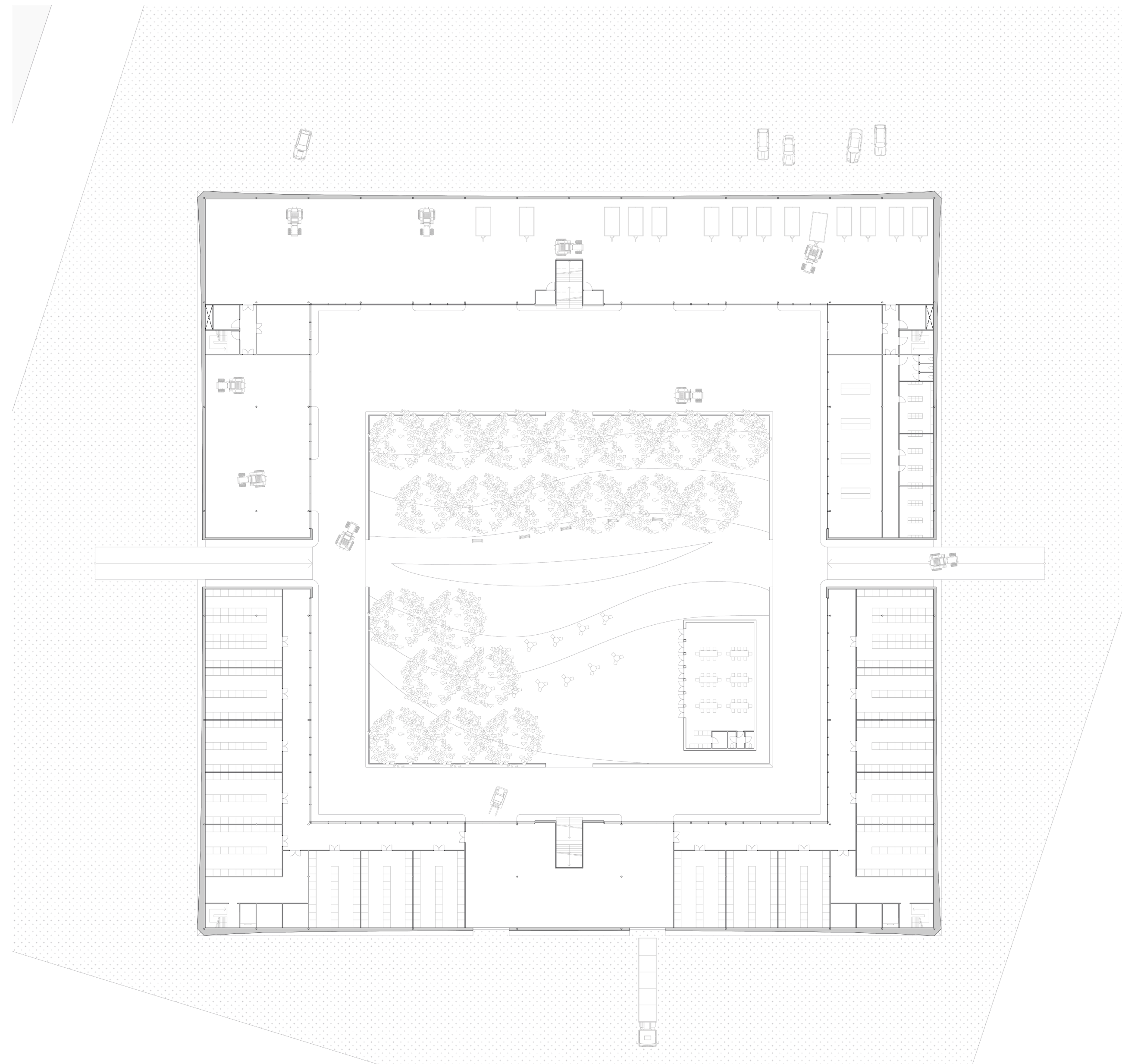
Plattegrond Hoofdgebouw Begane grond
