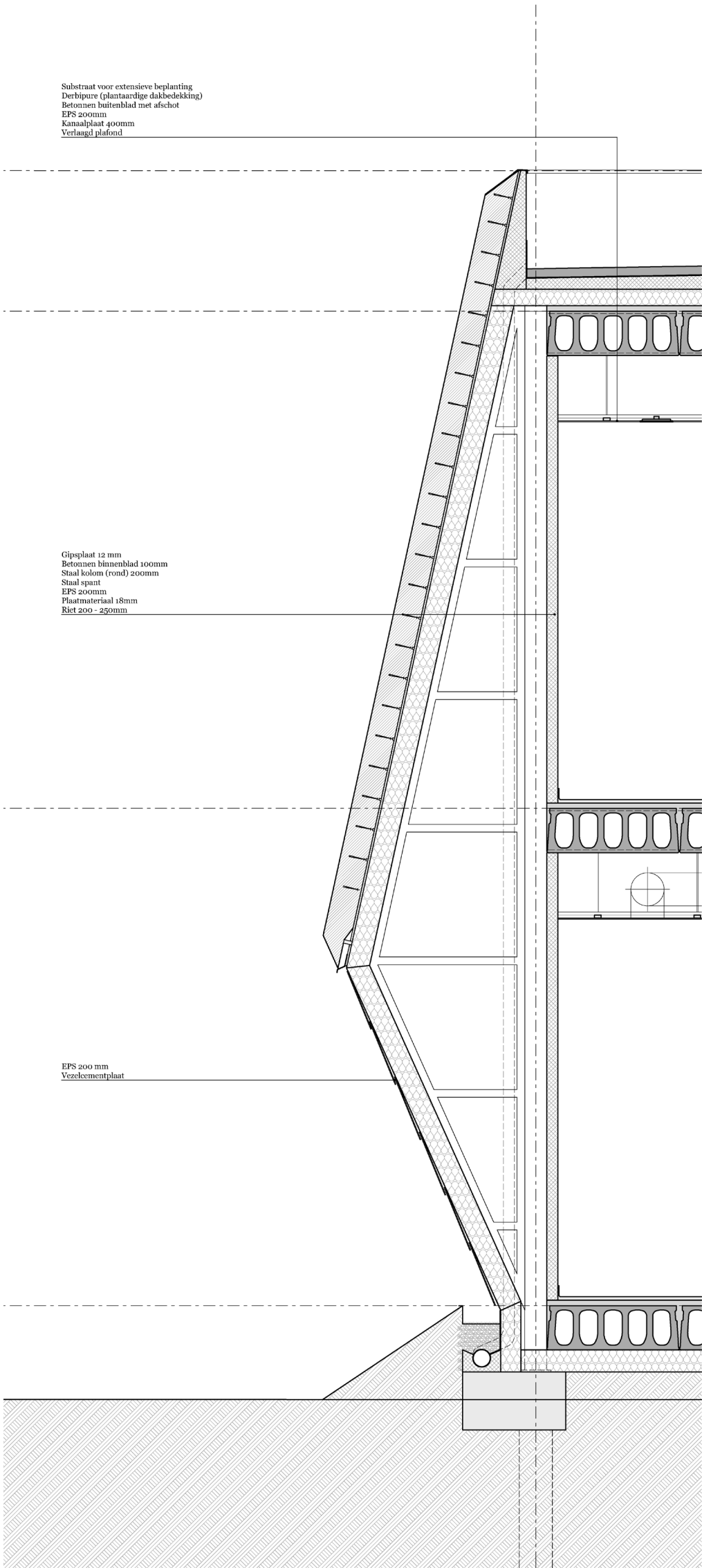
Buitengevel hoofdgebouw
