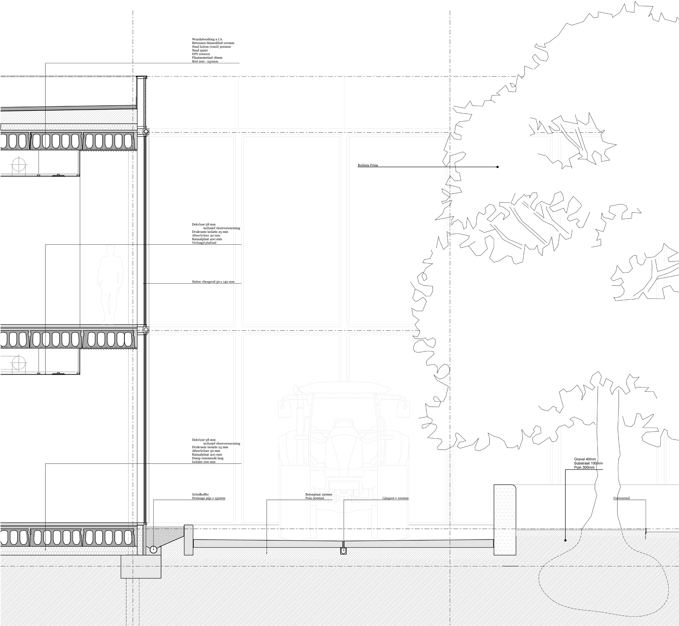
Doorsnede binnengevel en binnenplaats
