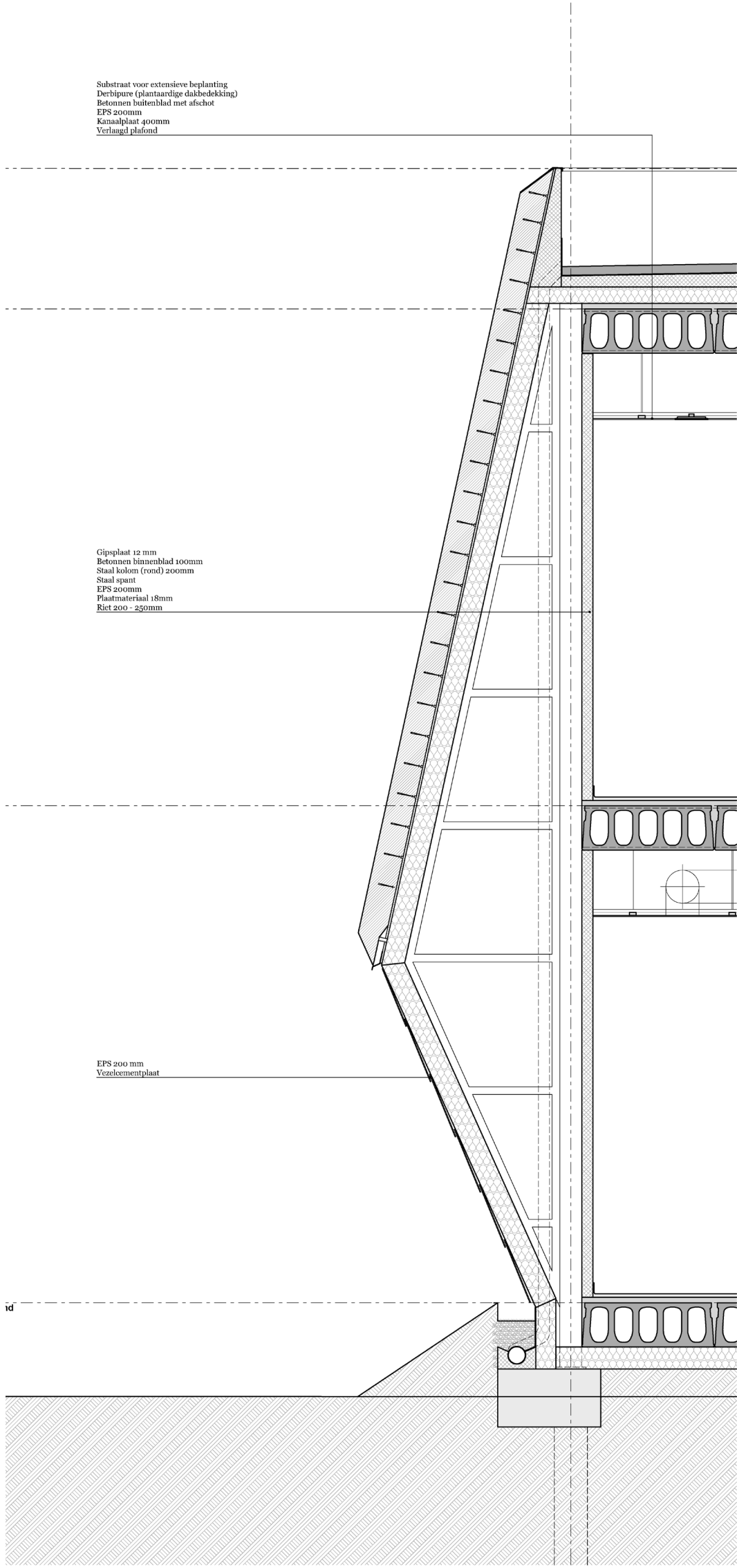
Buitengevel hoofdgebouw
