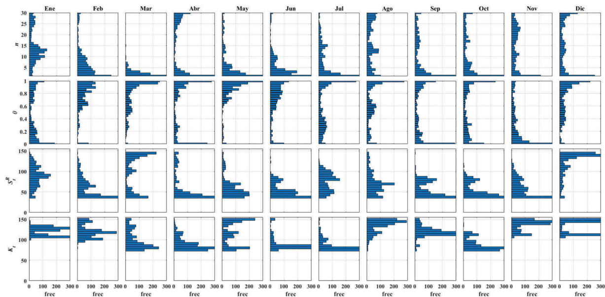
Figura 8. Histograma de parámetros obtenidos en el FP de OMC para el embalse Riogrande II con 3 criterios de escasez y 3 criterios de vertimiento de exceso. En cada fila se presentan los parámetros \theta , n , S_t^R y K_t . Las columnas representan cada mes del año.
