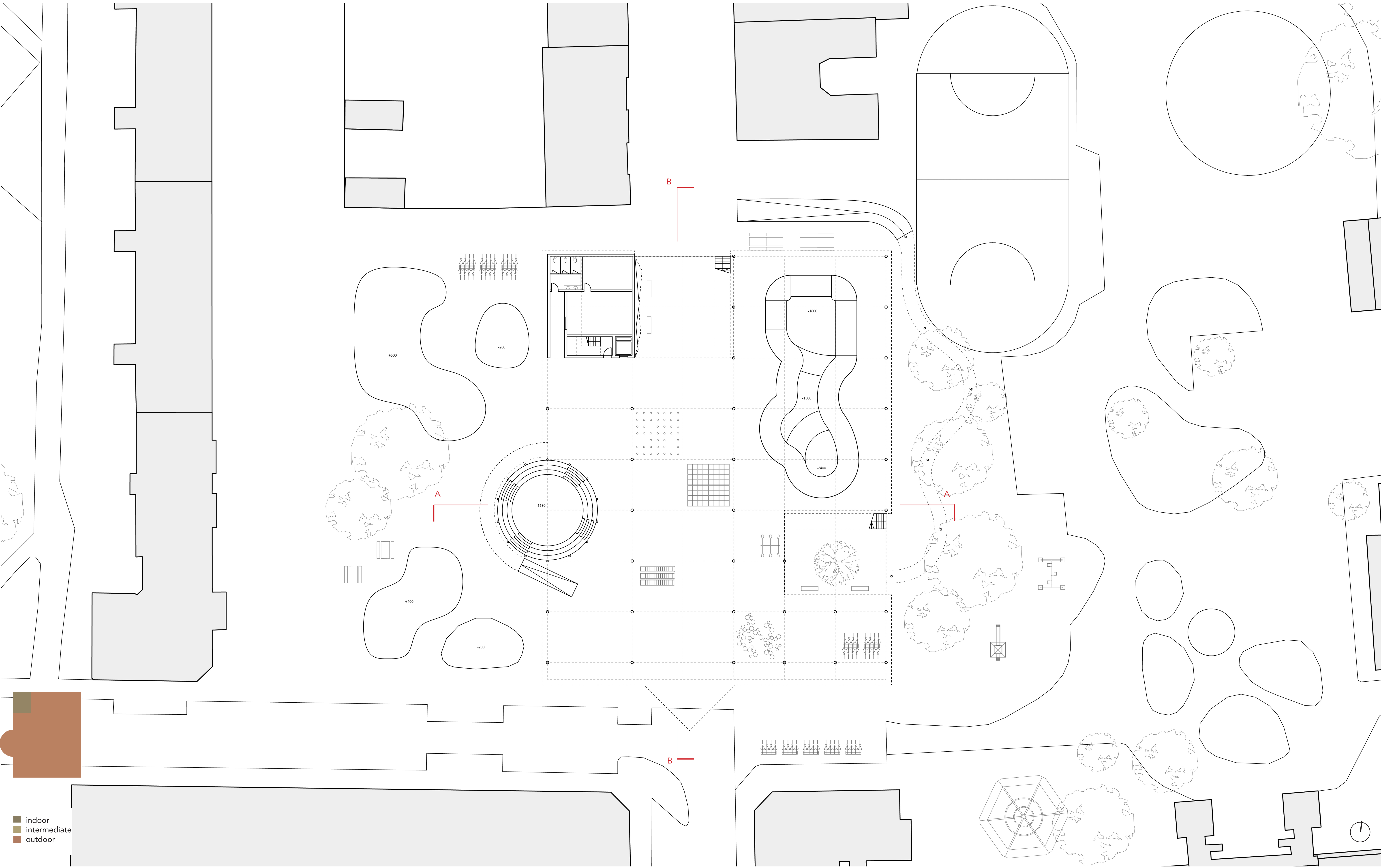
Plan G/F 1:200
