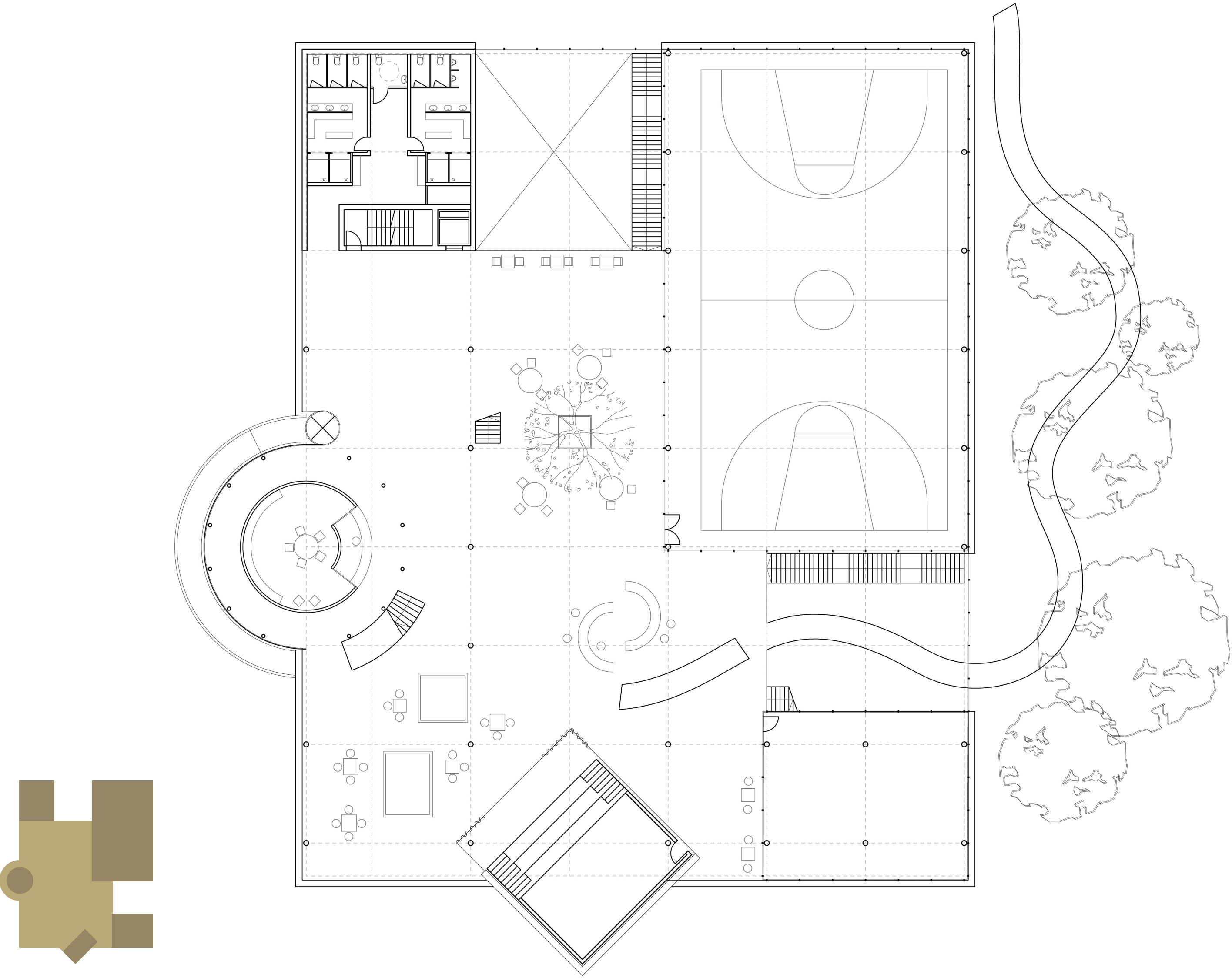
Plan 1/F 1:200
