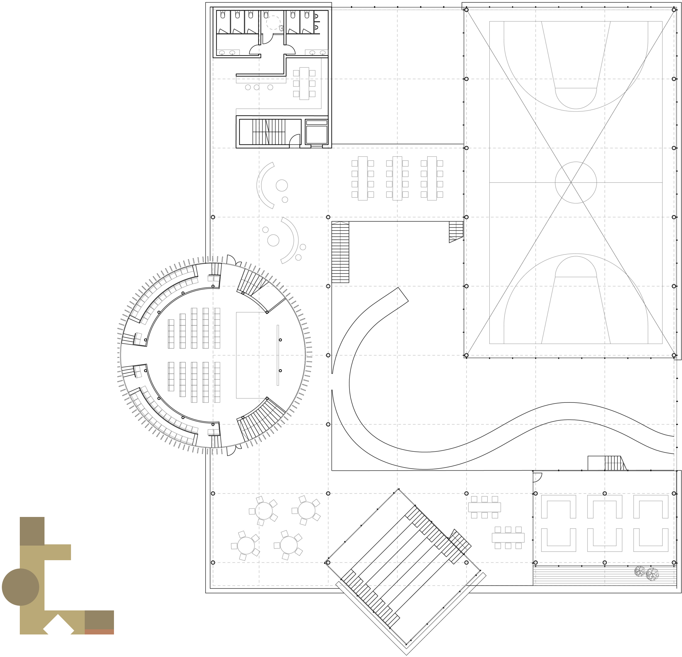
Plan 2/F 1:200
