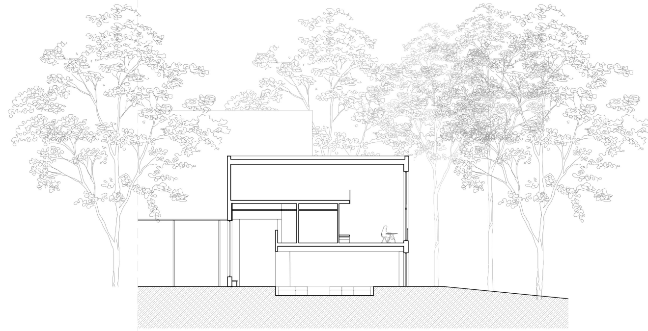
Section A-A
