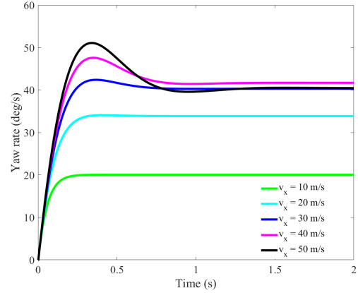
(d) Model response to varying velocity
