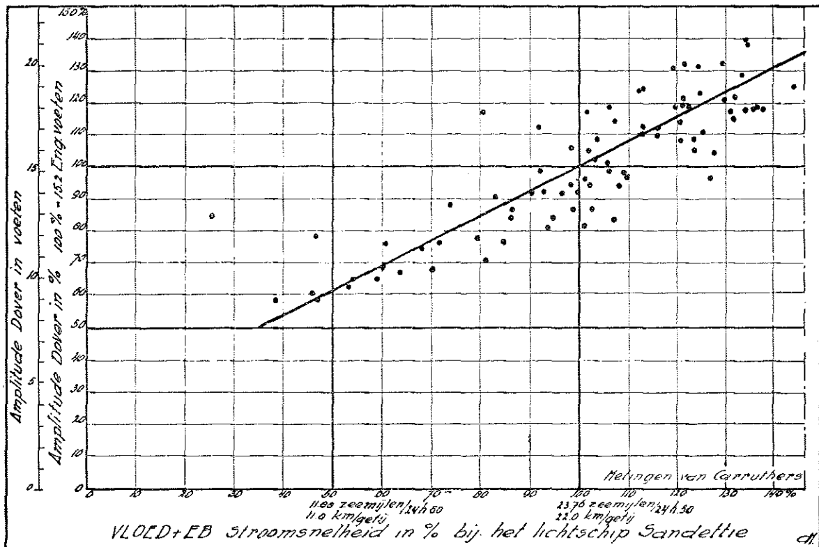
Fig. 22. Reductiegrafiek voor de stroomen bij het Sandettie lichtschip.
