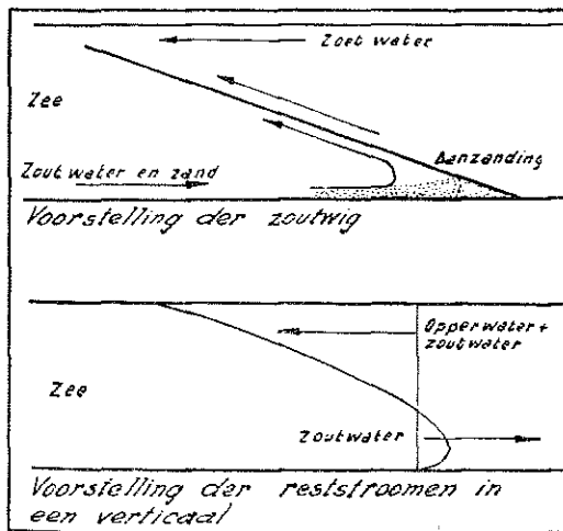
Fig. 4. Schematische voorstelling van de stroomingen veroorzaakt door verschillen in soortelijk gewicht in riviermonden.
