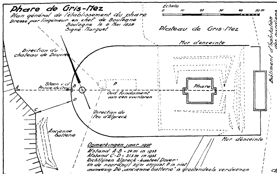
Fig. 52. Situatie van de vuurtoren van Gris Nez in 1838.
