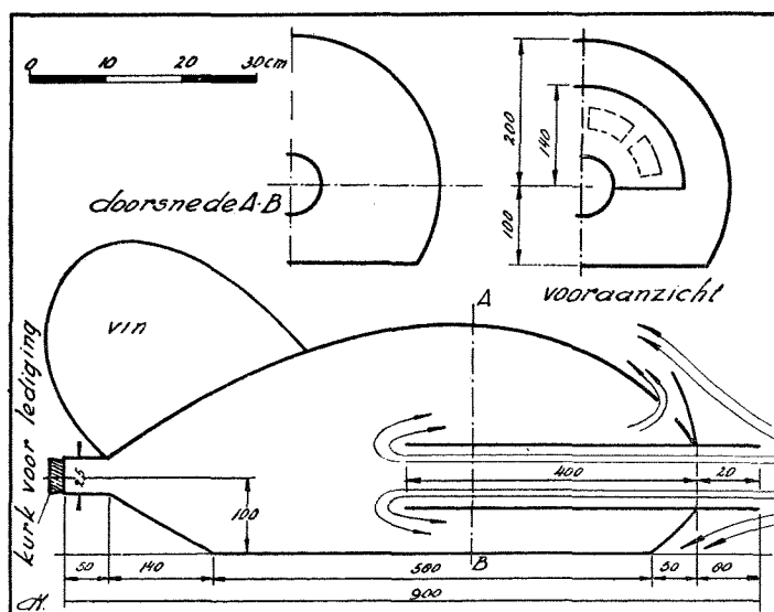
Fig. 131. Zandvanger van CANTER CREMERS.
