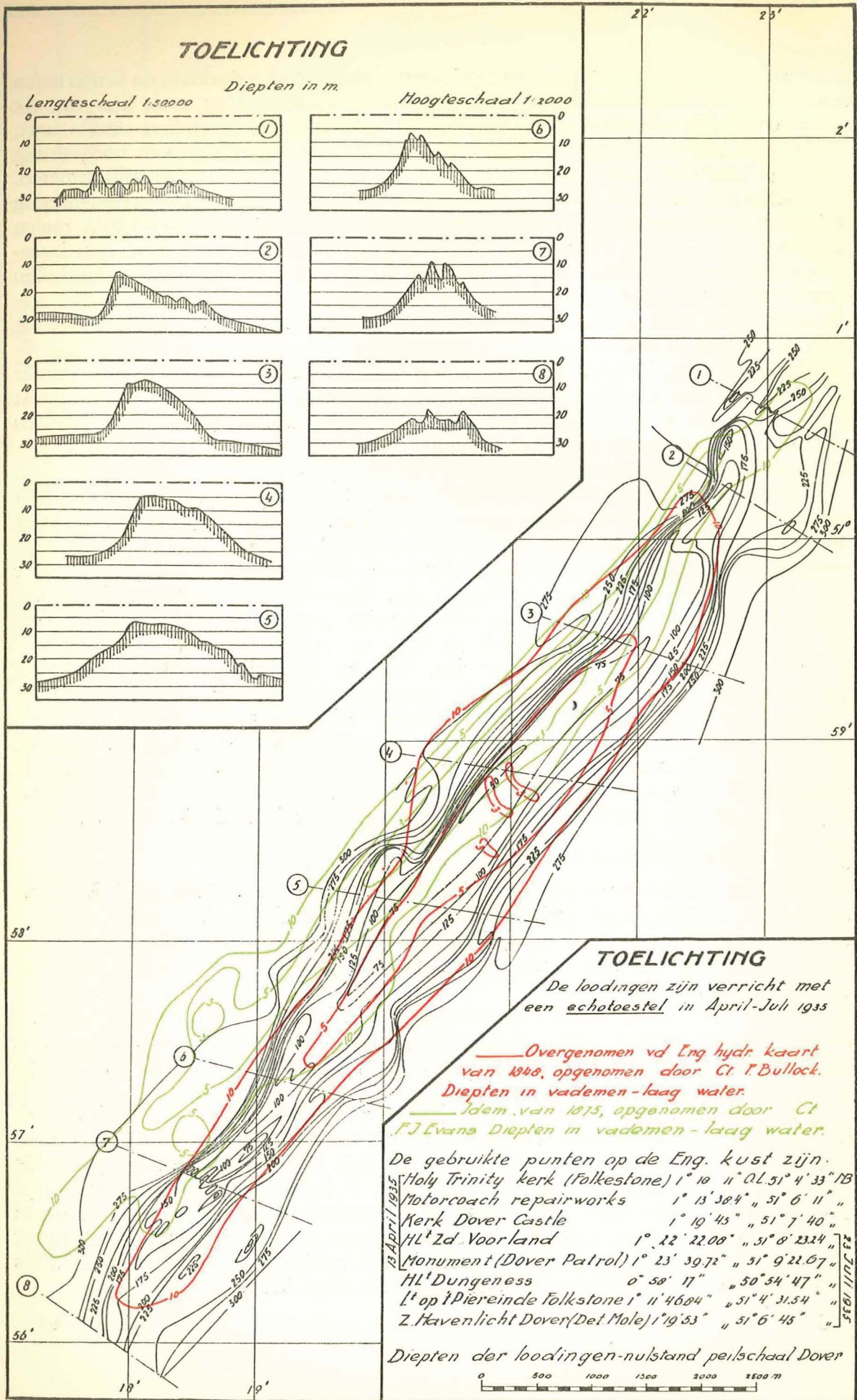
Fig. 41. Looding van de Varne in 1935, vergeleken met die van 1848 en 1875.
