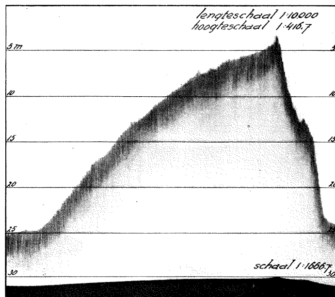
Fig. 71. Dwarsprofiel van de Varne.
