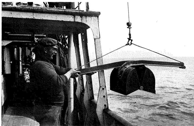
Fig. 136. Grijper, geopende stand.
