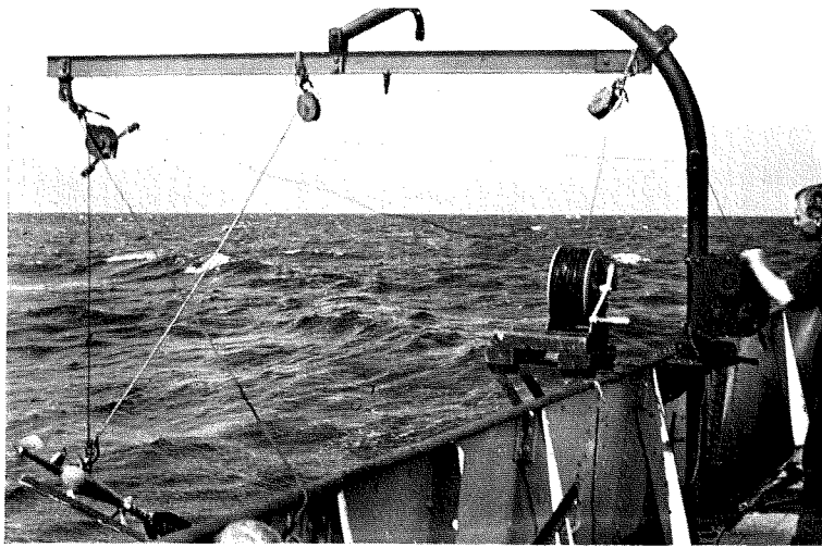
Fig. 129. Davit voor den OTT-stroommeter.
