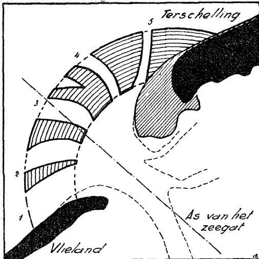
Fig. 98. Schema van de geulen eener buitendelta. (Zeegat van het Vlie.)
