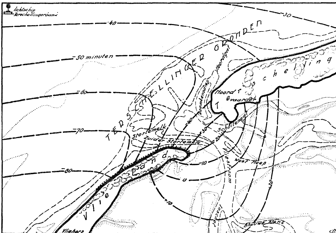
Fig. 100. Voorbeeld van de ligging der tijdlijnen voor het M 2 -getij bij het zeegat van het Vlie. (Verschillen van de x-getallen ten opzichte van West-Terschelling.)
