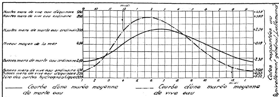
Fig. 39. Getijgegevens van Boulogne.
