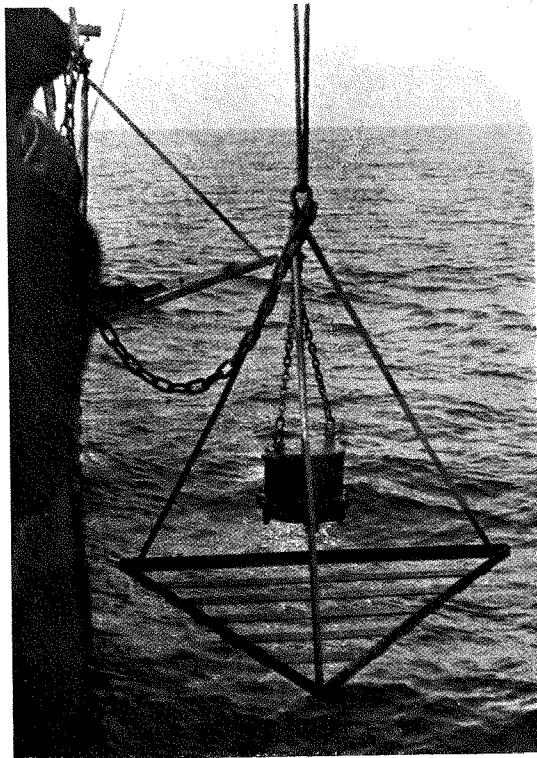
Fig. 127. Ophanging van een DE VRIES-meter.
