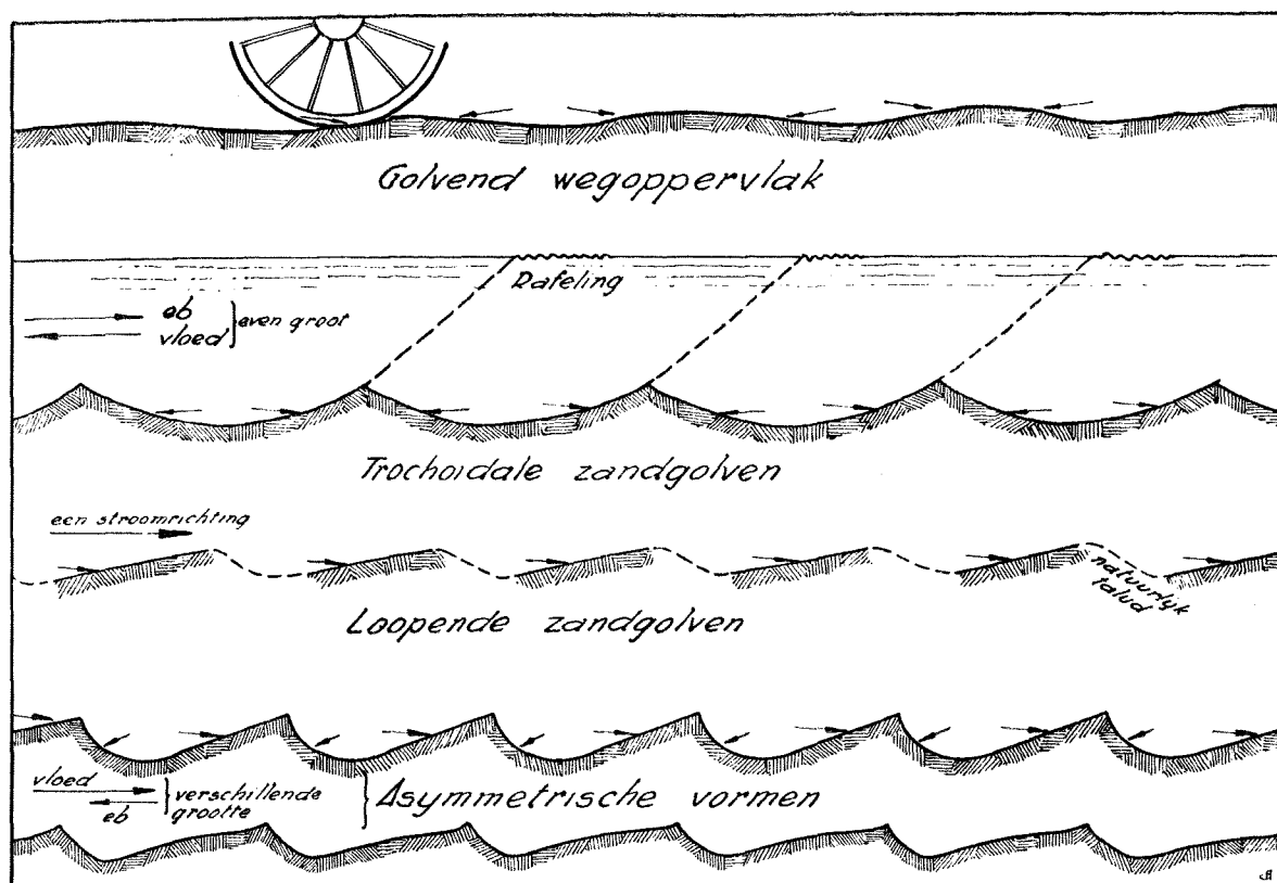
Fig. 74. Golfvormen (voldoende zand).
