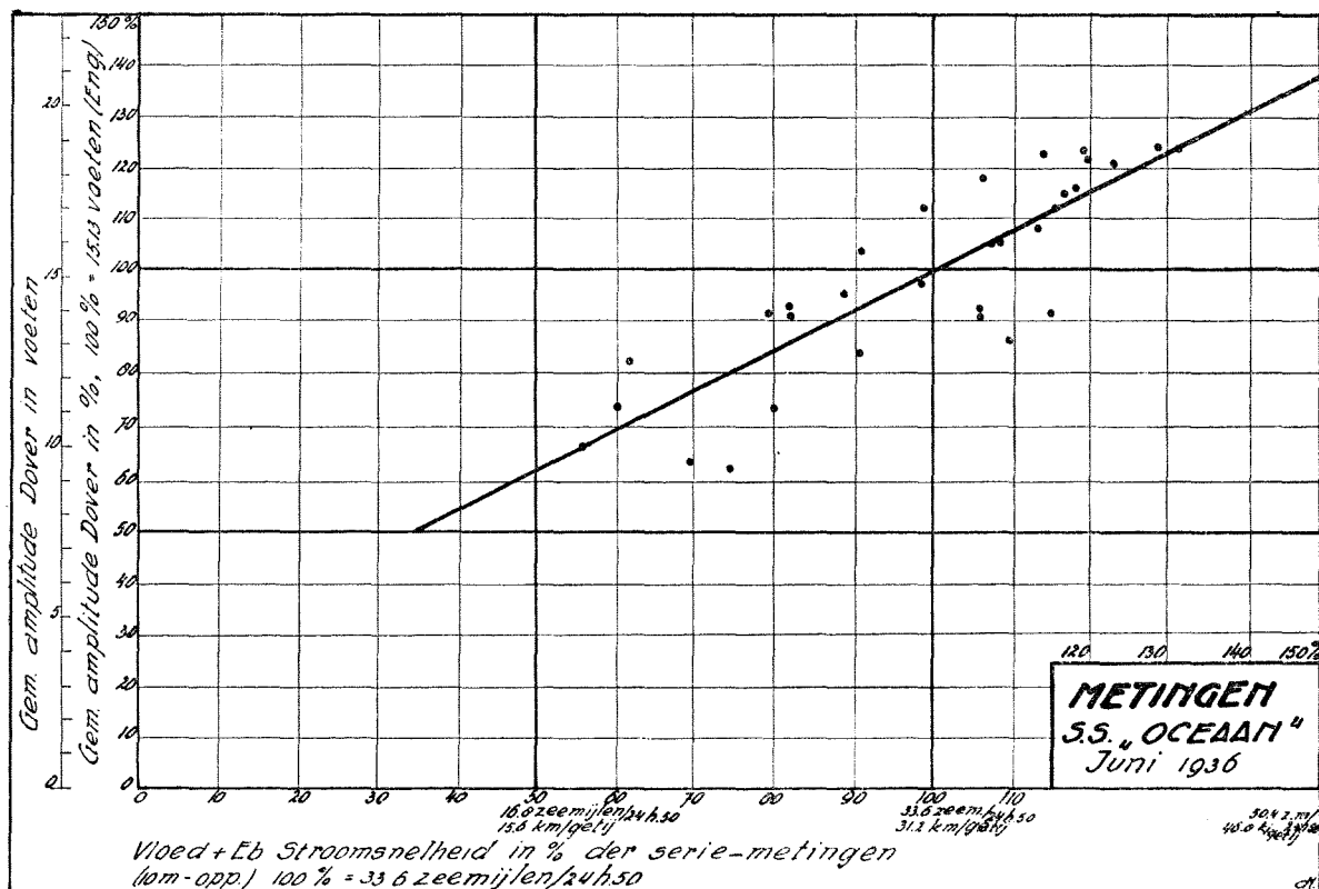
Fig. 145. Reductiegrafiek volgens 16 daagsche meting door de „Oceaan“ in 1936.
