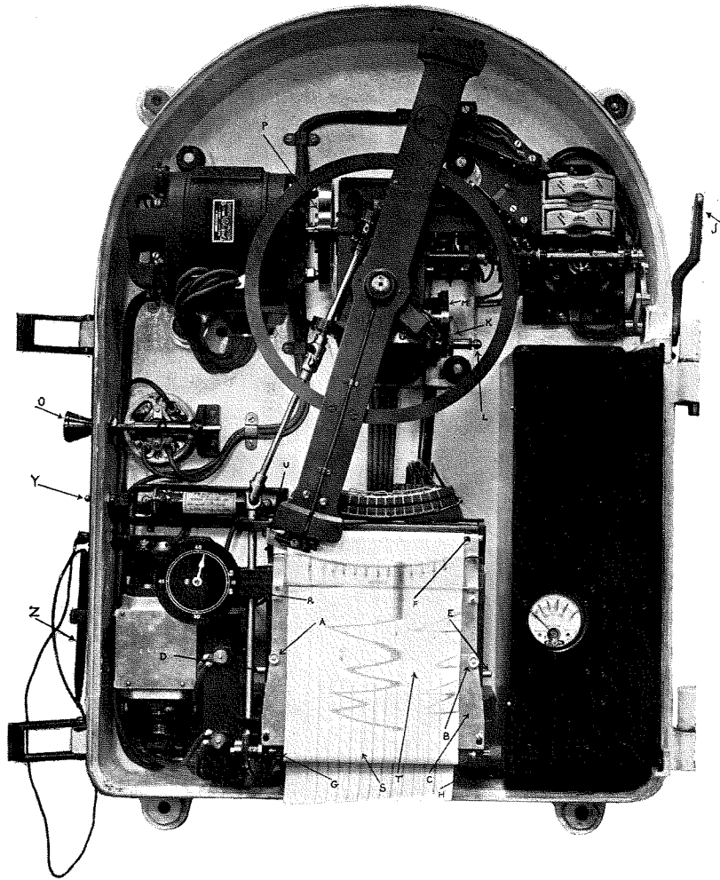
Fig. 124. Echotoestel voor ondiep water (Rijkswaterstaatsmodel, diepteschaal 1 : 400 en 1 : 100).
