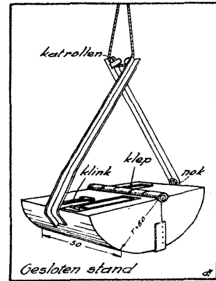
Fig. 135. Gripper (eigen ontwerp).
