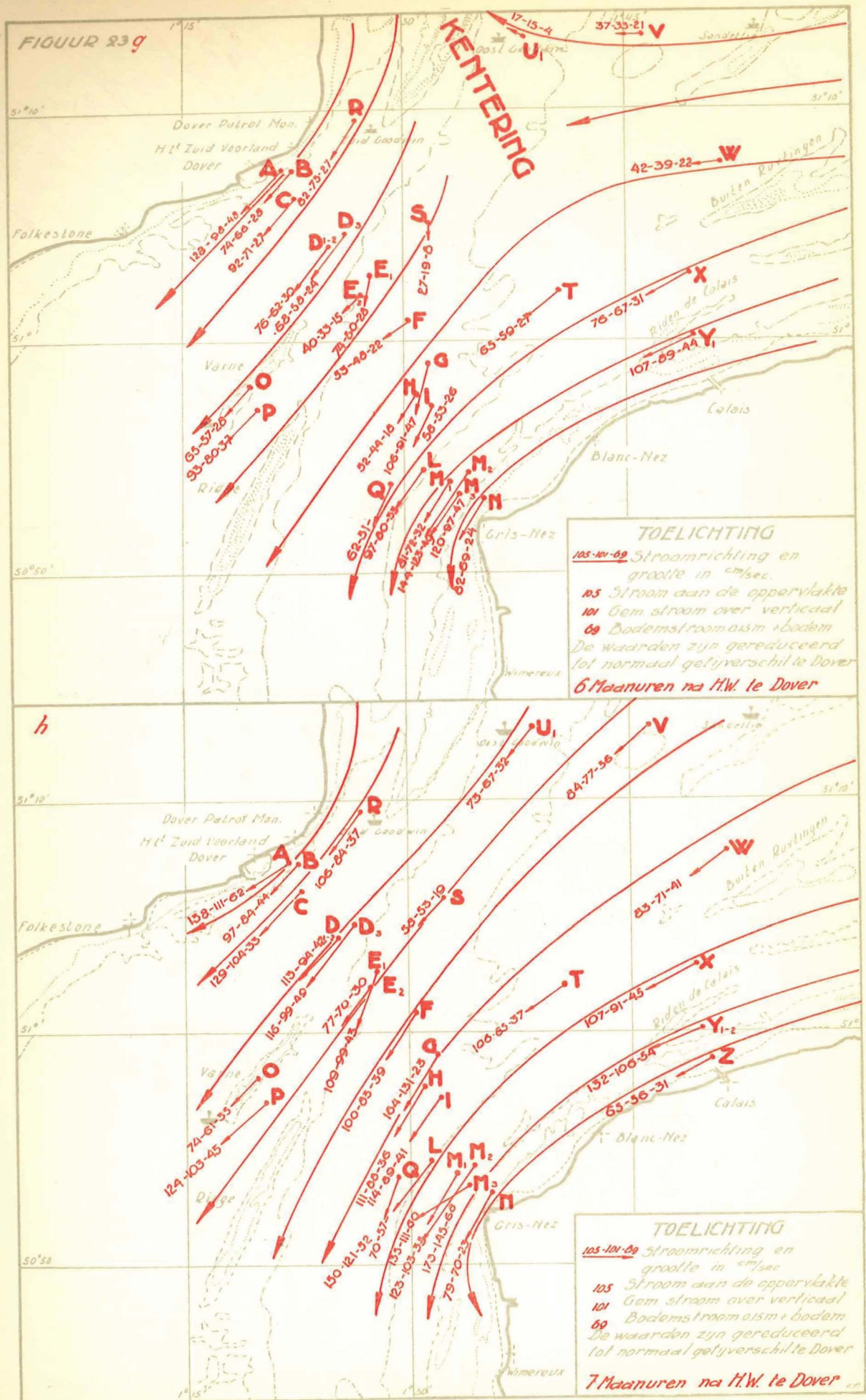
Fig. 23g en h. De twaalf-urenkaartjes van de normale stroomen in de Hoofden.
