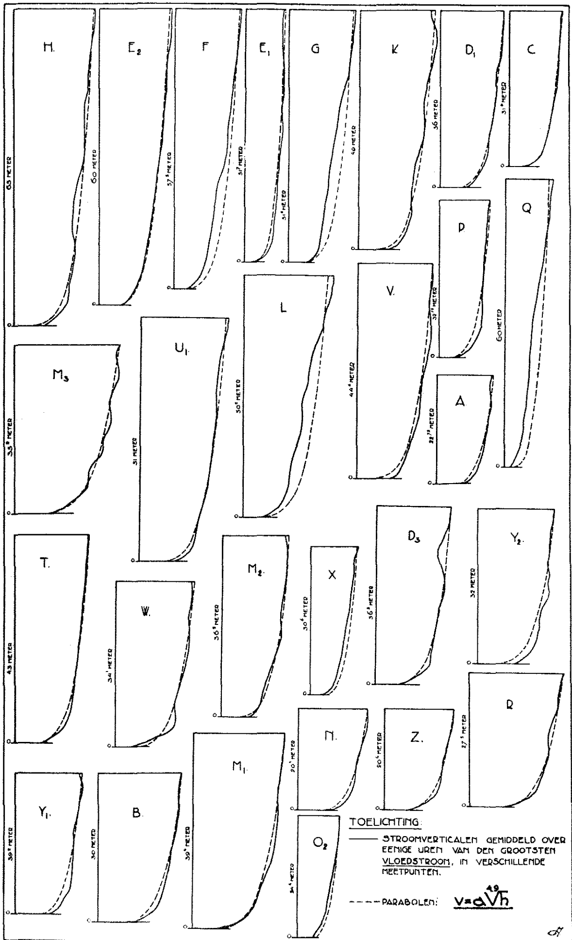
Fig. 15. Gemiddelde stroomverticaalen in de Hoofden bij vloedstroom. Snelheidsschaal 1 cm = 0.60 m/sec.
