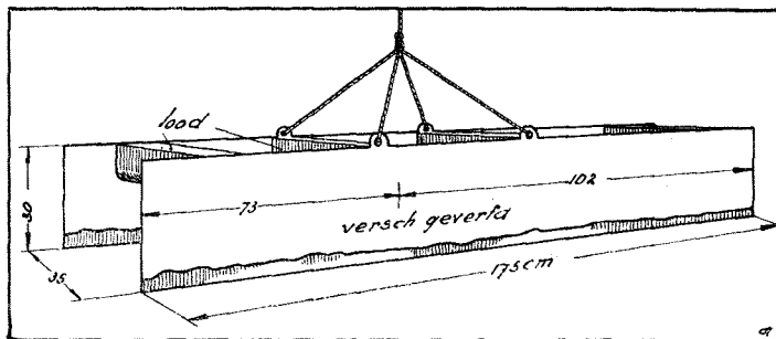
Fig. 142. Ribbelmeter.
