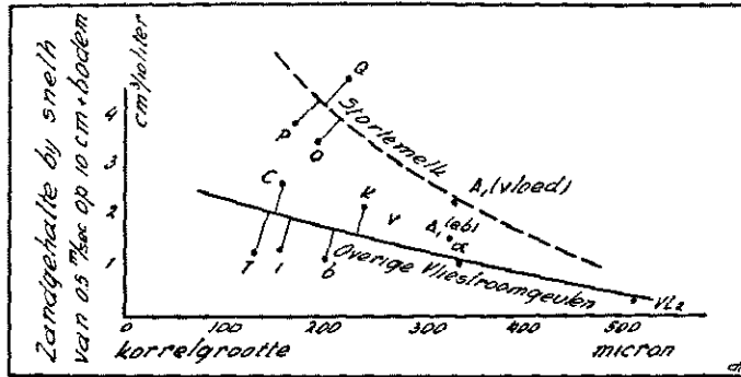
Fig. 18. Verband tusschen korrelgrootte en zandgehalte bij een snelheid van \frac{1}{2} m/sec. op 10 cm. boven den bodem.
