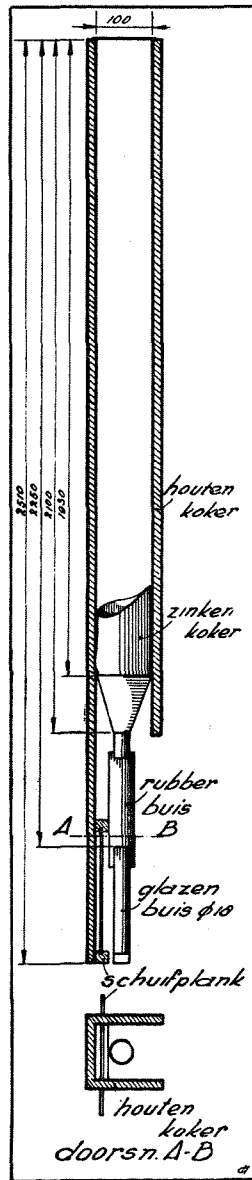
Fig. 138. Bezinkingsmeter (eigen ontwerp).
