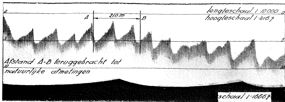
Loopende zandgolven op de Baas; noordzijden steil.
