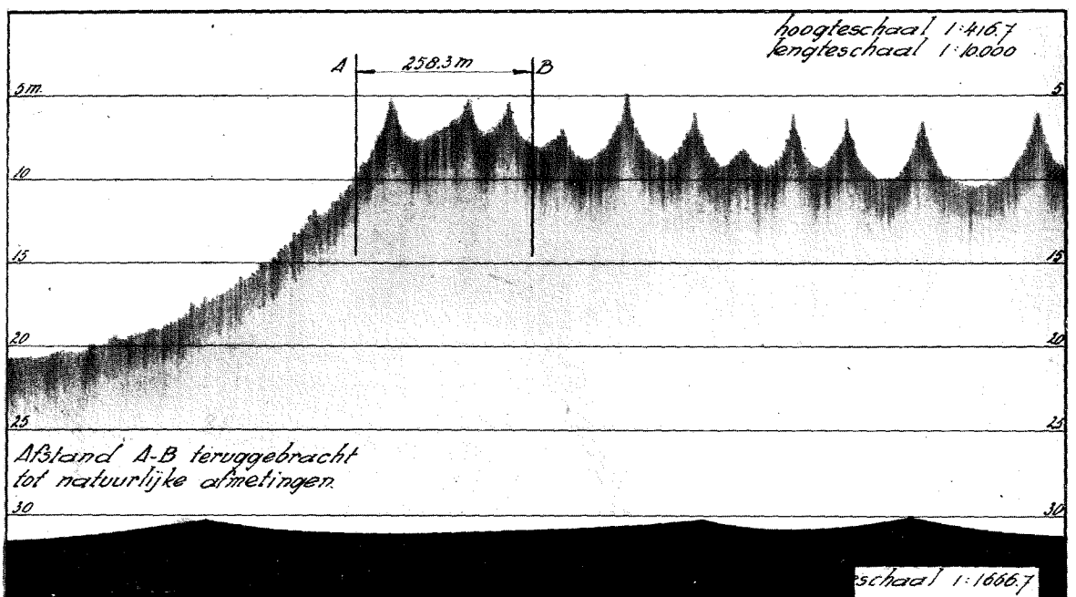
Fig. 78. Dwarsprofiel van de Rabsbank.
