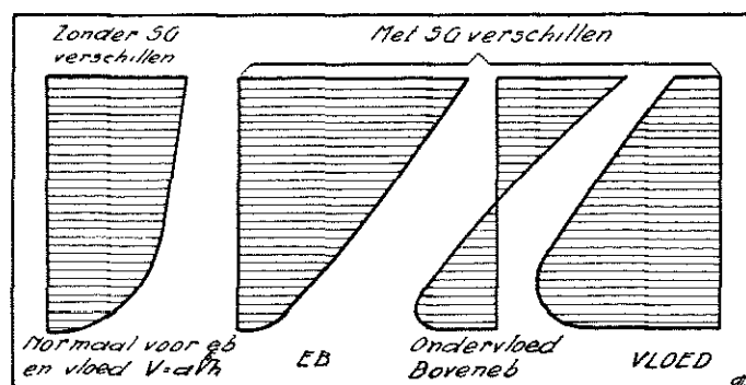
Fig. 13. Voorbeelden van normale en gestoorde stroomverticalen.
