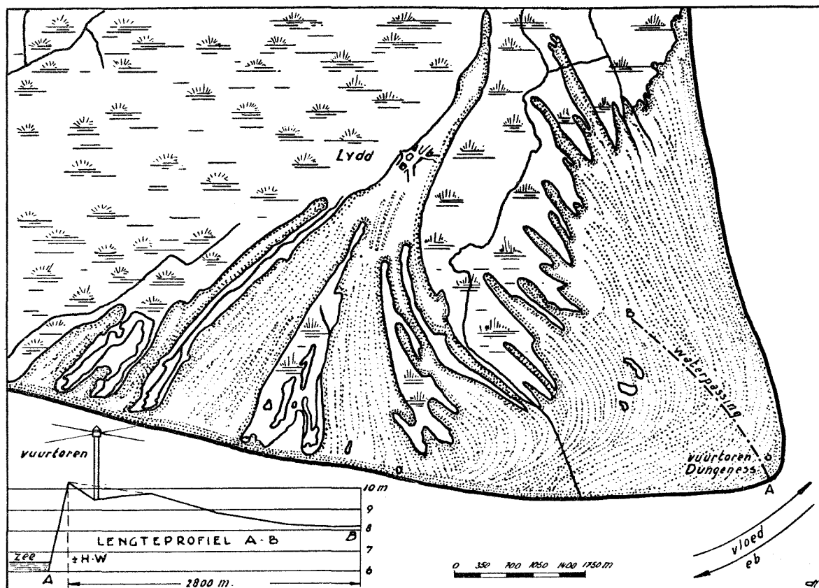
Fig. 93. De grindruggen op Dungeness (naar JOHNSON en een foto van de Royal Air Force).
