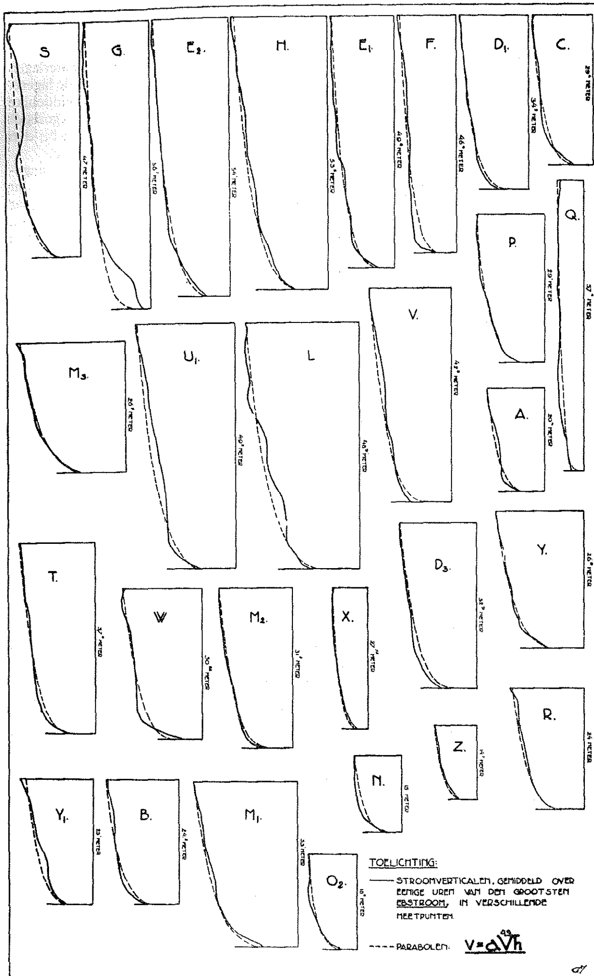
Fig. 16. Gemiddelde stroomverticaLEN in de Hoofden bij ebstroom. Snelheidsschaal 1 cm = 0.60 m/sec.
