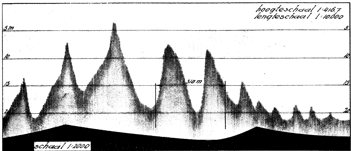
Fig. 70. Dwarsprofiel over de zuidpunt van de Falls.
