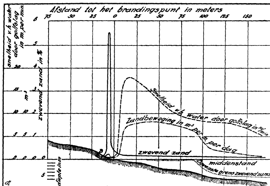
Fig. 88. Zandtransport en snelheden in de brandingsstrook volgens de „Beach Erosion Board”.
