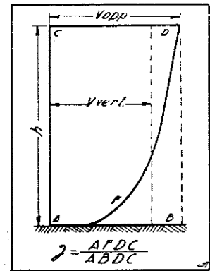
Fig. 14. Benaderende parabool v = a \sqrt[q]{h} voor de stroomverticalen.
