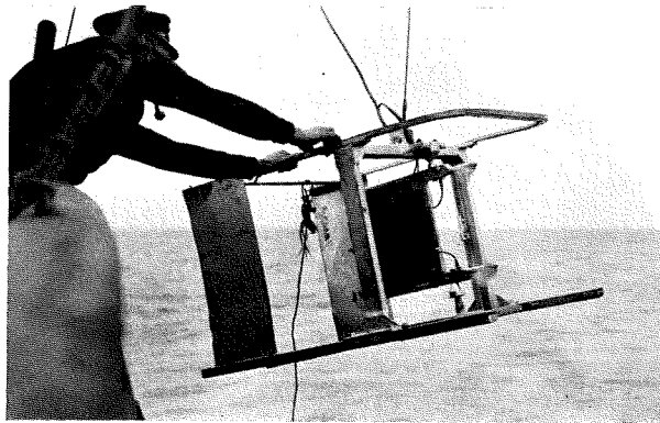
Fig. 130. Bodemstroommeter voor stroomen op 0,15 en 0,50 m + bodem.
