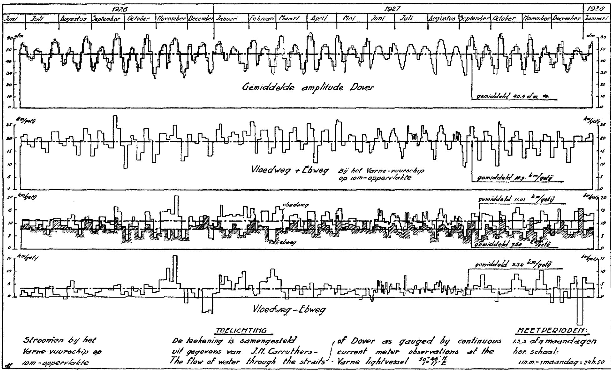
Fig. 35. Overzicht van de Stroomingen bij het Varne-lightschip.
