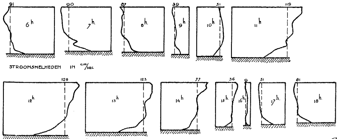
Fig. 6. Voorbeeld voor een meetgrafiek (voor punt R).
