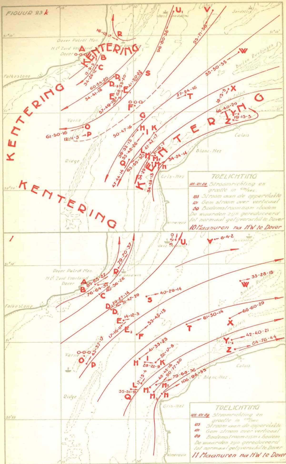
Fig. 23k en l. De twaalf-urenkaartjes van de normale stroomen in de Hoofden.
