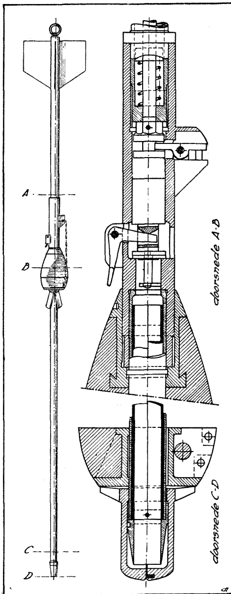
Fig. 137. Bodemstooter (naar EKMAN).
