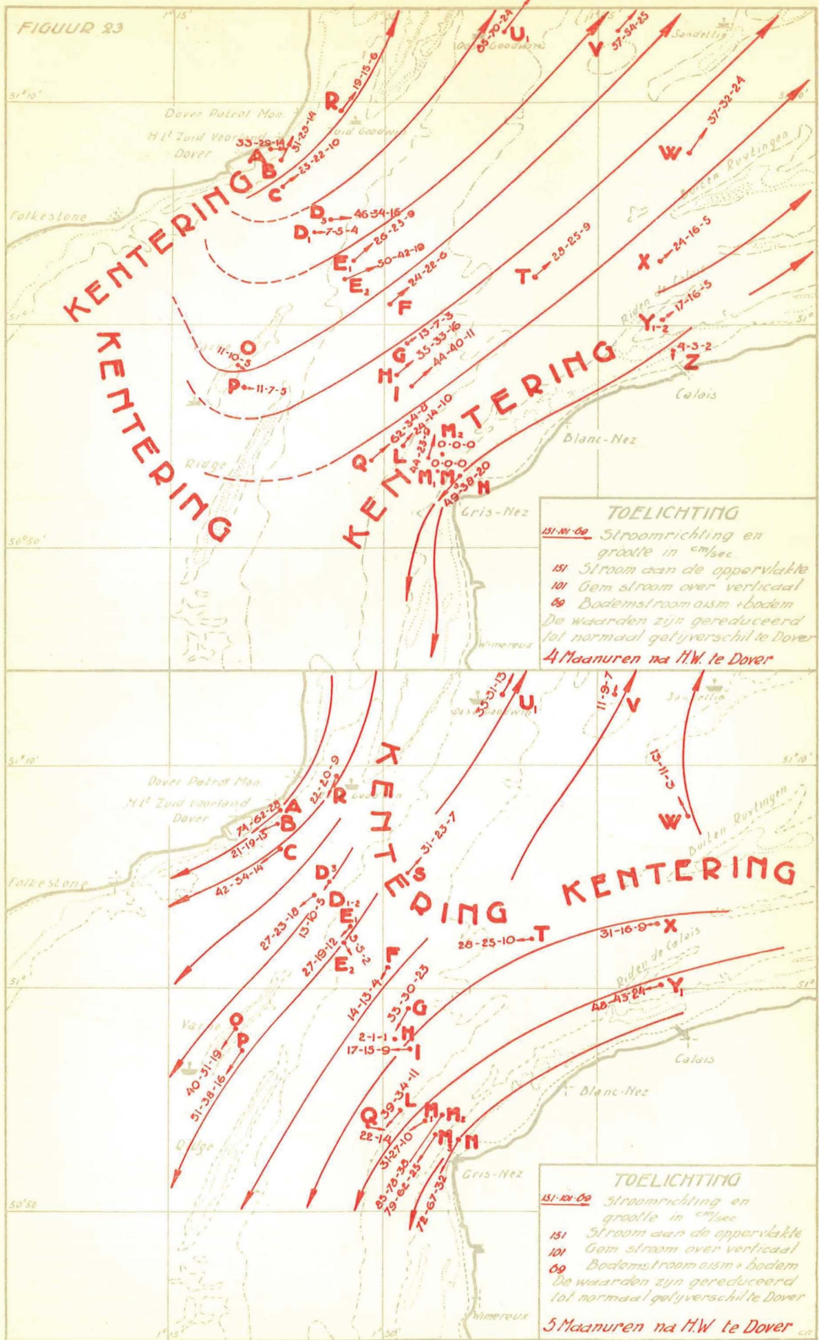
Fig. 23e en f. De twaalf-urenkaartjes van de normale stroomen in de Hoofden.
