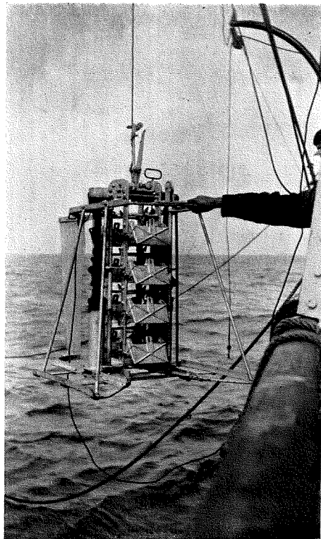
Fig. 134. Het binnenhalen van den gehaltemeter.
