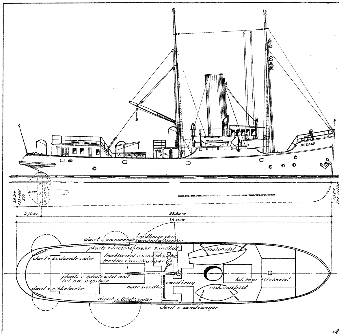
Fig. 144. Inrichting van het opnemingsvaartuig „Ocean”.
