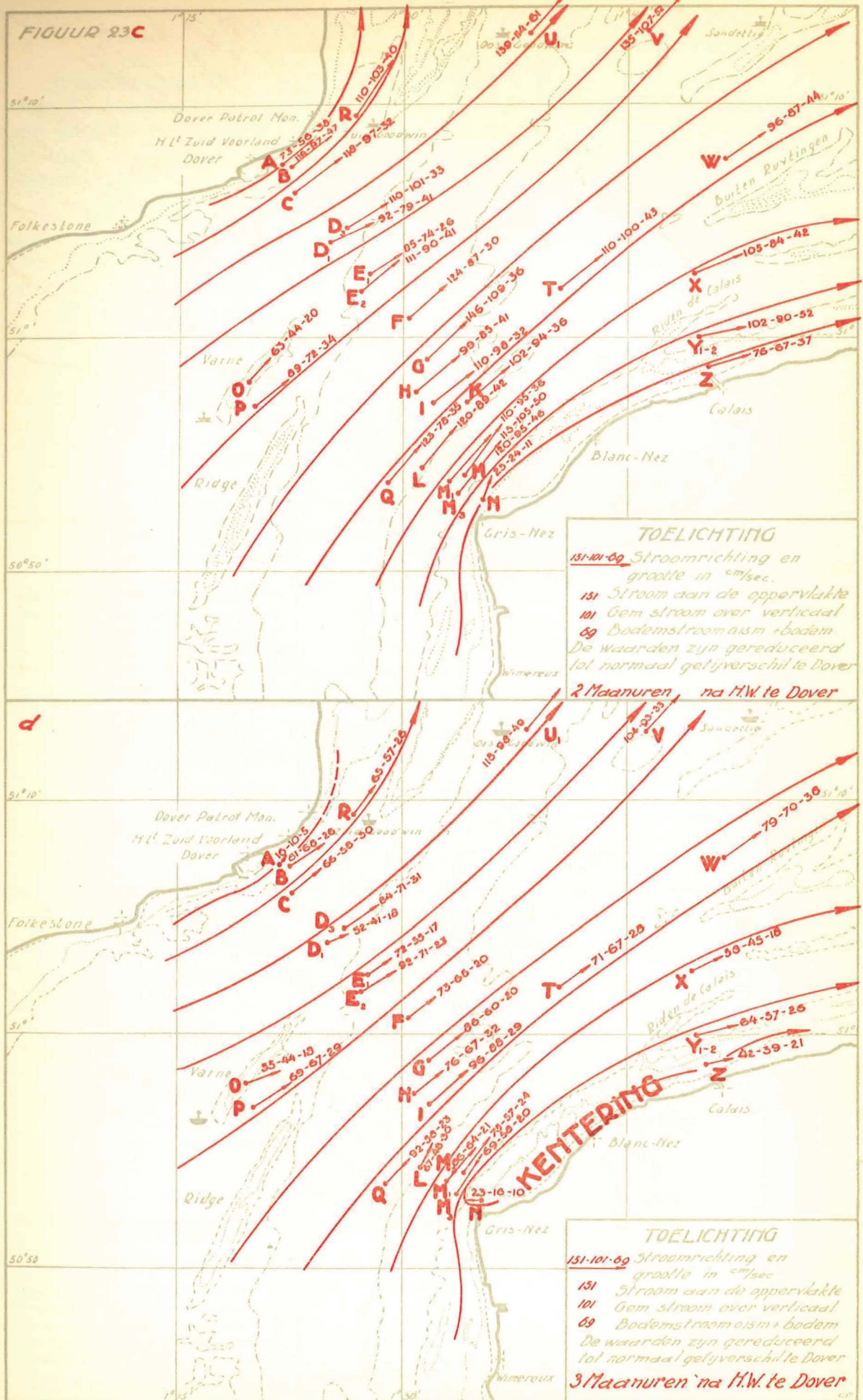
Fig. 23c en d. De twaalf-urenkaartjes van de normale stroomen in de Hoofden.
