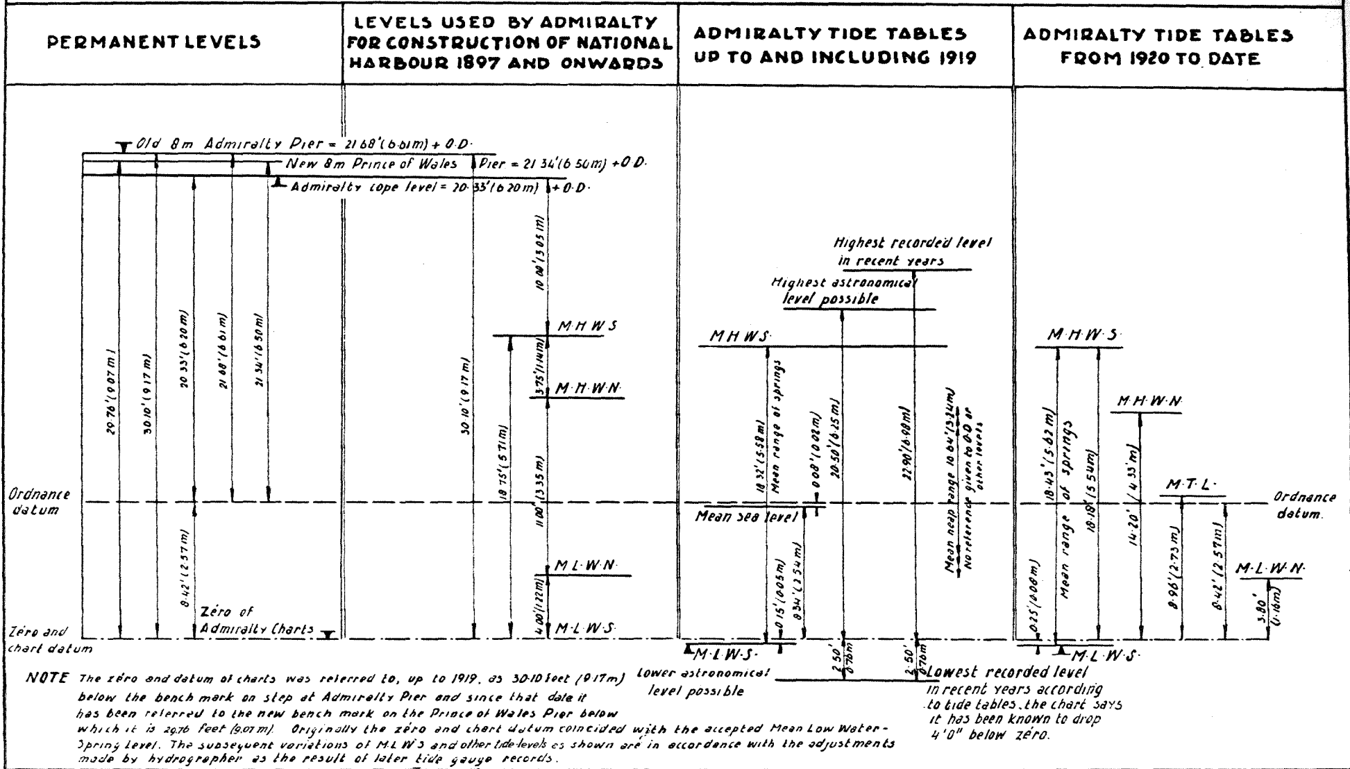
Fig. 40. Getijgegevens van Dover.
