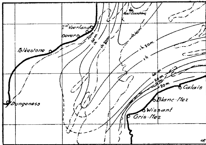
Fig. 25. Tijdlijnen der maximum ebstroomen ten opzichte van L. W. te Dover.
