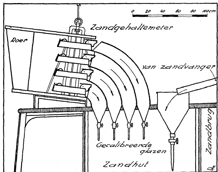
Fig. 143. Schets der zandhutinstallatie.
