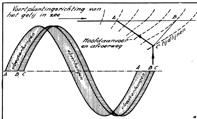
Fig. 97. Schema van de getijvoortplanting in een dubbelen mond.
