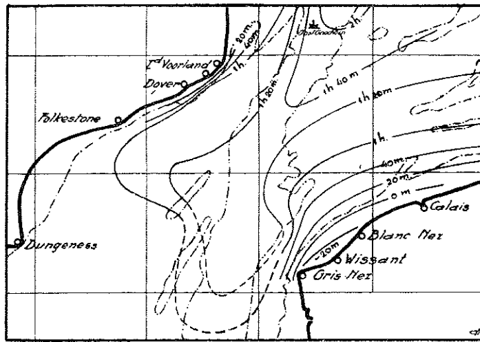
Fig. 24. Tijdlijnen der maximum vloedstroomen ten opzichte van H. W. te Dover.
