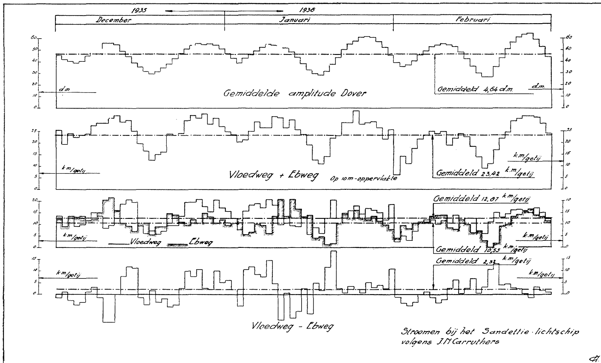
Fig. 36. Overzicht van de Stroommetingen bij het Sandettie-lichtschip.
