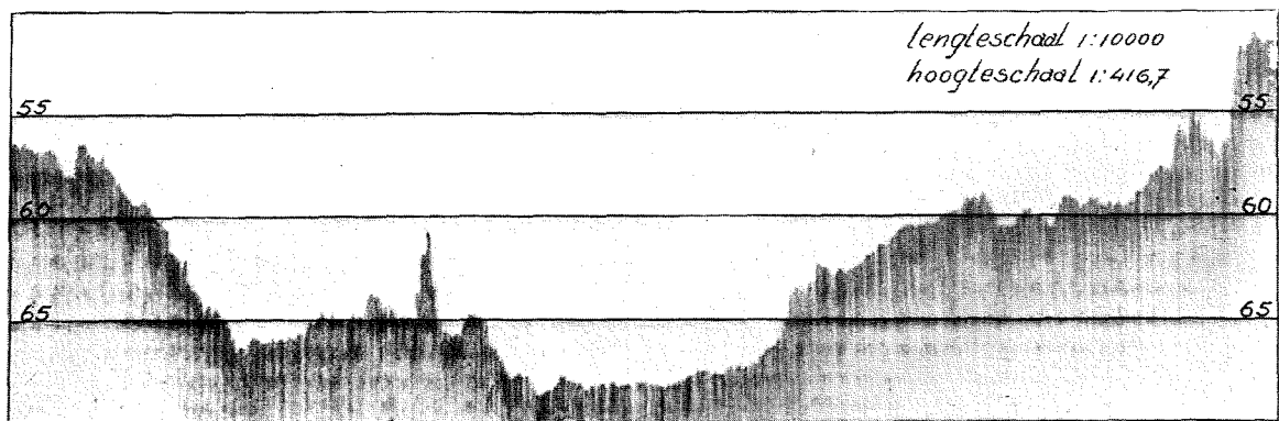
Registratie van den rotsbodem in de raai Gris Nez-Zuid Voorland.
