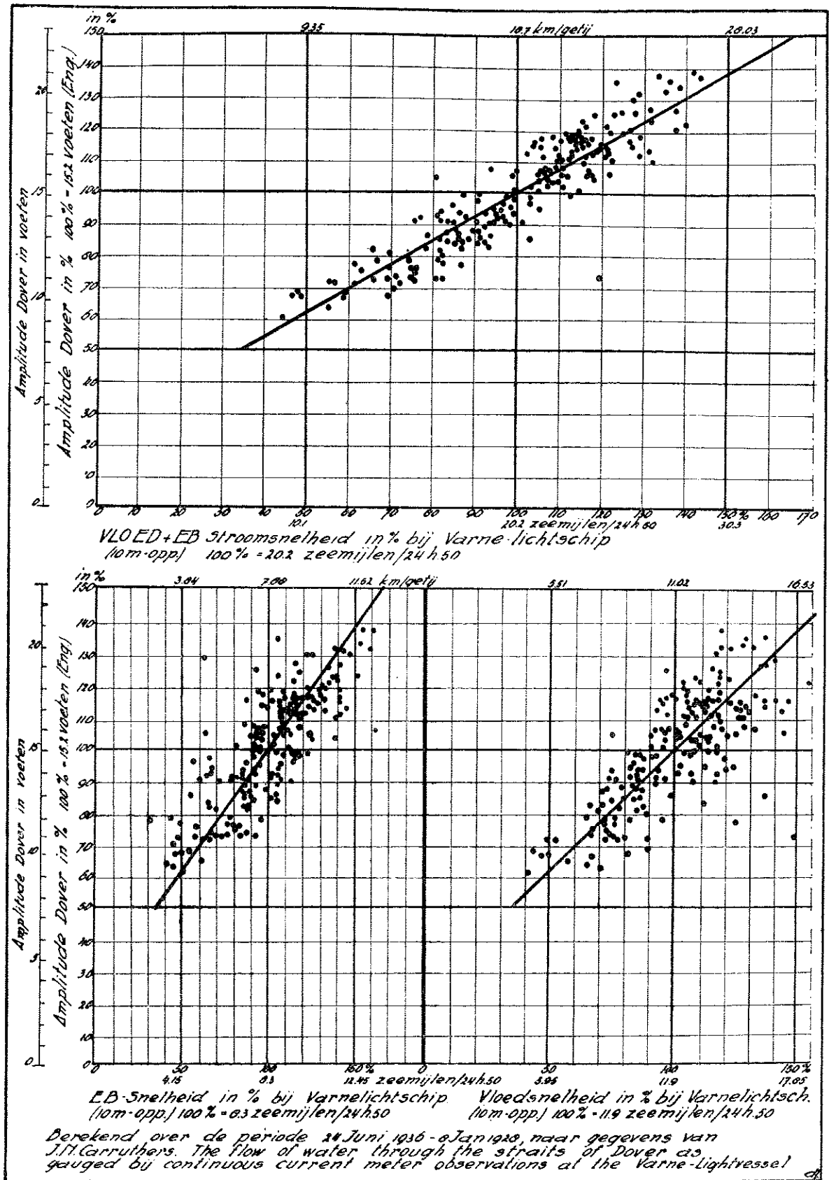
Fig. 21. Reductiegrafiek voor de stroomen bij het Varne lichtschip.
