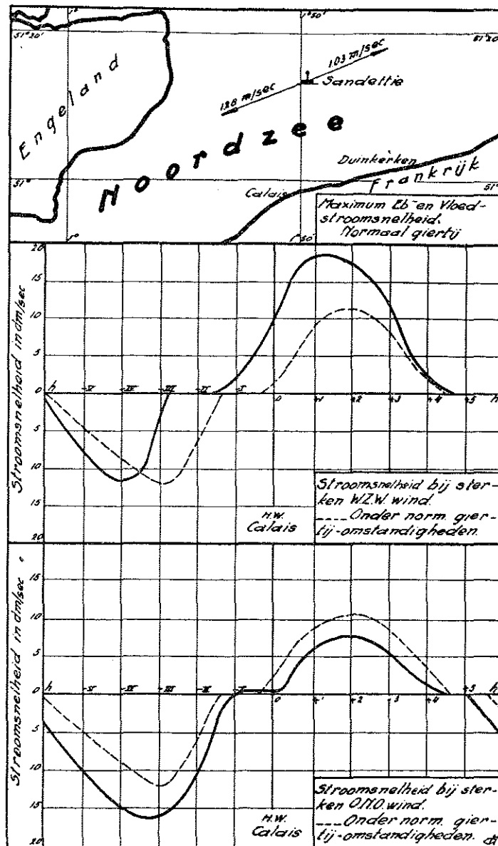
Fig. 34. Stroommetingen bij het Sandettie lichtschip volgens HELDT. (1923)
