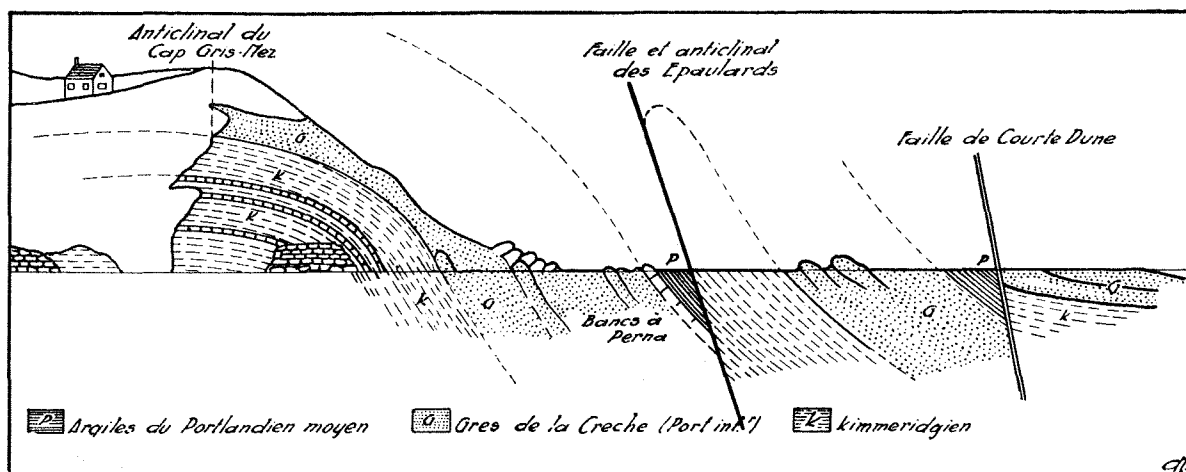
Fig. 50. Aanzicht van Kaap Gris Nez (Zwartenes) volgens PRUVOST.
