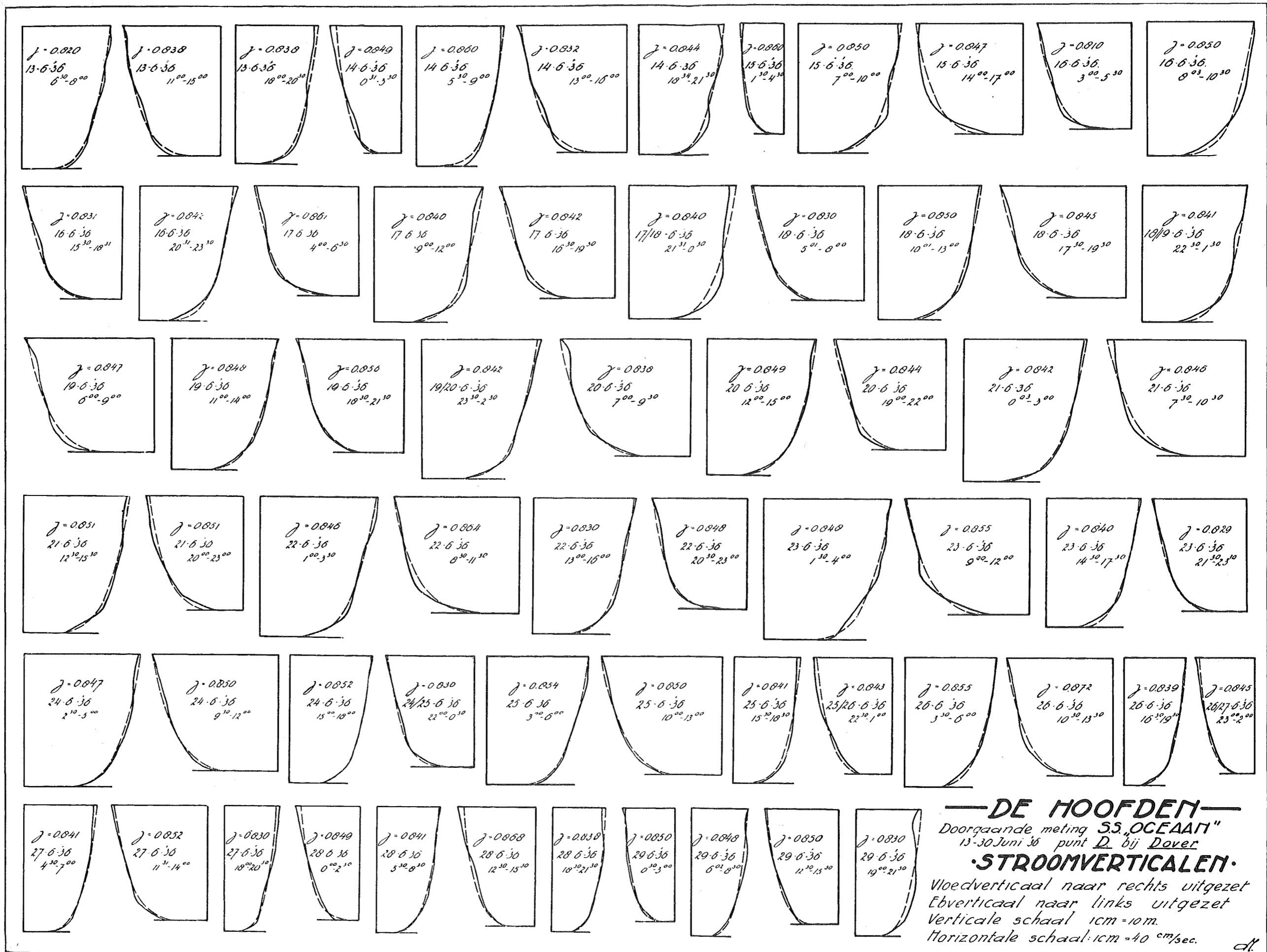
Fig. 148. Stroomverticalen in punt D.
