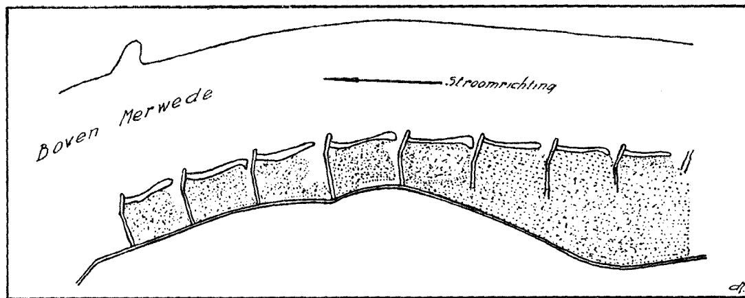
Fig. 106. Oeverlijnen tusschen de kribben van rivieren.
