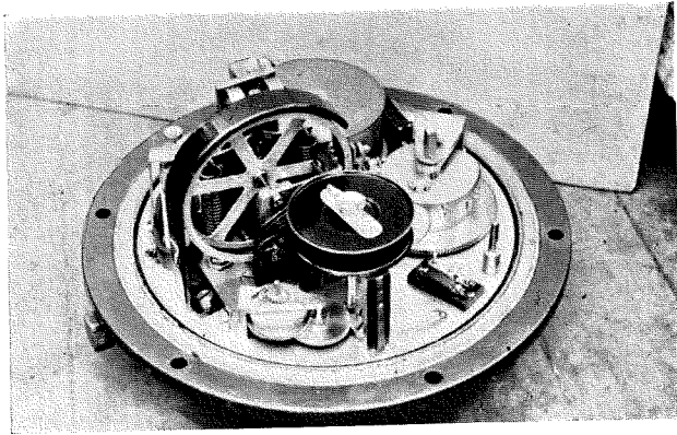
Fig. 126. Zelfteekenende peilschaal (DE VRIES).
