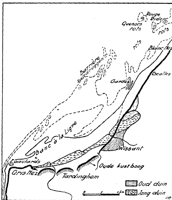
Fig. 64. Situatie kustboog bij Wissant volgens BRIQUET.
