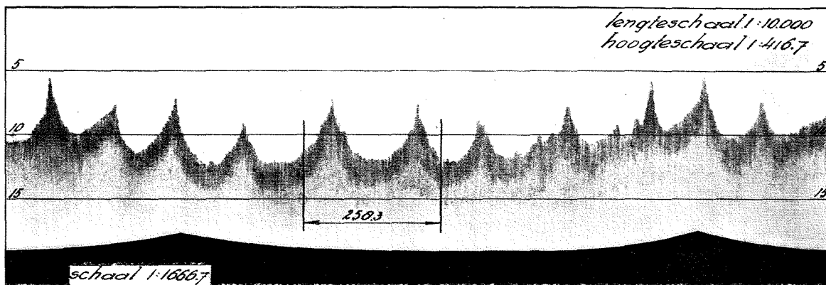
Trochoïdale zandgolven bij Goeree.
