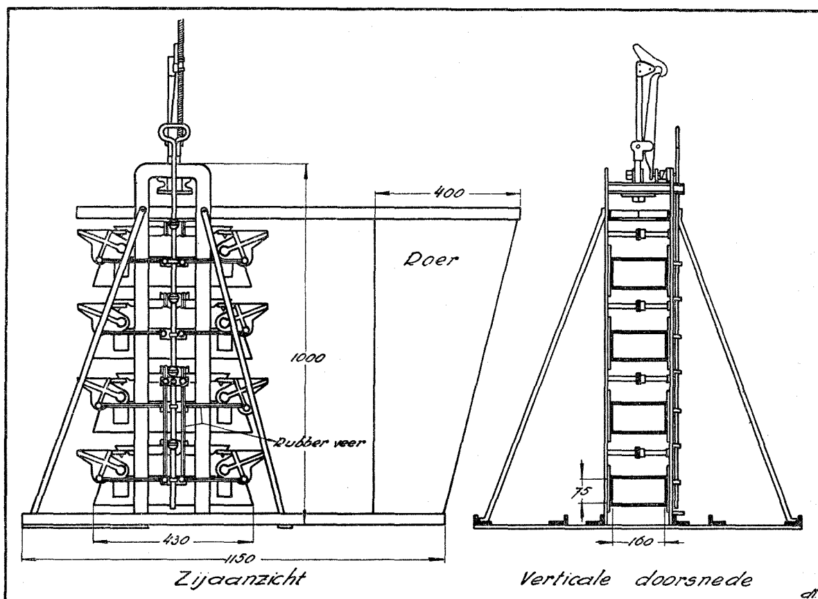
Fig. 133. Gehaltemeter (eigen ontwerp).
