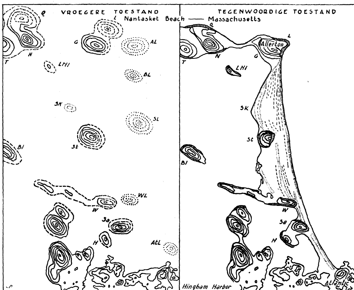
Fig. 95. Voorbeeld van een landtongformatie met vaste punten (JOHNSON).
