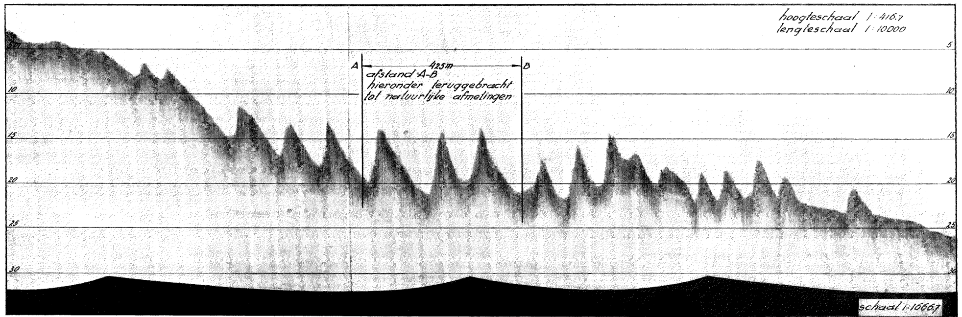
Fig. 68. Echoregistratie voor de lengte-as van het noordeinde der Varnebank.
