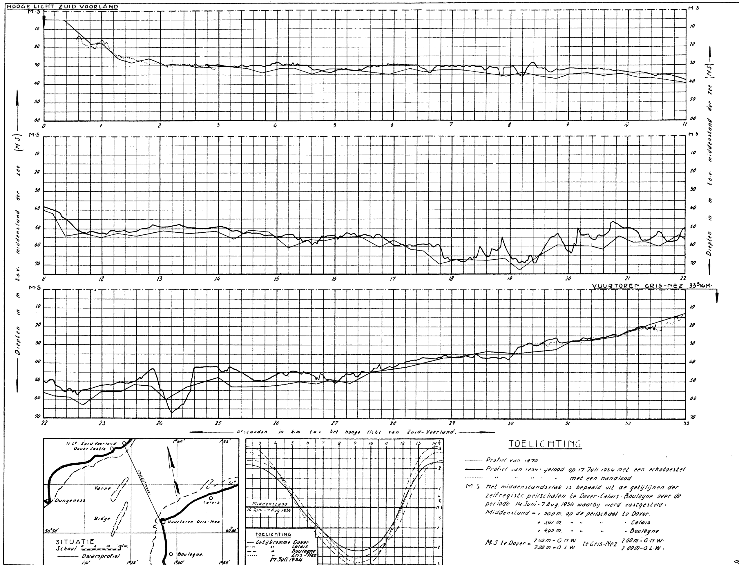
Fig. 38. Loading van het profiel Gris-Nez — Zuid Voorland. Opname 1934.
