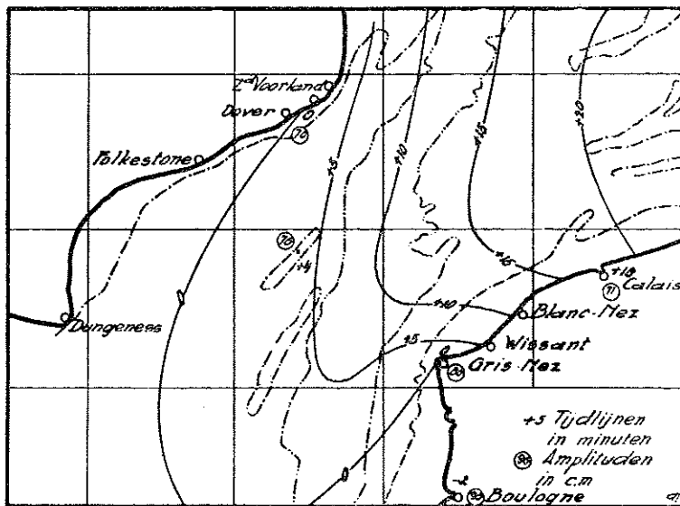
Fig. 29. Tijddijnen en amplituden van het M_2 getij in de periode van waarneming.
