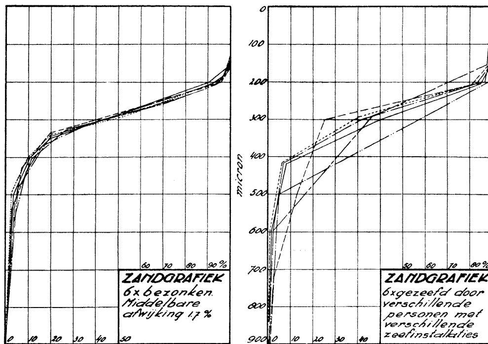
Fig. 139. Vergelijking der uitkomsten van bezinkingsmeter en zeefinstallaties.
