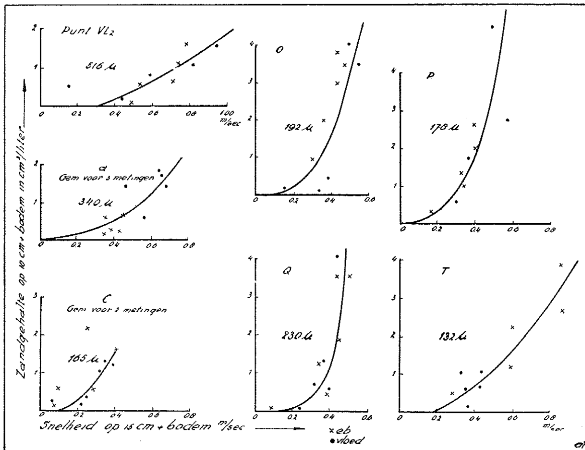
Fig. 20. Verband tusschen de snelheid op 0,15 m boven den bodem en het zandgehalte op 0,10 m boven den bodem voor verschillende plaatsen in het zeevat van het Vlie.
