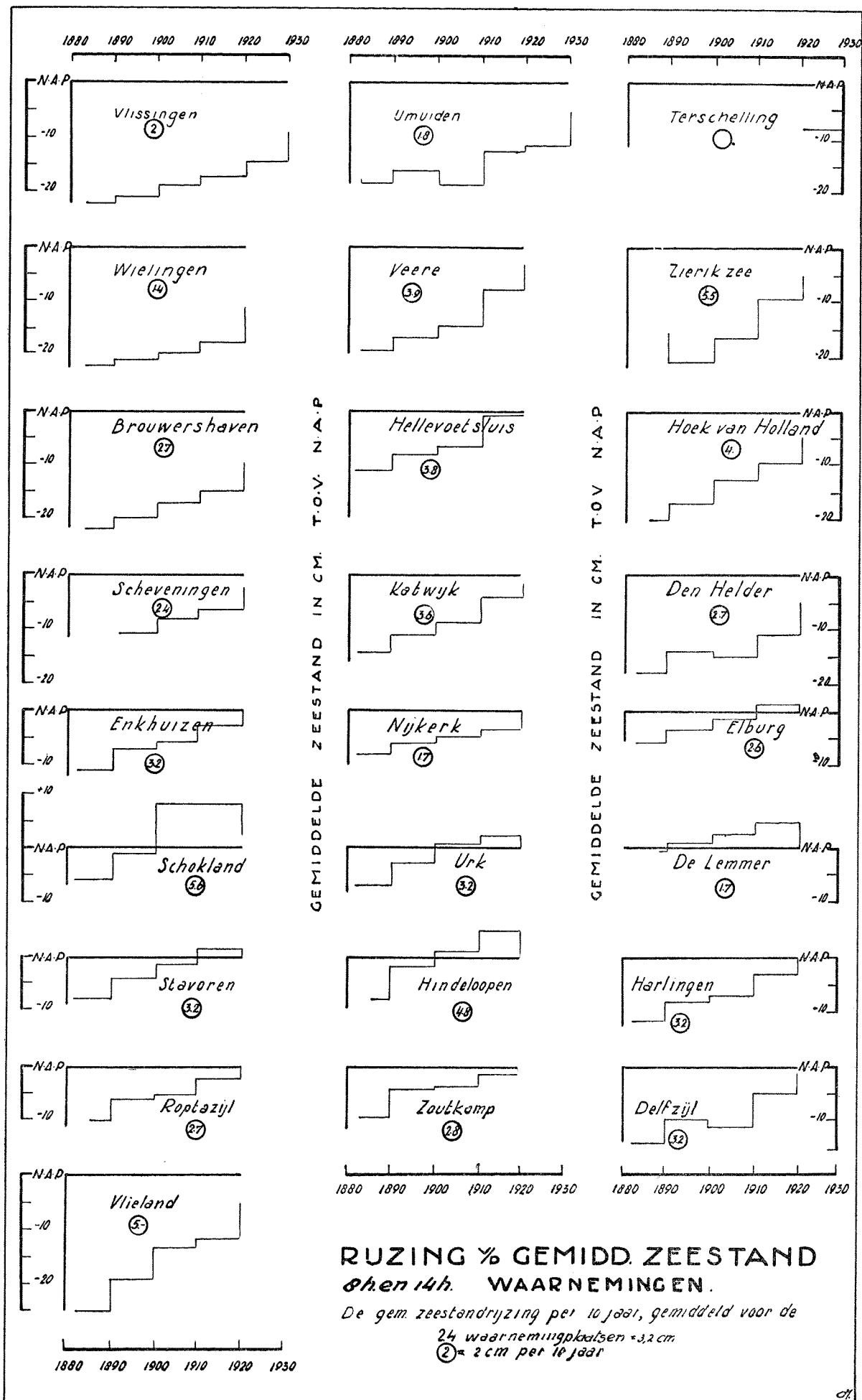
Fig. 118. Rijzing van den gemiddelden zeebestand.
