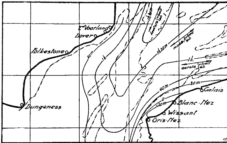
Fig. 28. Algemeen phaseverschil tusschen het horizontale getij en het verticale getij te Dover. Het horizontale getij ijlt na.
