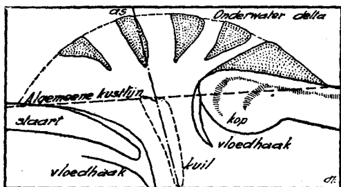
Fig. 96. Algemeene vorm van een zeegat in strandwalkusten.
