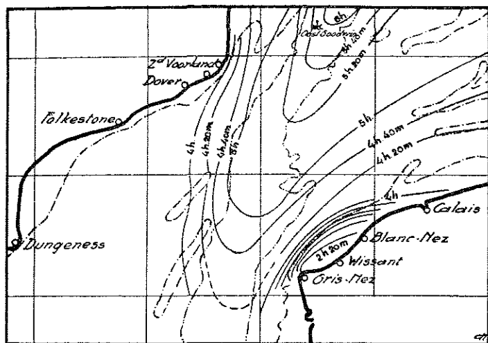
Fig. 26. Tijdlijnen der kenteringen van vloed op eb ten opzichte van H. W. te Dover.
