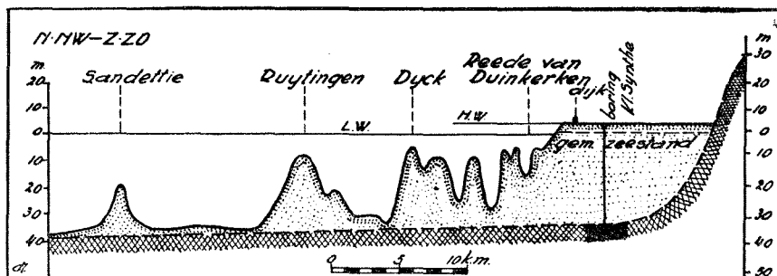
Fig. 81. Profiel loodrecht op de Vlaamsche kust (BRIQUET).
