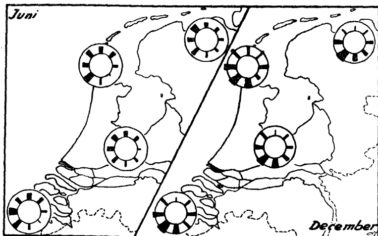
Fig. 101. Windrozen voor Nederland voor Juni en December.
