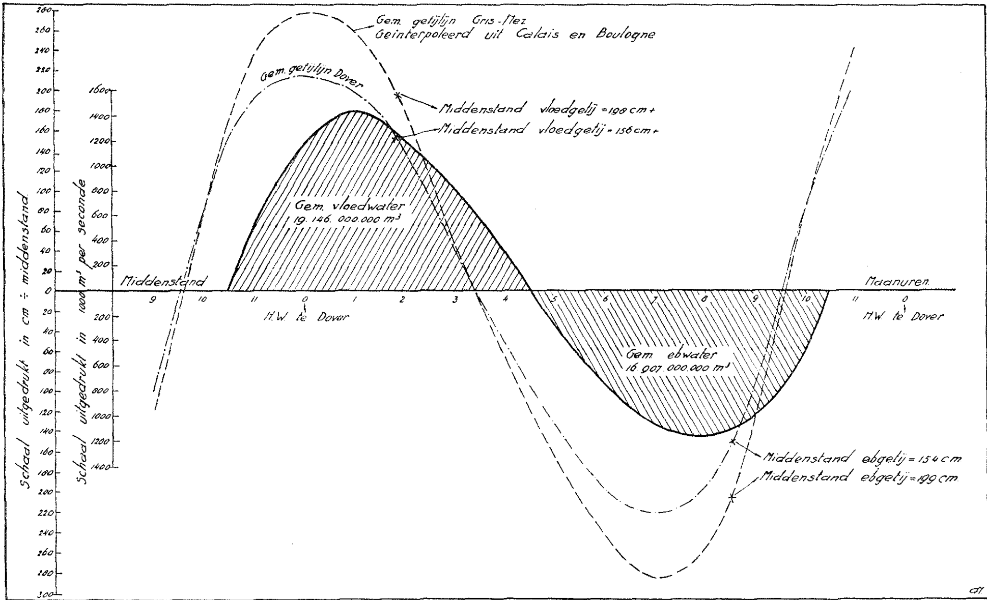
Fig. 32. De afvoerkromme van de Hoofden.
