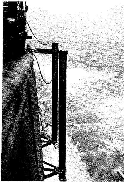
Fig. 125. Bevestiging der oscillatoren van het echotoestel.
