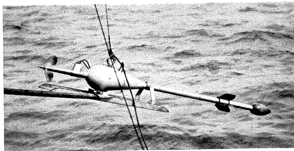
Fig. 128. OTT-stroommeter van 100 kg.
