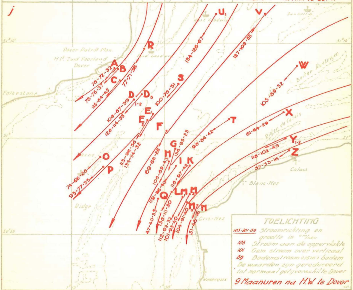
Fig. 23i en j. De twaalf-urenkaartjes van de normale stroomen in de Hoofden.
