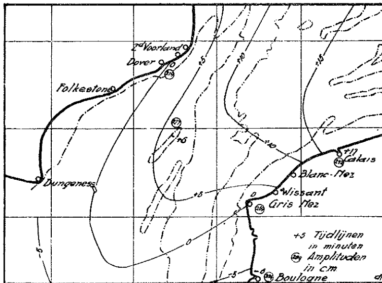
Fig. 30. Tijddijnen en amplituden van het S_2 getij in de periode van waarneming.
