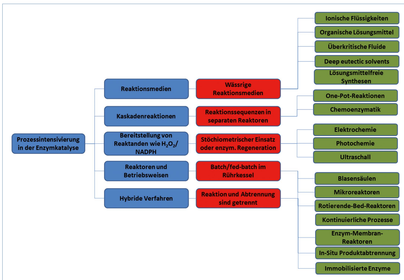
▲ Abb. 1: Die Prozessintensivierung (PI) in der Enzymkatalyse. blau: in der PI adressiertes Verfahren, rot: Ausgangspunkt eines hypothetischen „Standardprozesses“, grün: Werkzeuge und Methoden im PI.
