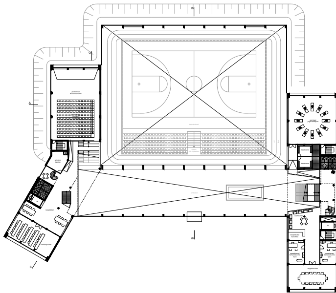
eerste verdieping (1:200)
