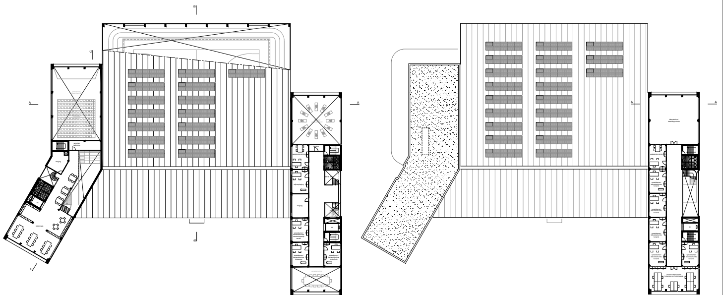
tweede verdieping (1:200)
