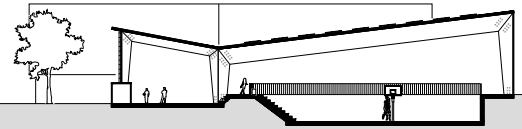
doorsnede B-B (1:200)
