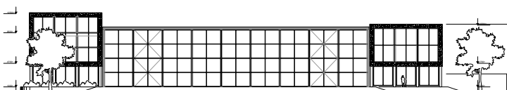
noordgevel (1:200)
