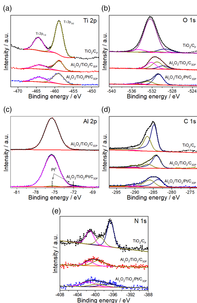
Figure 4. XPS spectra of a) Ti 2 p , b) O 1 s , c) Al 2 p , d) C 1 s , and e) N 1 s of the pyrolyzed samples TiO 2 /C P , Al 2 O 3 /TiO 2 /C 3DP , and Al 2 O 3 /TiO 2 /Pt/C 3DP .
