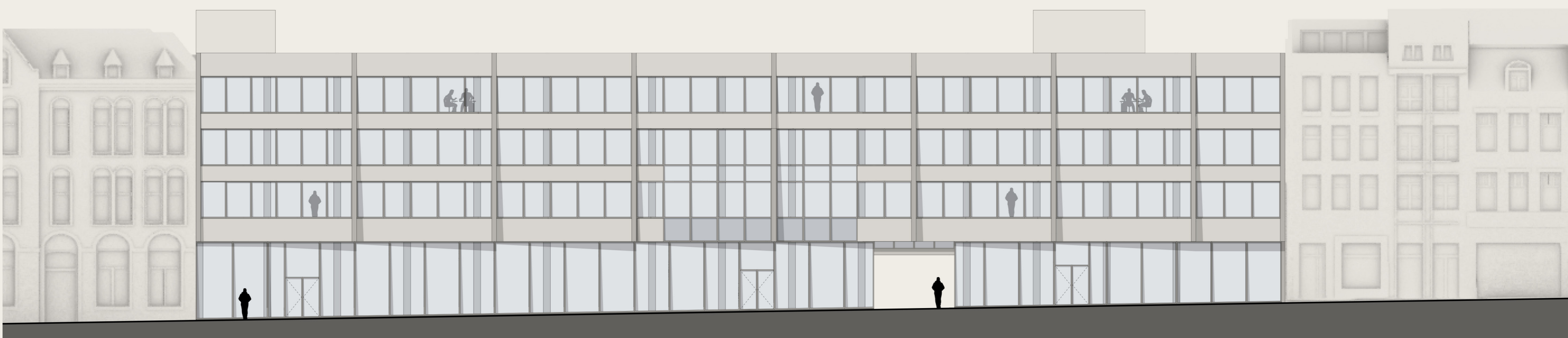
MOLENSTRAAT ELEVATION
