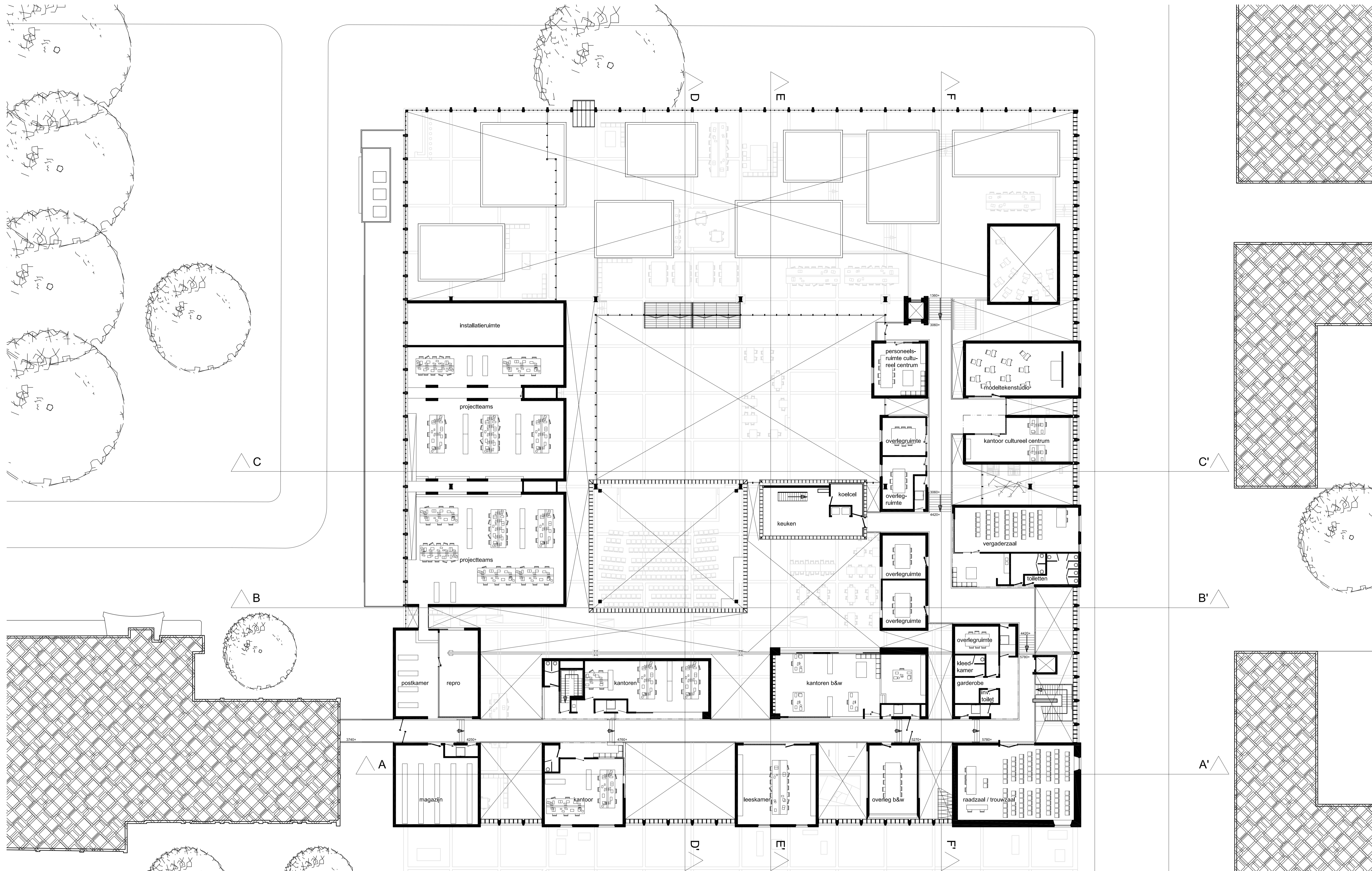
Verdieping - 1:200
