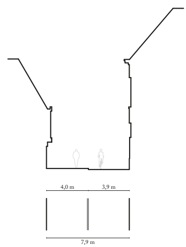
Section A Zakstraat
