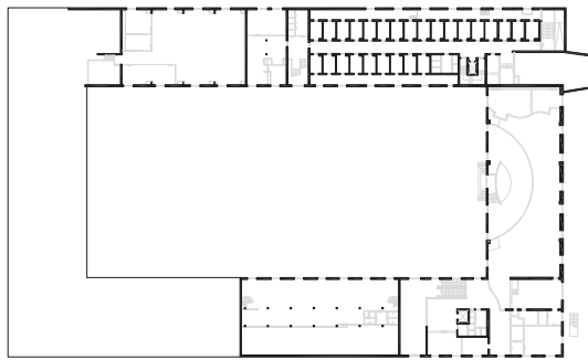
Entresol
